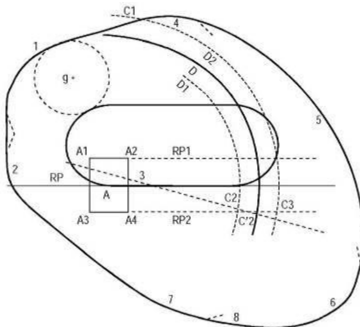
Рисунок III-3-7-Доб А-5 - Основная зона ожидания RNAV для системы RNAV без функции ожидания. Участок удаления определяется по расстоянию
