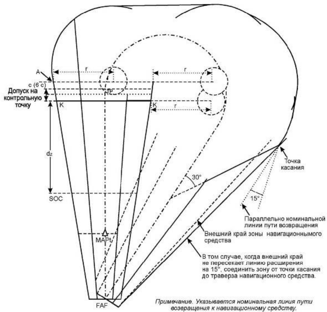
Рисунок I-4-6-17 - Уход на второй круг с разворотом при наличии контрольной точки ТР и возвращением к навигационному средству по линии пути возвращения
