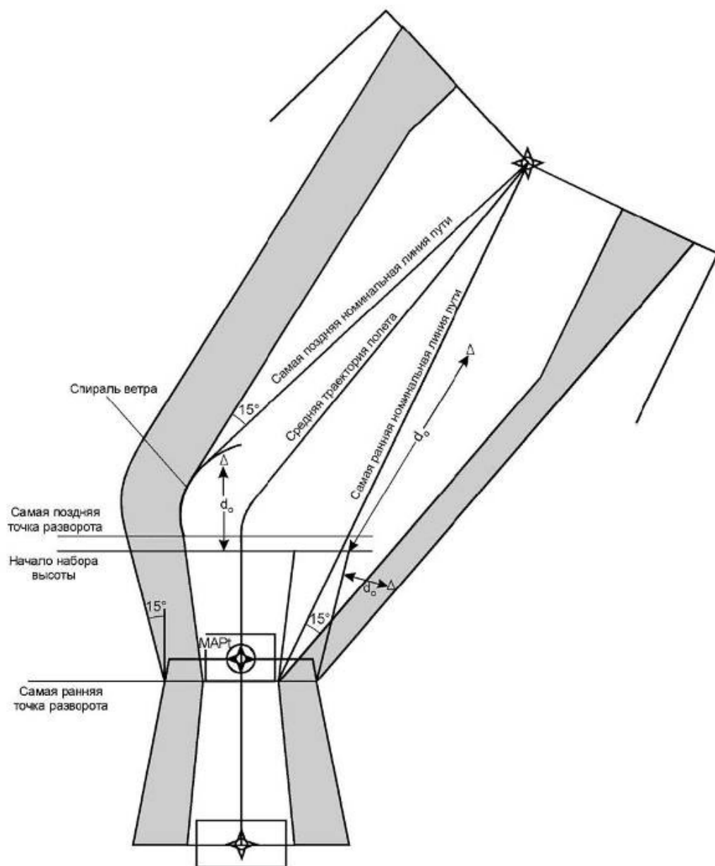
Рисунок III-2-2-11 - Разворот при уходе на второй круг в MAPt, после которого следует участок DF
