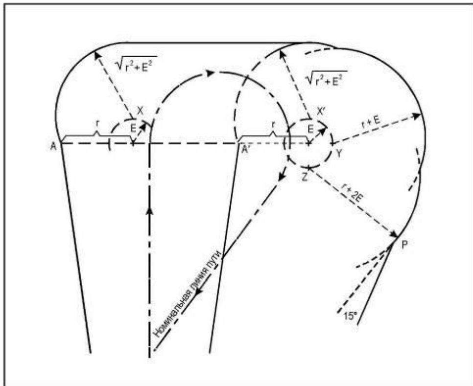
Рисунок 1-2-3-5 - Построение внешней границы разворота
