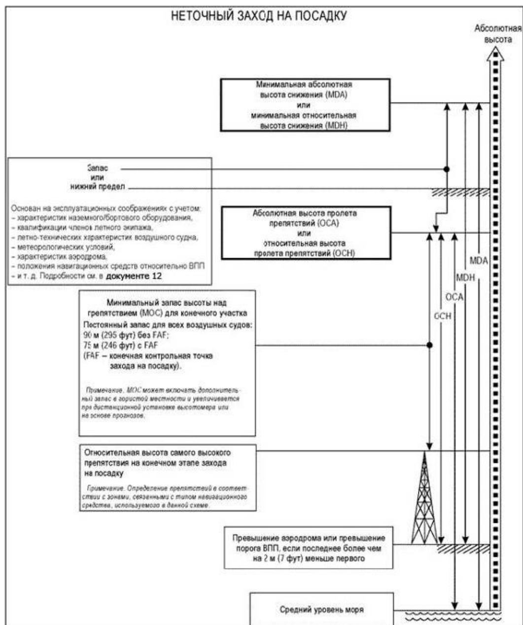
Рисунок I-4-5-3 b) - Взаимосвязь абсолютной/относительной высоты пролета препятствий (OCA/H) с минимальной абсолютной/относительной высотой снижения (MDA/H) при неточных заходах на посадку
