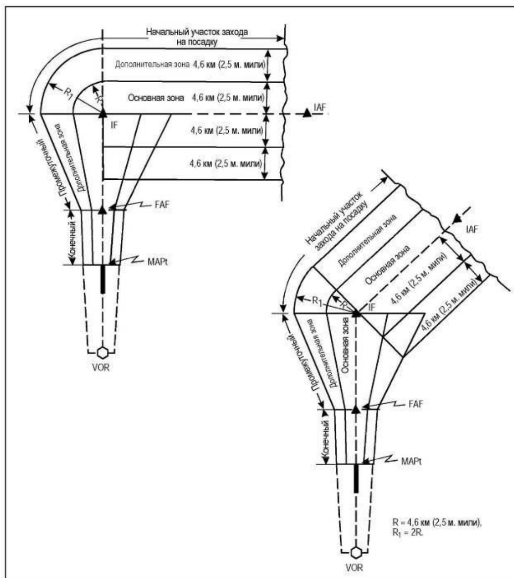
Рисунок II-2-4-3 - Типичный участок захода на посадку (развороты на 45 и 90°)
