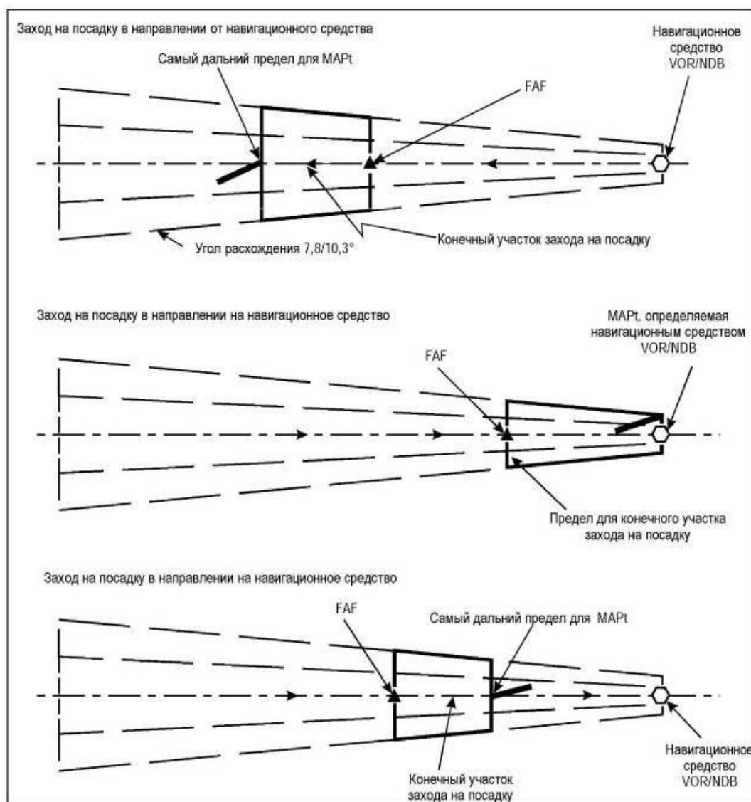
Рисунок II-2-4-4 - Конечный участок захода на посадку (VOR/NDB)
