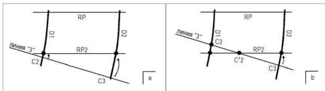
Рисунок III-7-3-Доб А-6 - Зона, включающая конец участка удаления (п. А.3.7.3.2.2.3 г) Добавления А к главе 3.7 части III)
