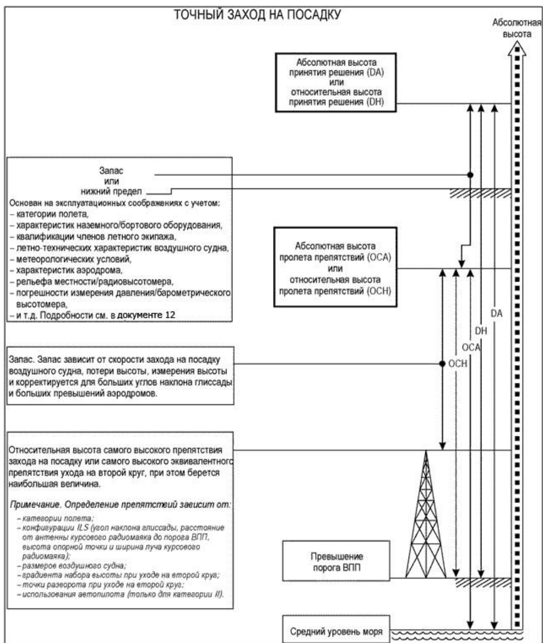
Рисунок I-4-5-3 а) - Взаимосвязь абсолютной/относительной высоты пролета препятствий (OCA/H) с абсолютной/относительной высотой принятия решения (DA/H) при точных заходах на посадку
