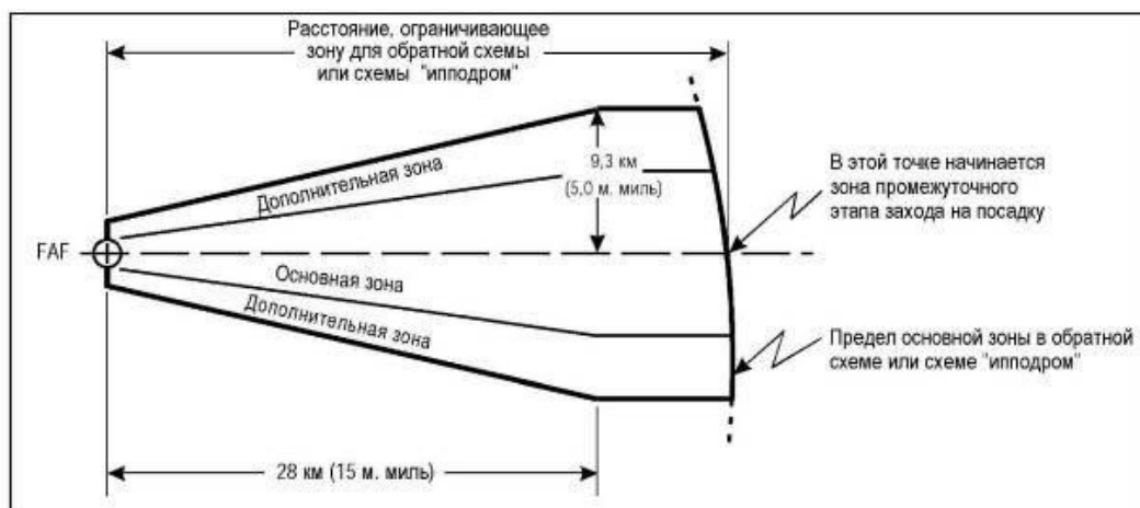
Рисунок I-4-4-2 - Зона промежуточного этапа захода на посадку в пределах обратной схемы или схемы "ипподром" при отсутствии IF
