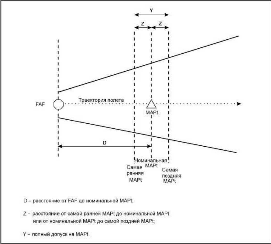
Рисунок I-4-6-3 - Расстояние от номинальной MAPt до самой ранней и самой поздней MAPt
