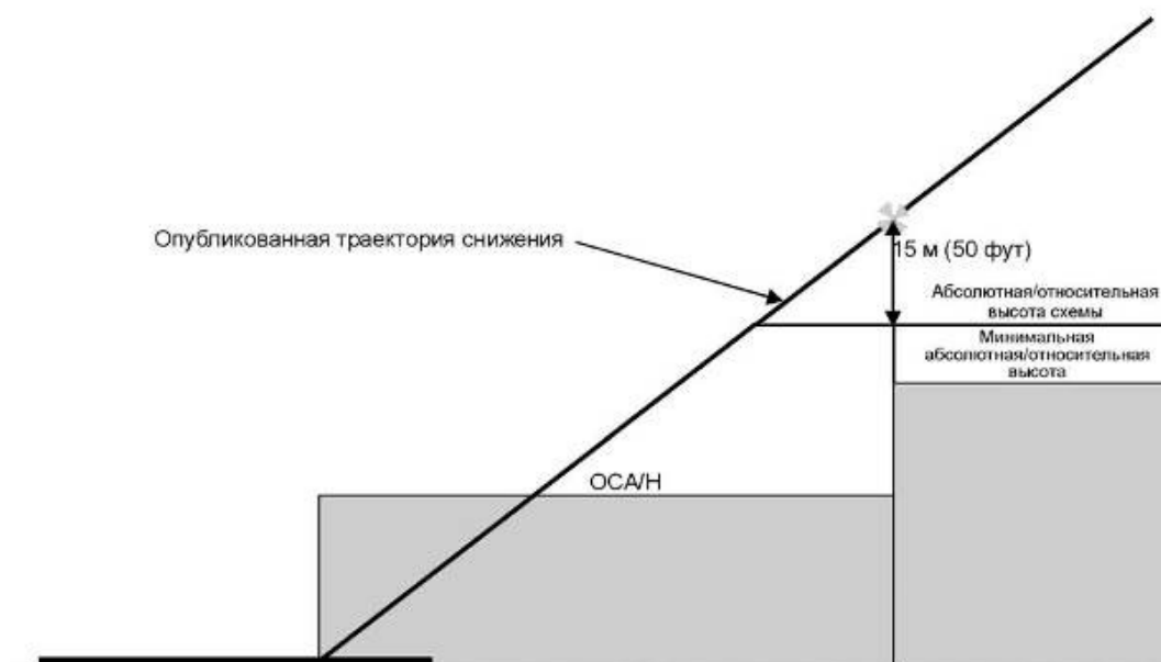
Рисунок I-4-5-6 - Абсолютная/относительная высота схемы и минимальная абсолютная/относительная высота
