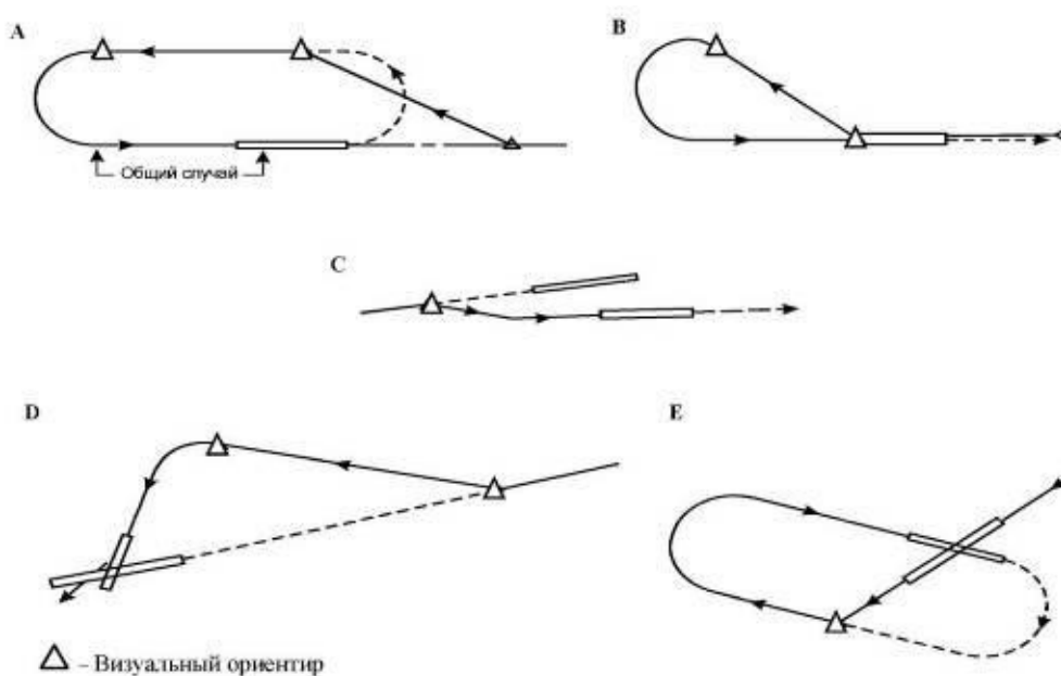
Рисунок I-4-7-Доб-1 - Характерные случаи линий пути
