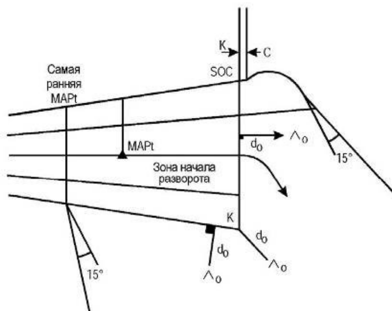
Рисунок I-4-6-20 - Разворот более чем на 15° в MAPt при уходе на второй круг
