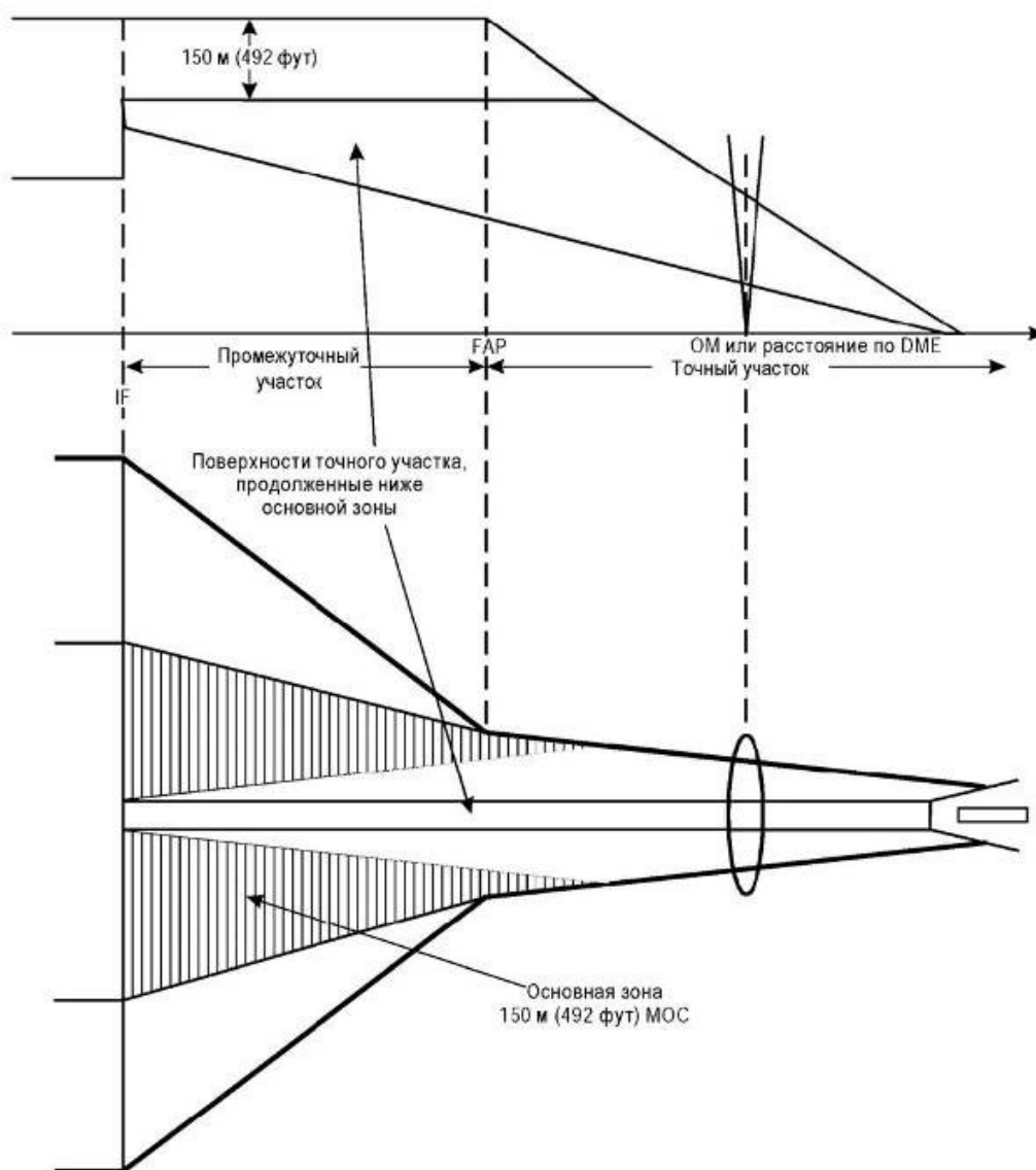
Рисунок II-1-1-3 - Точный участок при отсутствии конечной контрольной точки захода на посадку
