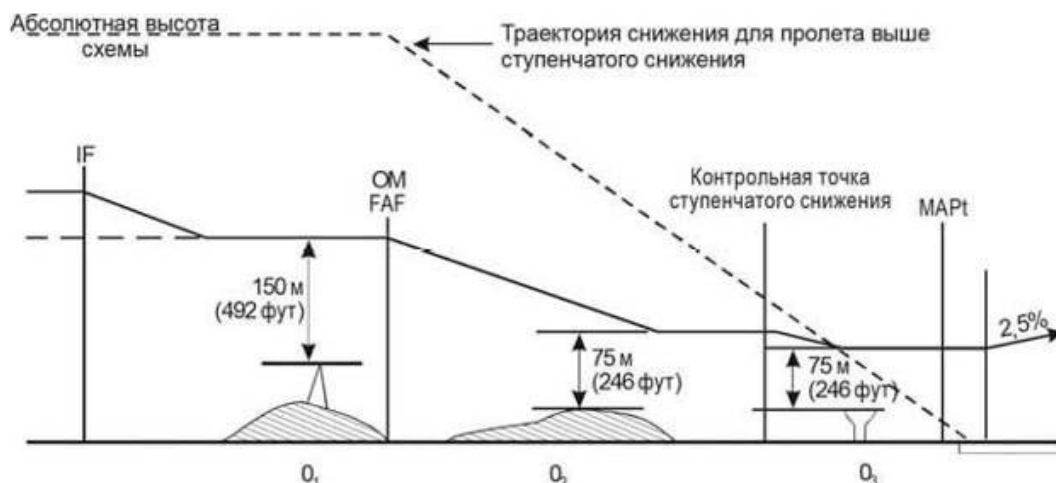
Рисунок II-2-1-2 - Схема только для курсового радиомаяка. Запас высоты над препятствиями и абсолютная высота схемы
