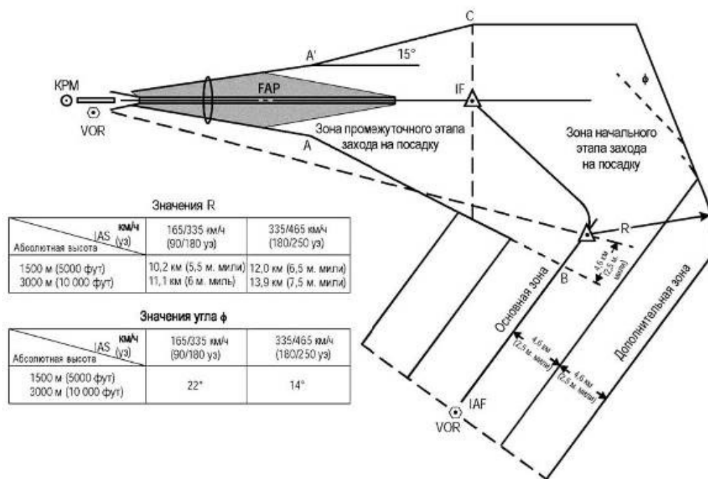
Рисунок I-4-3-Доб А-3 - Построение зон защиты в схеме типа U VOR/VOR
