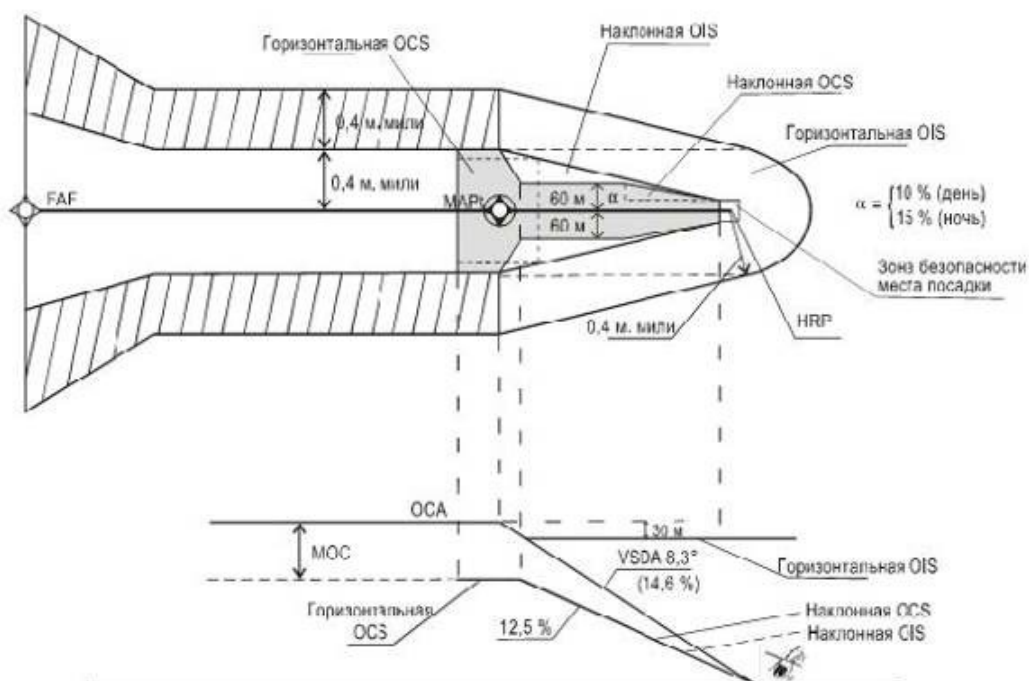
Рисунок IV-2-5 - Прямой VS без DP и без изменения курса
