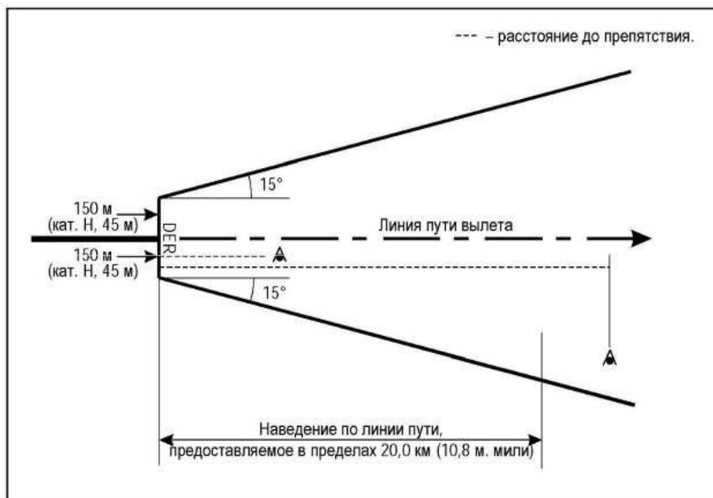
Рис. I-3-3-1 - Зона вылета по прямой без корректировки линии пути
