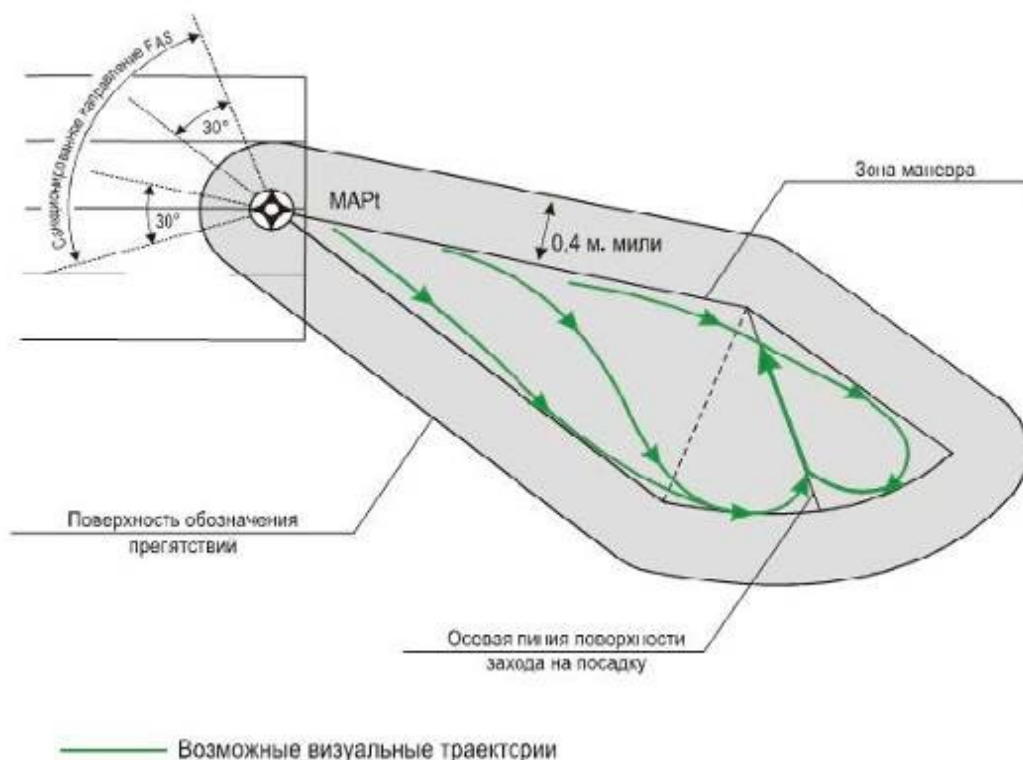
Рисунок IV-2-13 - Представление горизонтальной OIS для установленной поверхности захода на посадку
