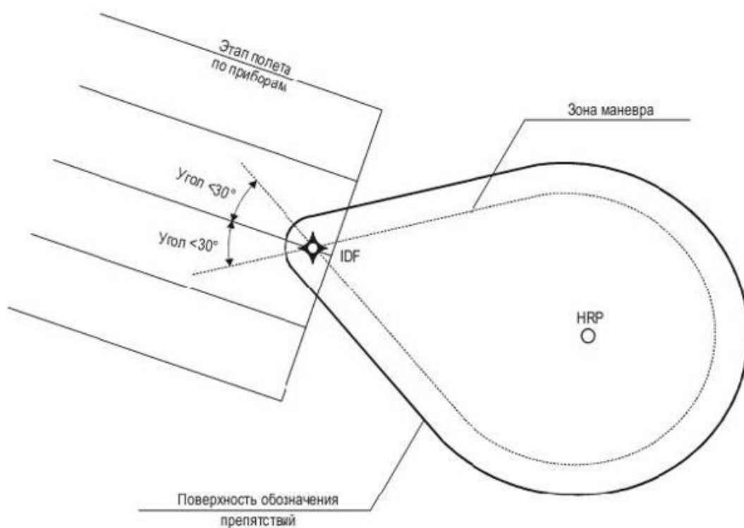
Рисунок IV-1-7 - Представление горизонтальной OIS в случае визуального участка маневрирования при заданной осевой линии поверхности набора высоты при взлете
