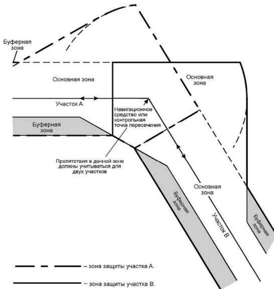
Рисунок II-3-1-6 - Объединение зон разворота для обоих направлений полета
