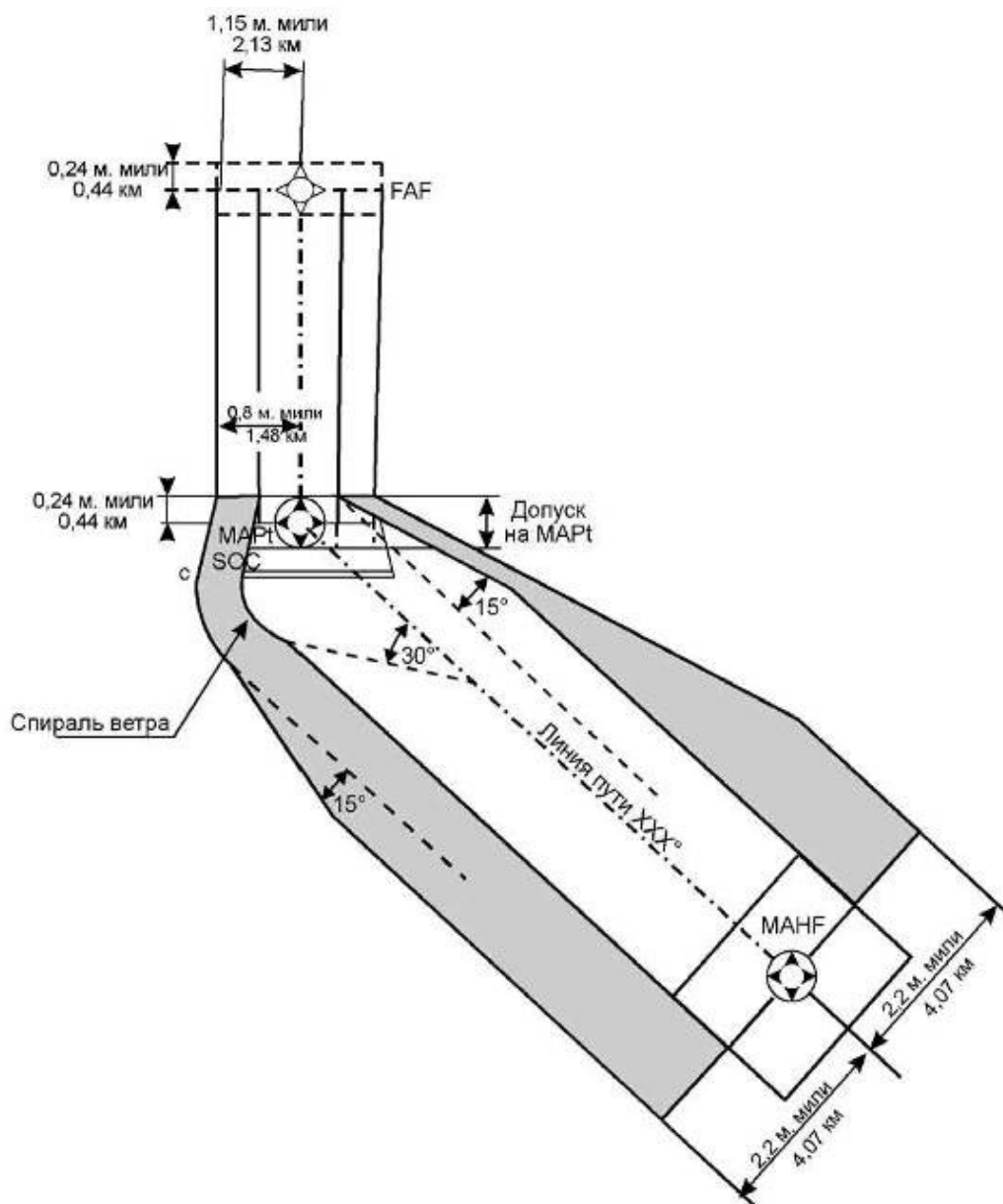
Рисунок IV-2-4 - Уход на второй круг с разворотом на угол, меньший или равный 90°
