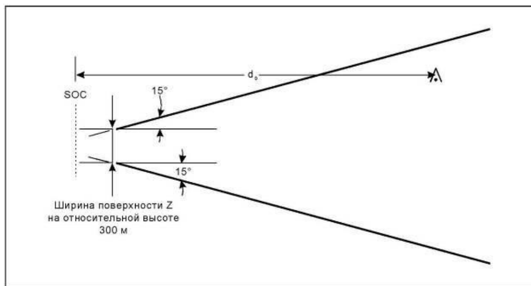
Рисунок II-1-1-15 - Конечный участок II ухода на второй круг по прямой
