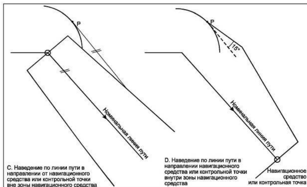
Рисунок 1-2-3-3 с) и d) - Наведение по линии пути в направлении от навигационного средства или контрольной точки вне зоны навигационного средства.
