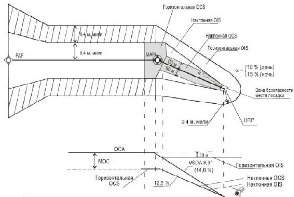
Рисунок IV-2-6 - Прямой VS без DP и с изменением курса на 30° в MAPt
