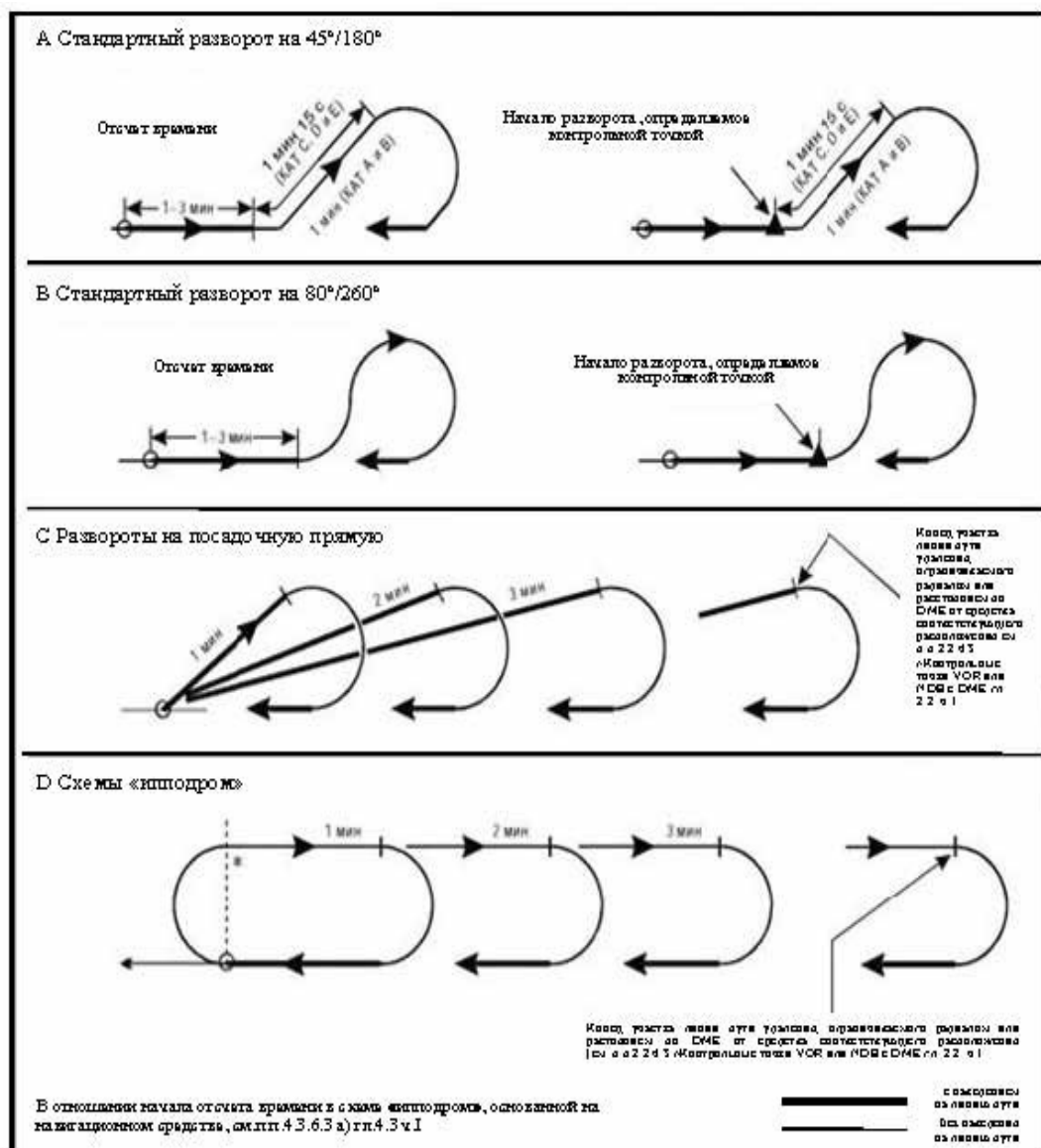
Рисунок I-4-3-7 - Типы обратных схем и схем "ипподром"
