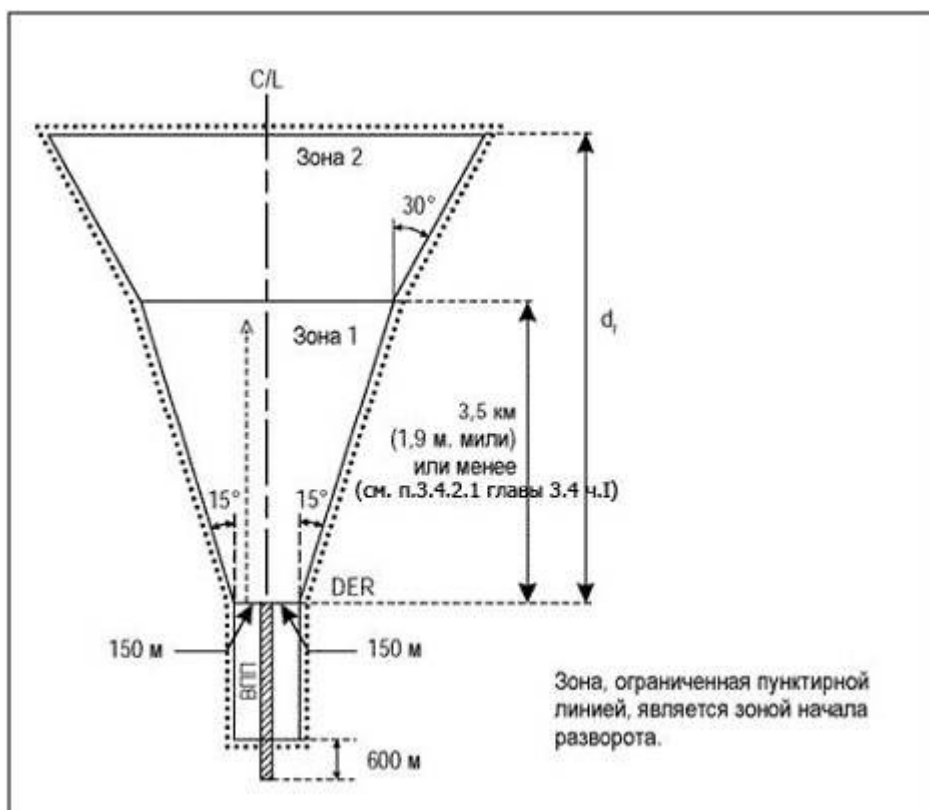
Рисунок I-3-4-1 - Зоны 1, 2 и зона начала разворота для вылета в любом направлении
