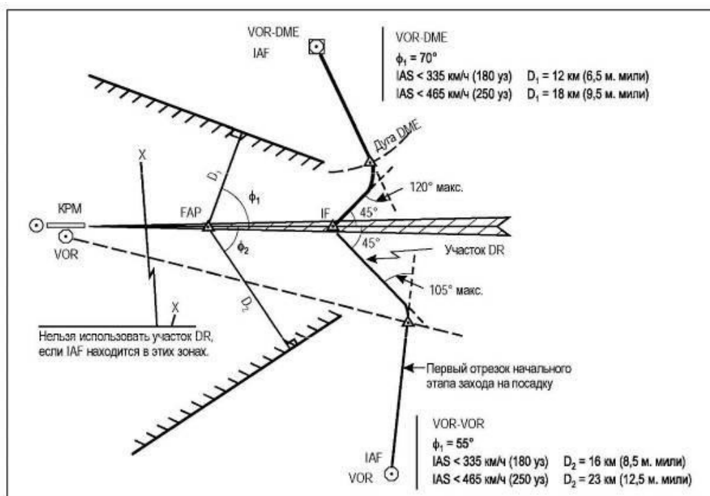
Рисунок I-4-3-Доб А-1 - Условия расположения IAF в схеме типа U
