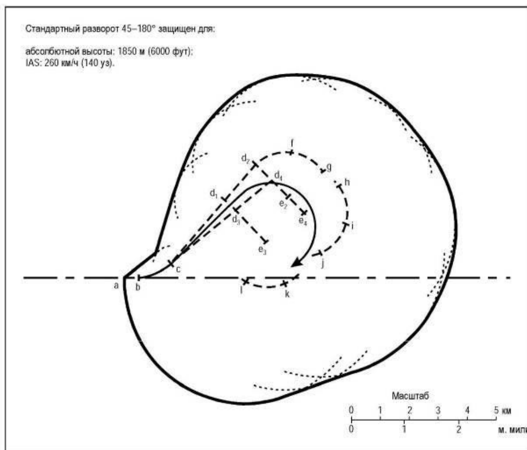
Диаграмма I-4-3-Доб С-3. Шаблон стандартного разворота 45°-180°
