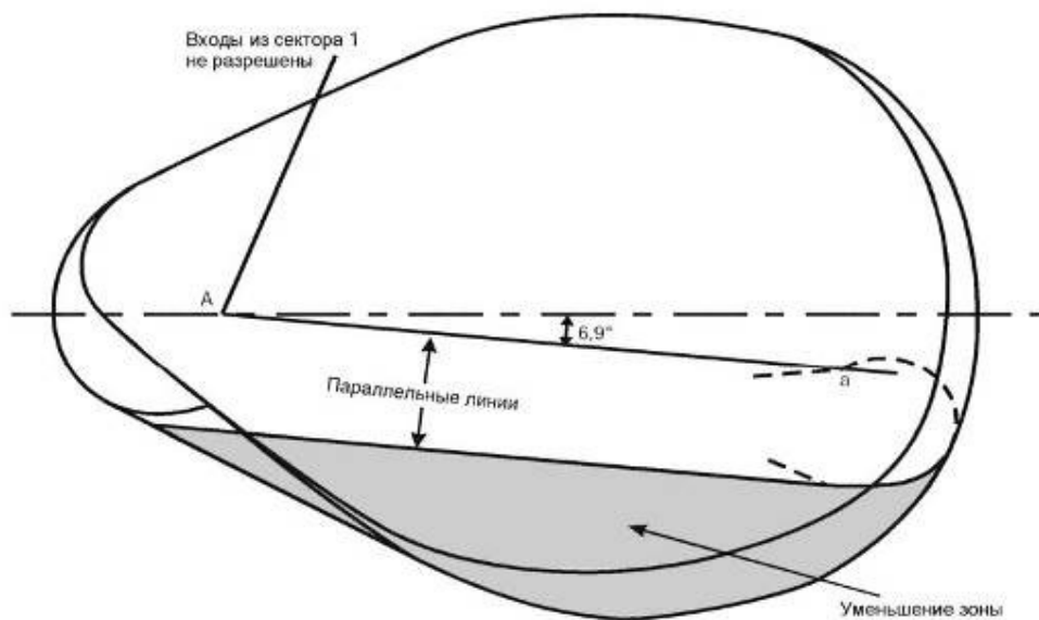
Диаграмма I-4-3-Доб С-13 - Уменьшение зоны для схемы над NDB, когда входы из сектора 1 не разрешены
