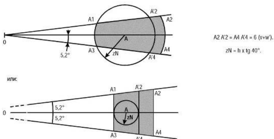
Рисунок I-4-3-Доб С-4 - VOR в 0 и NDB или привод в A
