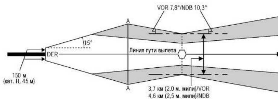
Рисунок I-3-3-4 - Вылет по прямой. Навигационное средство впереди
