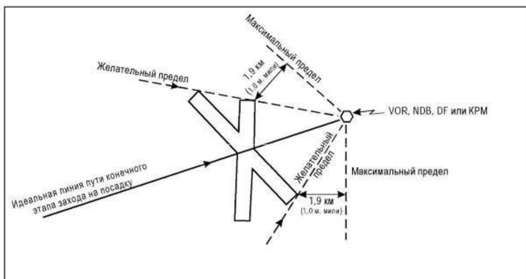
Рисунок I-4-5-2 - Выравнивание направления конечного этапа захода на посадку по кругу
