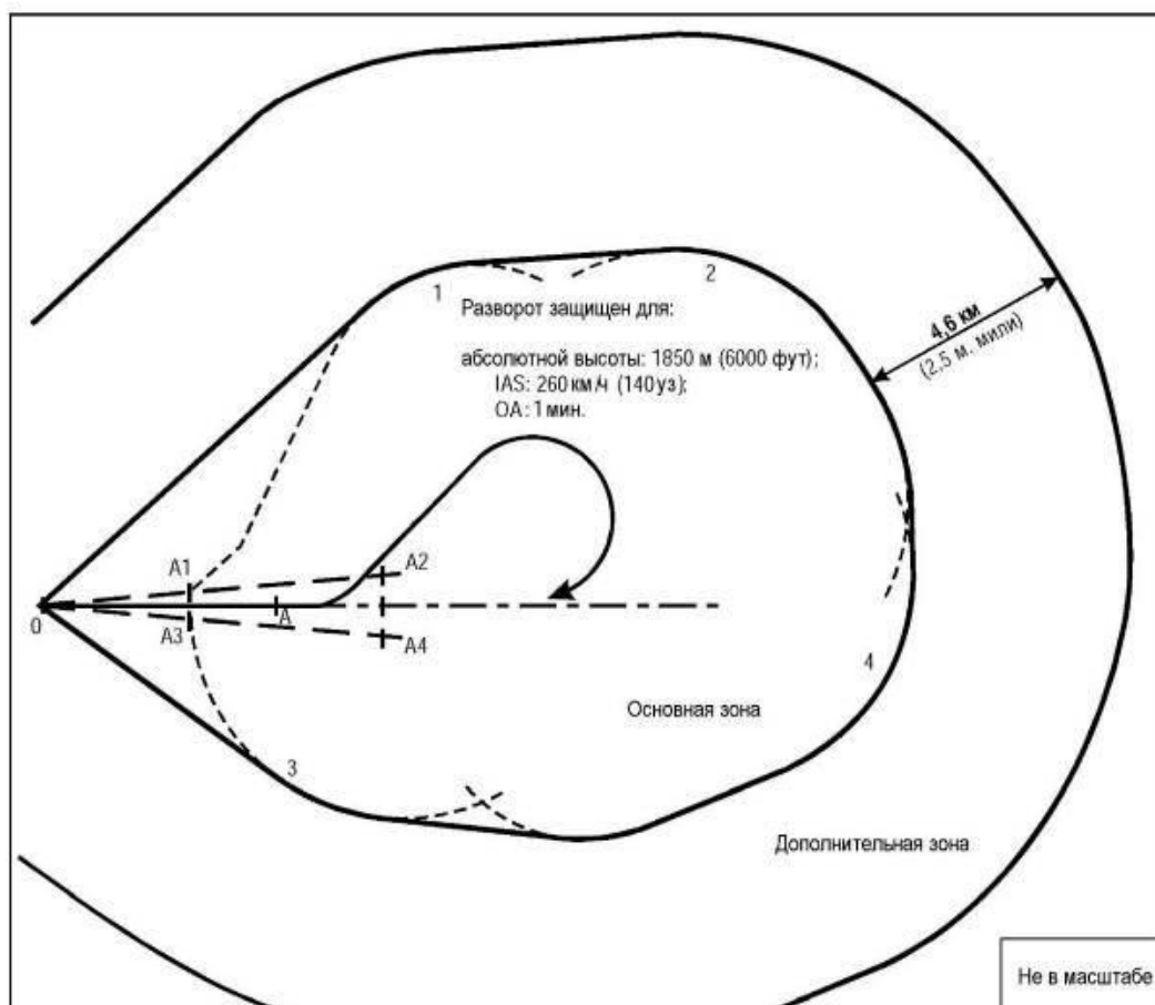
Диаграмма I-4-3-Доб С-5 - Стандартный разворот 45 - 180° по VOR
