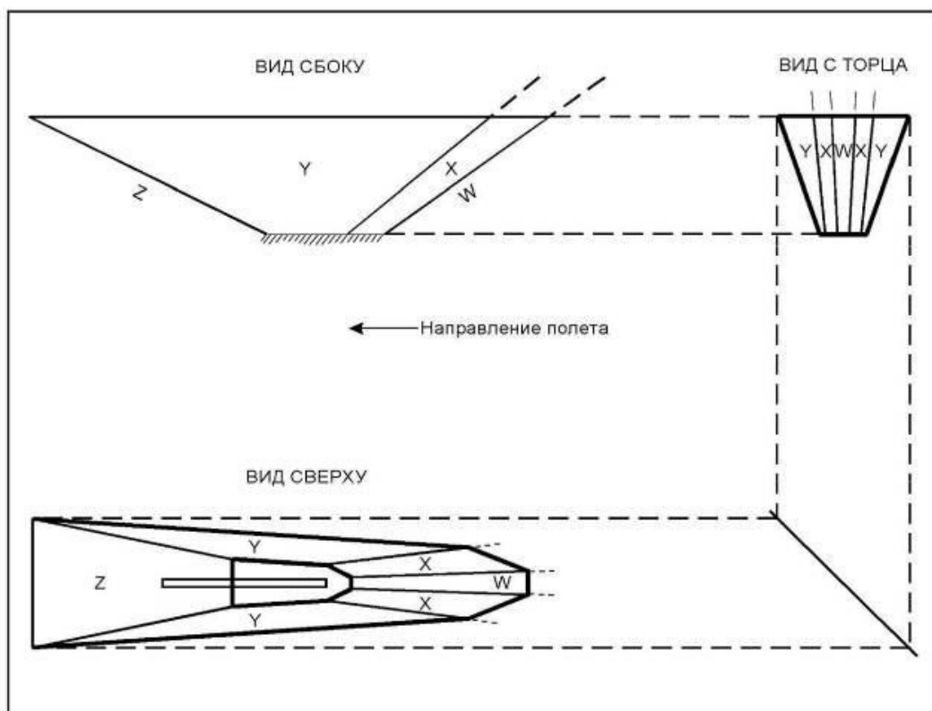
Рисунок II-1-1-8 - Поверхности II - оценки препятствий ILS
