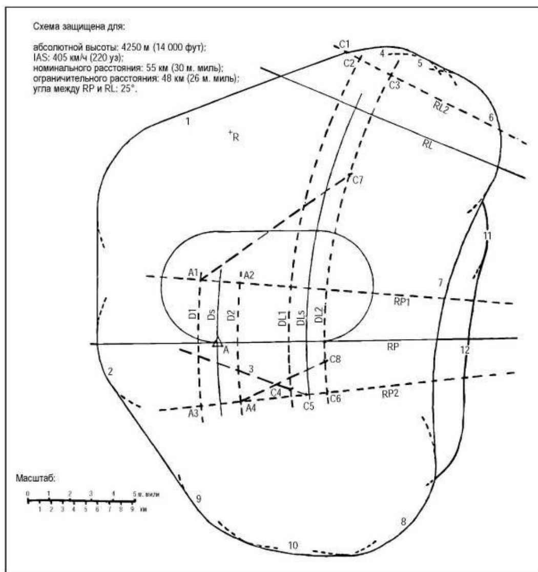
Диаграмма I-4-3-Доб C-19 - Основанная на VOR/DME схема в направлении от средства с ограничительным радиалом: основная зона и прилегающая зона для входов
