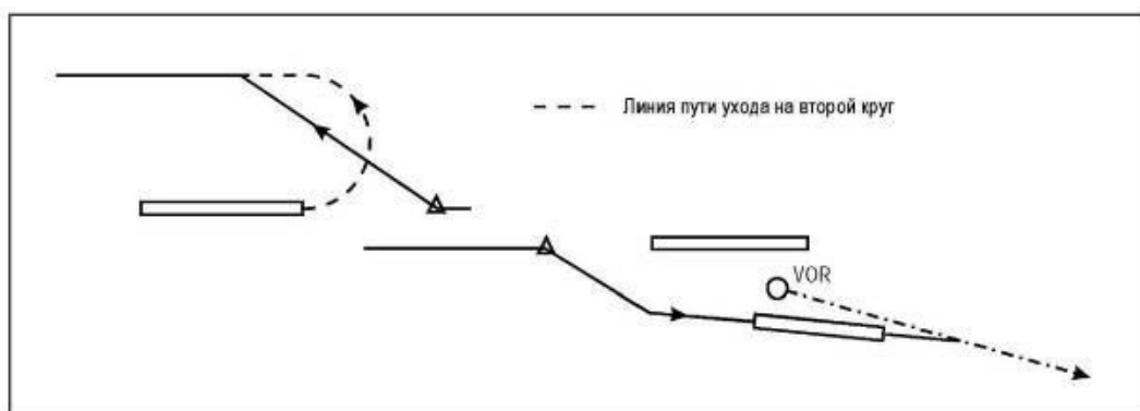
Рисунок I-4-7-Доб-3 - Предписанная линия пути ухода на второй круг
