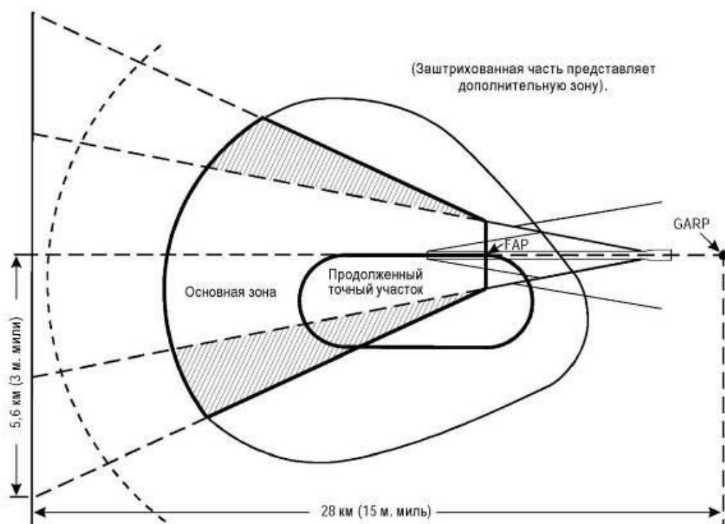
Рисунок III-3-6-3 - Зона промежуточного этапа захода на посадку. Заход на посадку по GBAS с использованием обратной схемы или схемы "ипподром"
