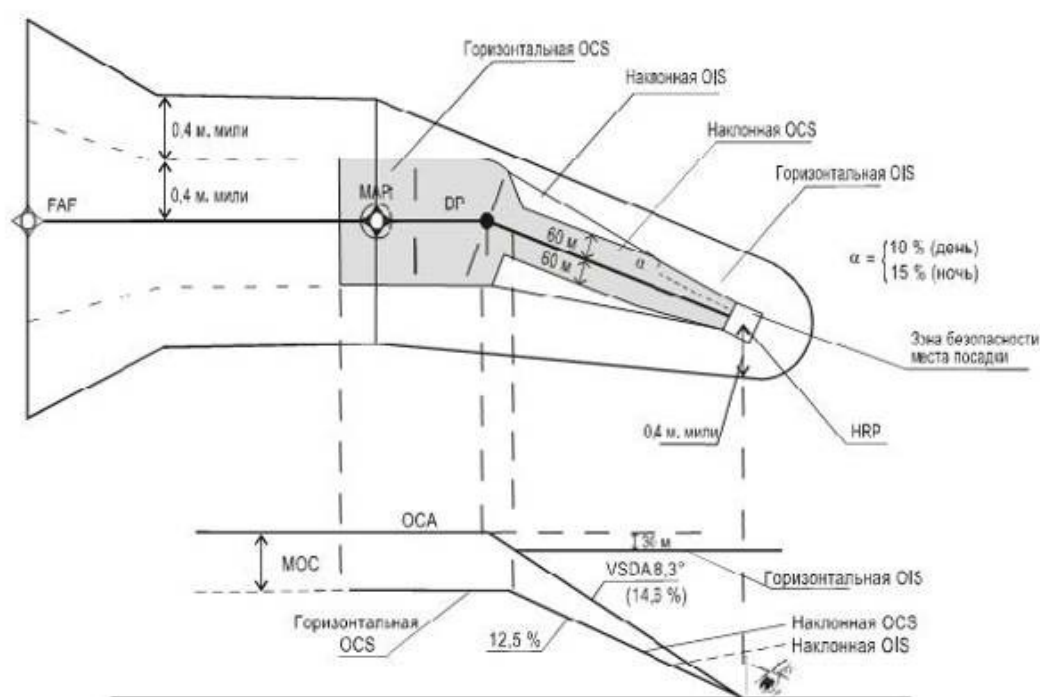
Рисунок IV-2-9 - Прямой VS с DP и с изменением курса на 30° в DP
