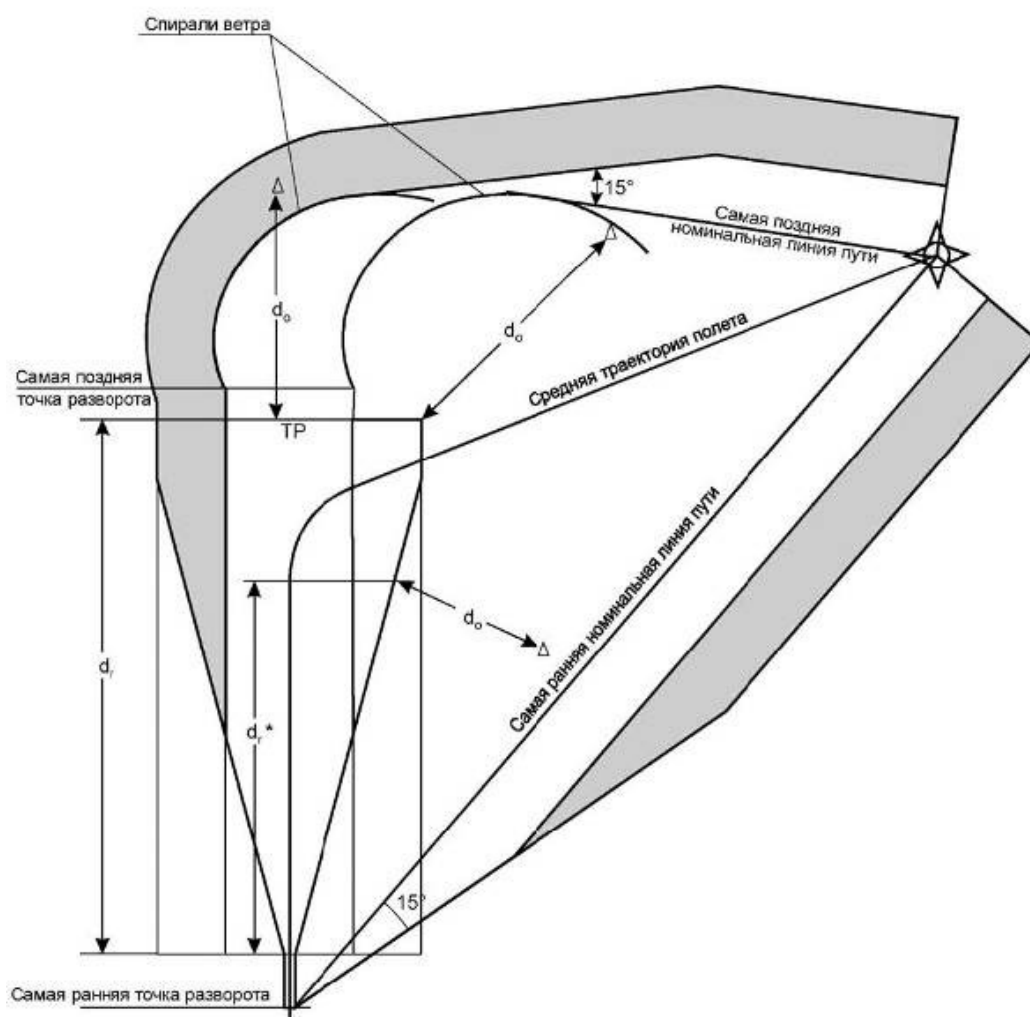
Рисунок III-2-2-9 - Разворот на абсолютной / относительной высоте, после которого следует участок DF
