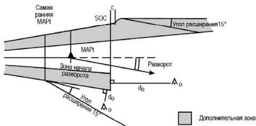
Рисунок I-4-6-10 - Разворот на 15° или менее в MAPt при уходе на второй круг
