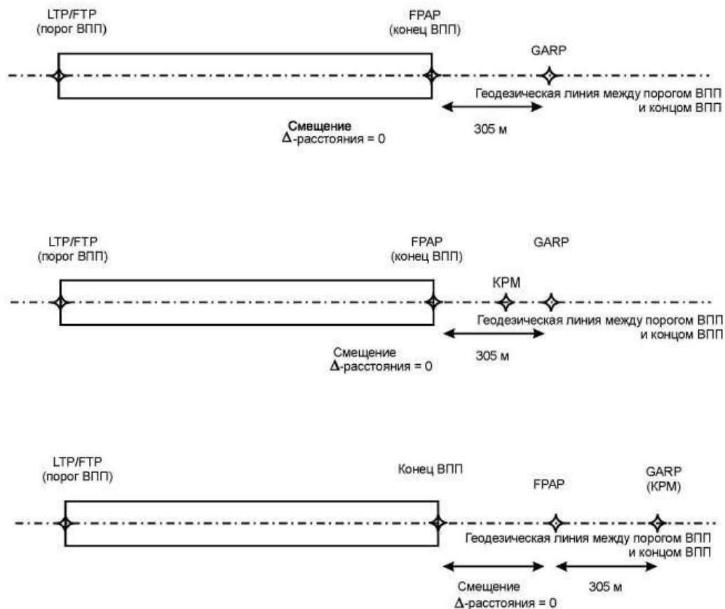
Рисунок III-2-6-3 - Местоположение FRAP (наличие ILS для захода на посадку и KPM на расстоянии более 305 м от конца ВПП)
