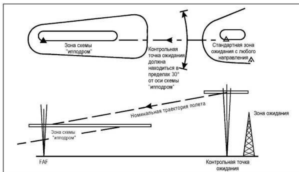
Рисунок I-4-3-Доб С-17 - Пример ограниченного входа в схему "ипподром" по ограниченной или заданной линии (линиям) пути. Зона схемы "ипподром" уменьшена соответственно входу "по оси".
