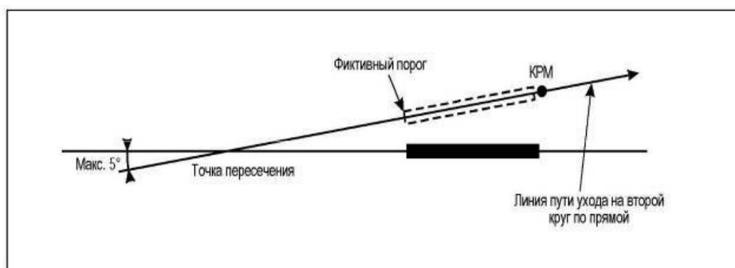
Рисунок II-1-2-1 - Смещенный курсовой радиомаяк
