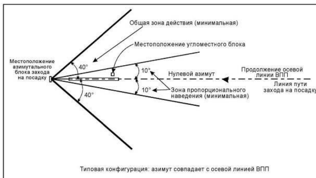
Рисунок II-1-3-1 - Конфигурация, пригодная для применения критериев MLS
