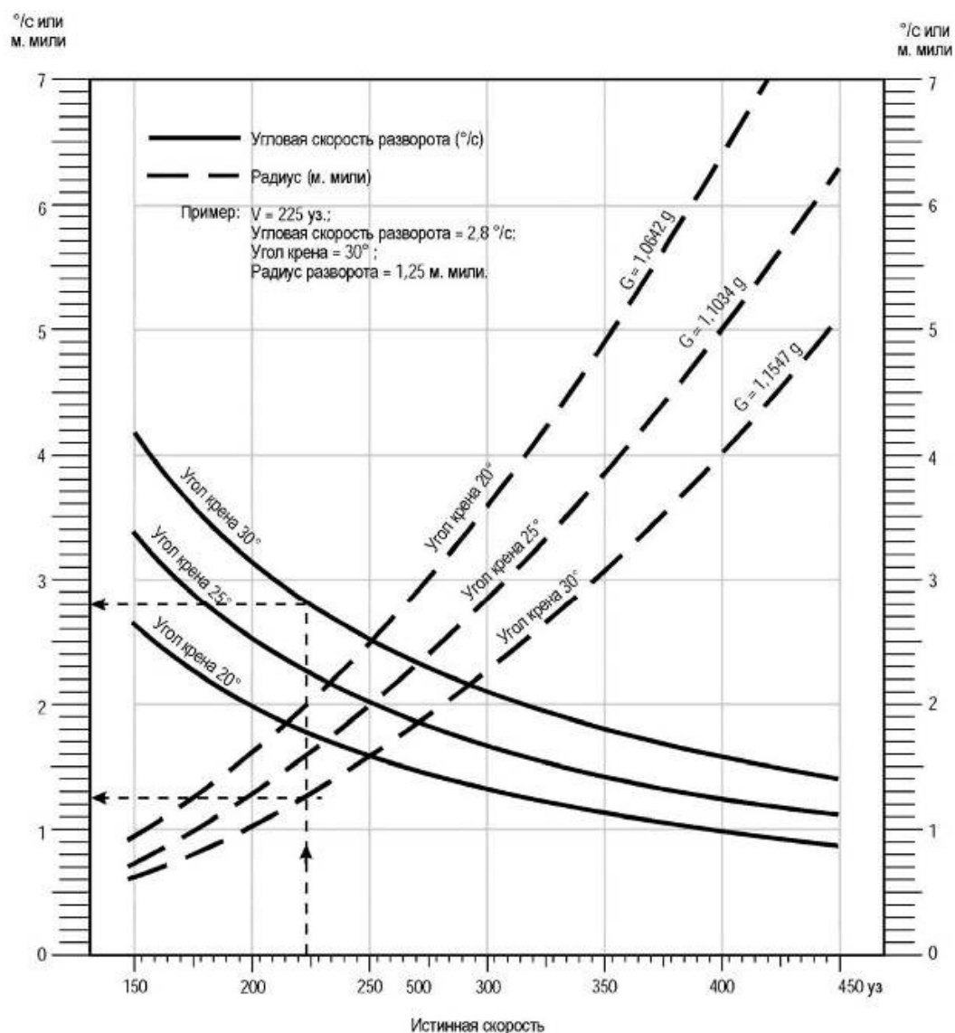
Рисунок II-4-1-Доб А-2 - Угол крена, угловая скорость разворота, радиус разворота и величины g при измерении скорости (не в единицах СИ)
