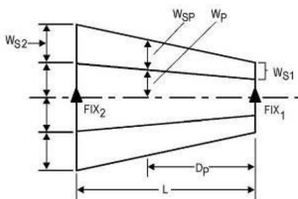
Рисунок 1-2-1-2 - Ширина дополнительной зоны
