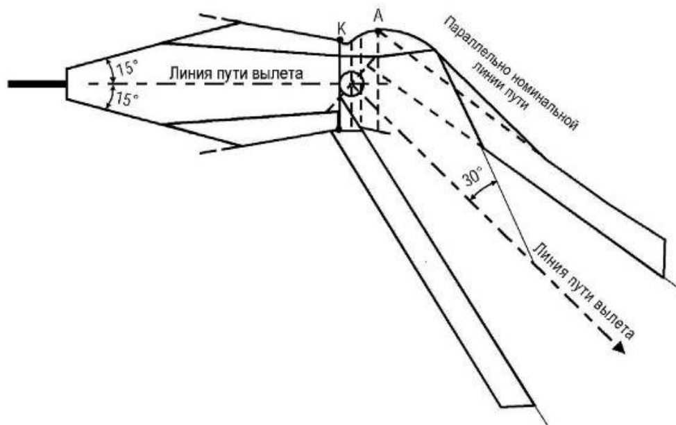
Рисунок I-3-3-11 d) - Вылет с разворотом. Разворот над навигационным средством
