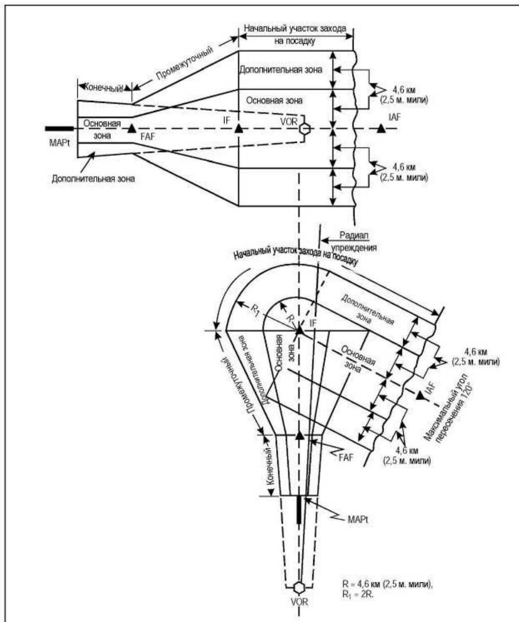
Рисунок II-2-4-2 - Типичные участки захода на посадку (прямолинейные и с разворотом >90°)
