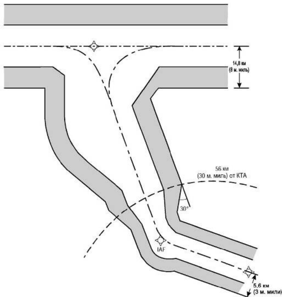
Рисунок I-4-2-6 - Критерии прибытия по GNSS, IAF в пределах 56 км (30 м. миль) от КТА
