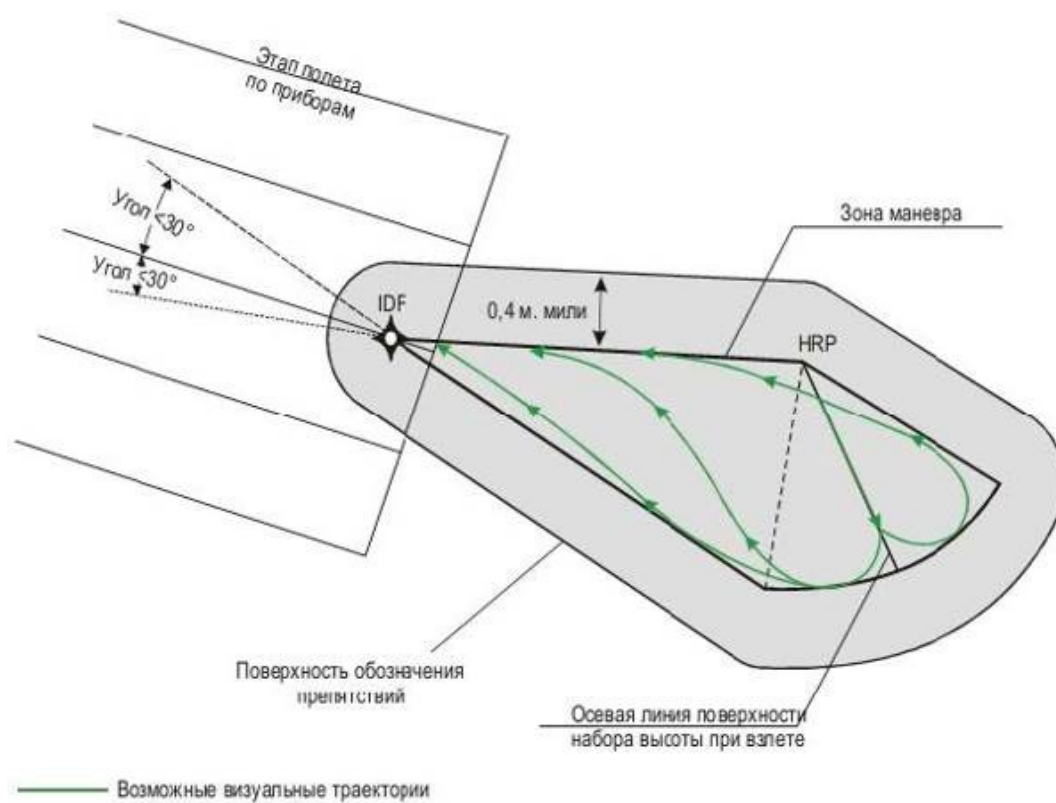
Рисунок IV-1-7 - Представление горизонтальной OIS в случае визуального участка маневрирования при заданной осевой линии поверхности набора высоты при взлете
