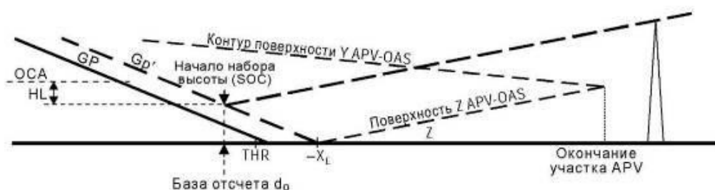
Рисунок III-3-5-9 - Запас высоты над препятствиями при уходе на второй круг по прямой
