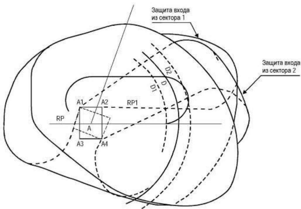
Рисунок III-3-7-Доб А-9 - Схема ожидания RNAV, включая защиту схем входа для системы RNAV без функции ожидания. Участок удаления определяется по расстоянию
