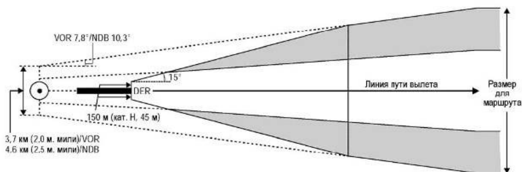
Рисунок I-3-3-4 - Вылет по прямой. Навигационное средство впереди
