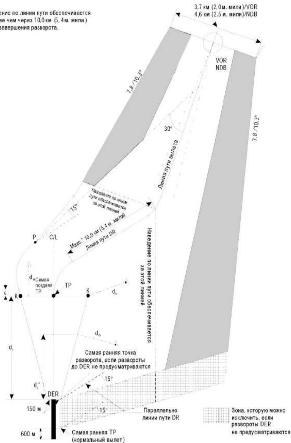
Рисунок I-3-3-10 - Вылет с разворотом: разворот на абсолютной высоте
