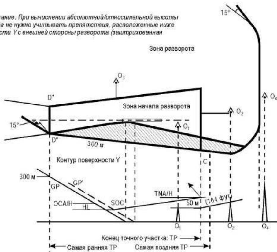
Рисунок III-3-6-16 - Разворот на заданной абсолютной высоте
