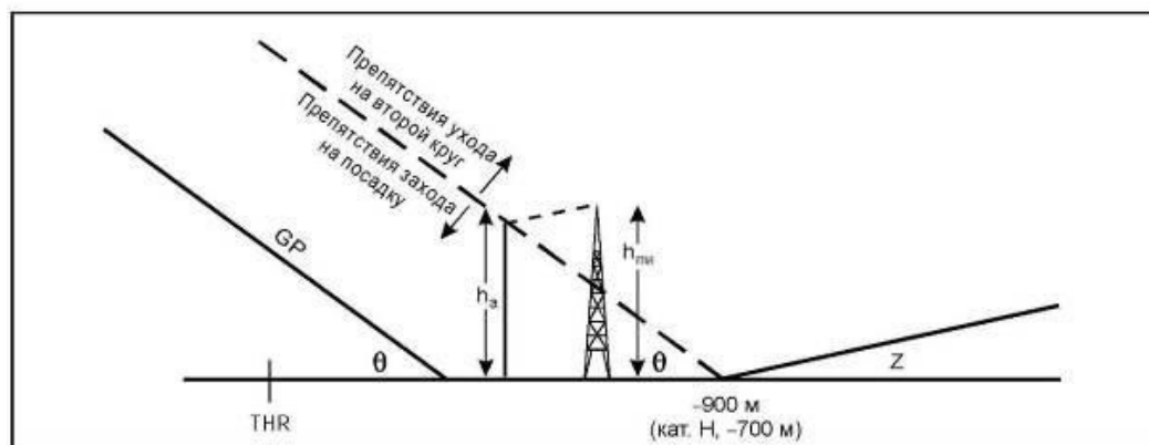
Рисунок II-1-1-14 - Препятствие ухода на второй круг, расположенное до дальности - 900 м
