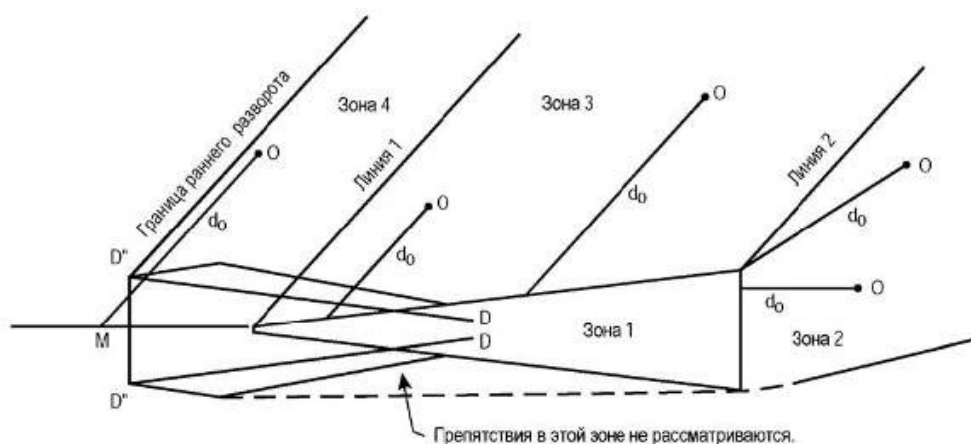
Рисунок II-1-1-Доб А-6 - Измерение расстояний d_0 до препятствий (разворот менее чем на 75^\circ )
