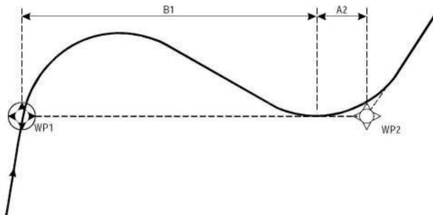
Рисунок III-2-1-5 - Точка пути "флайовер", а затем точка пути "флай-бай"
