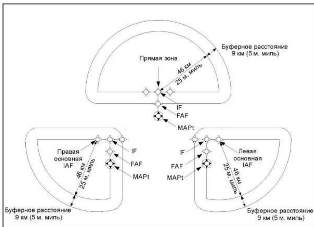
Рисунок III-2-4-2 - Т-образная конфигурация зон ТАА
