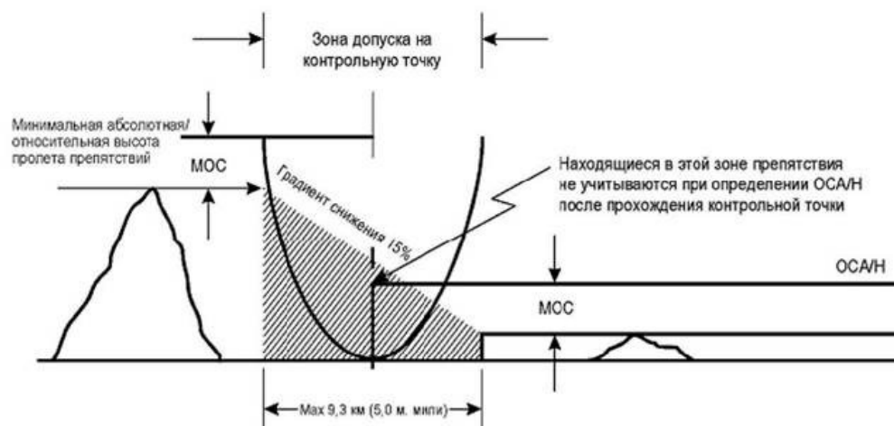
Рисунок 1-2-2-11 - Зона, в которой не требуется учитывать препятствия
