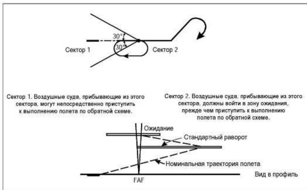
Рисунок I-4-3-6 - Пример прибытия с любого направления с использованием схемы ожидания совместно с обратной схемой
