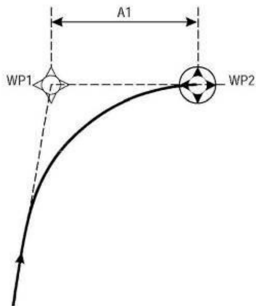
Рисунок III-2-1-3 - Точка пути "флай-бай", затем точка пути "флайовер"
