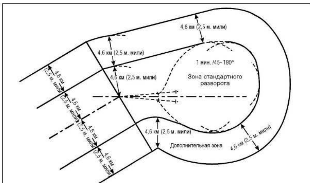
Рисунок I-4-3-Доб С-6 - Сопряжение зон начальных участков и зон стандартного разворота
