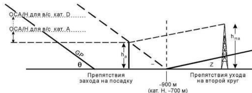
Рисунок III-3-6-12 - Препятствие ухода на второй круг, расположенное за дальностью - 900 м
