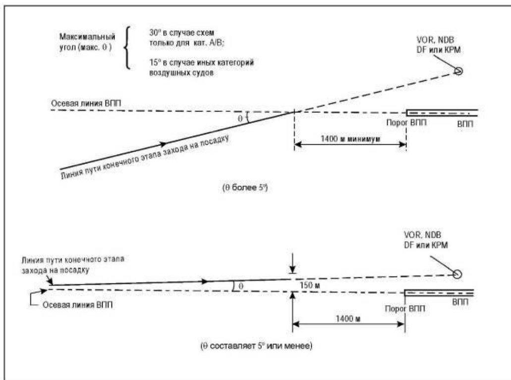
Рисунок I-4-5-1 - Выравнивание направления конечного этапа захода на посадку по прямой
