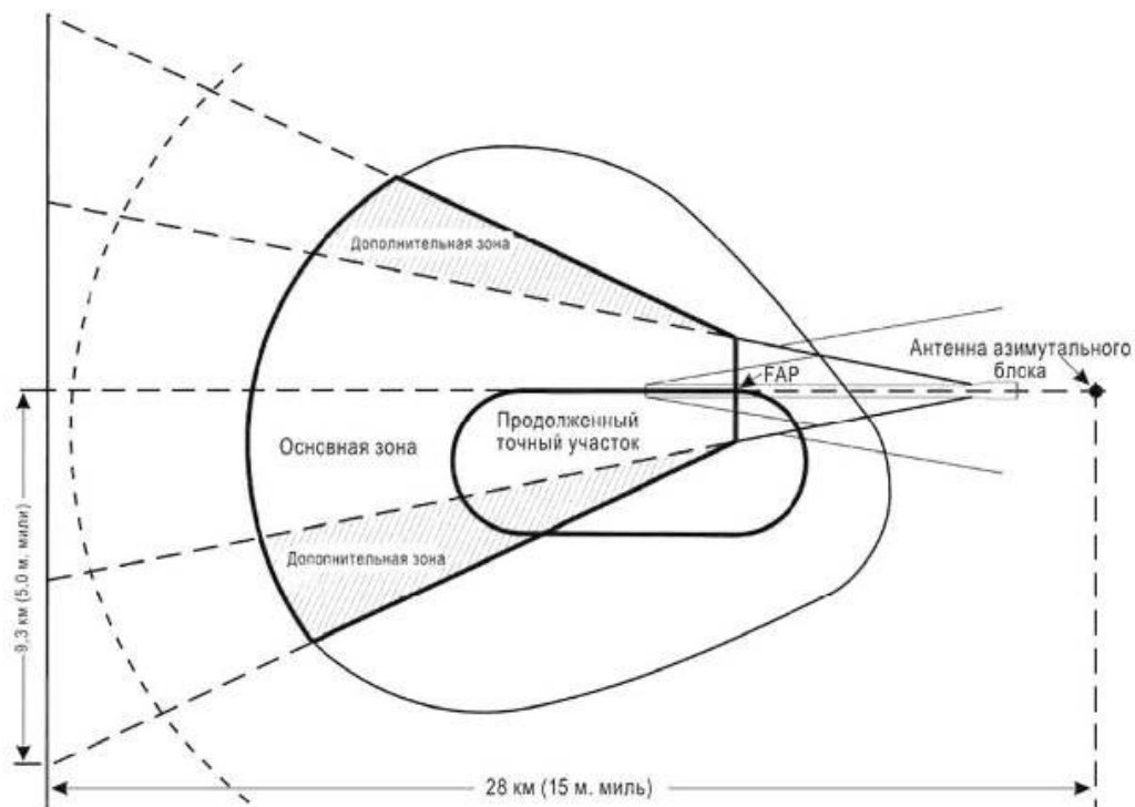
Рисунок II-1-3-5 - Зона промежуточного этапа захода на посадку. Заход на посадку по MLS с использованием обратной схемы "ипподром"
