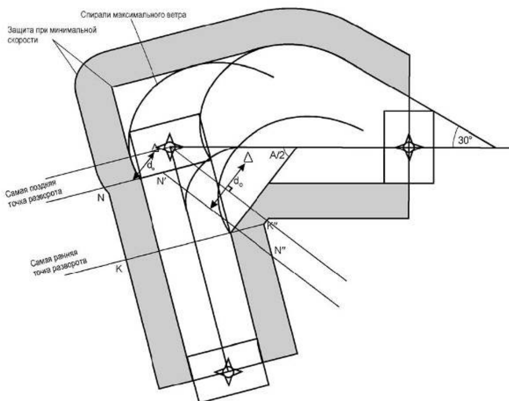
Рисунок III-3-2-3 - Разворот в точке пути "флай-бай"
