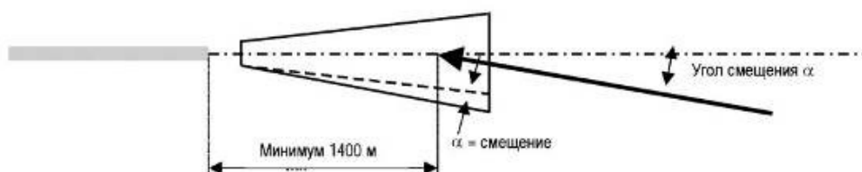
Рисунок I-4-5-8 - Вид в плане; поверхность визуального участка. Смещенный конечный участок захода на посадку с пересечением осевой линии ВПП
