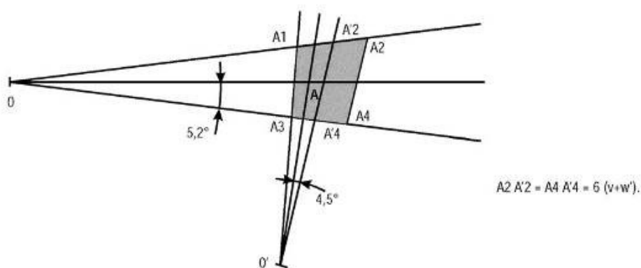
Рисунок I-4-3-Доб С-3 - VOR в 0 и VOR в 0'
