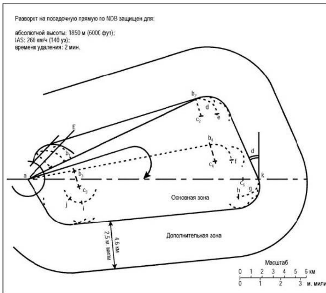
Диаграмма I-4-3-Доб С-1 - Разворот по NDB на посадочную прямую
