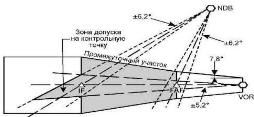
Рисунок 1-2-2-9 - Зона, в которой обеспечивается запас высоты над препятствиями
