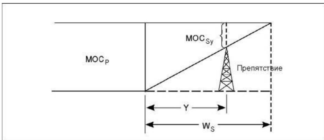
Рисунок 1-2-1-3 - Запас высоты над препятствиями в дополнительных зонах
