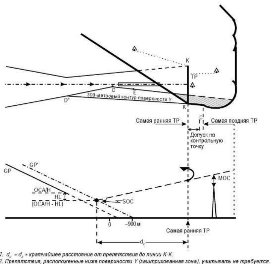
Рисунок III-3-6-17 - Разворот с заданной TP (при наличии контрольной точки TP)
