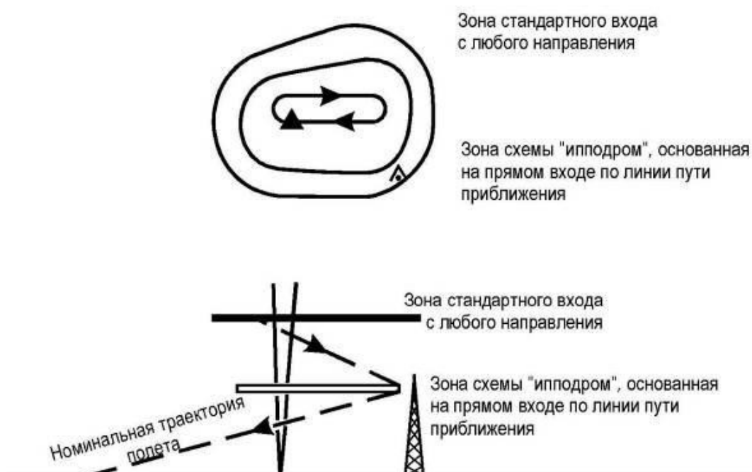
Рисунок I-4-3-Доб С-16 - Пример входа в схему "ипподром" с использованием стандартного входа с любого направления на большей абсолютной высоте. Зона "ипподром" уменьшена соответственно входу "по оси".
