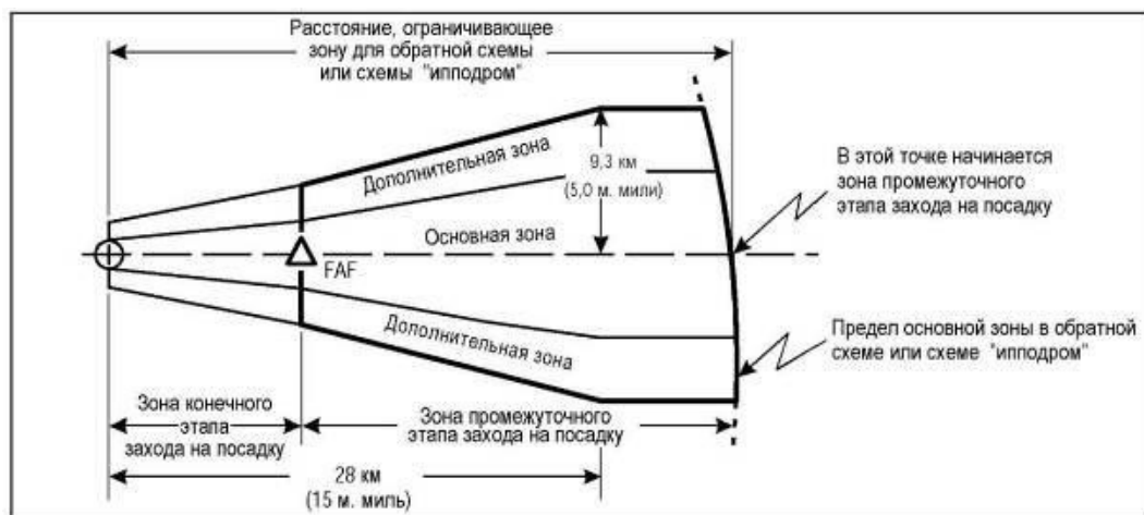
Рисунок I-4-4-3 - Зона промежуточного этапа захода на посадку в пределах обратной схемы или схемы "ипподром", основанных на FAF, а не на навигационном средстве
