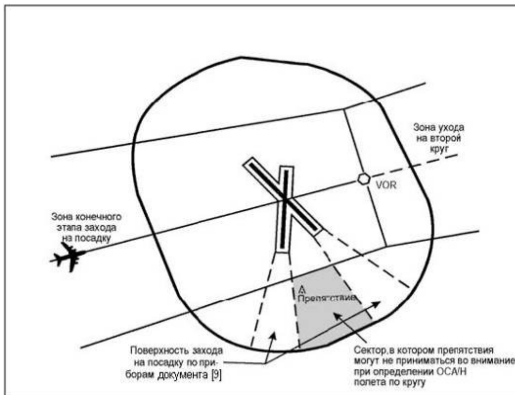
Рисунок I-4-7-3. Зона визуального маневрирования (полета по кругу). Запас высоты над препятствиями
