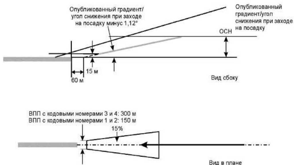
Рисунок I-4-5-7-b) - Поверхность визуального участка. Другие схемы захода на посадку; обычный заход на посадку по прямой
