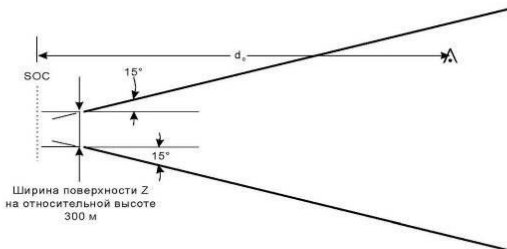
Рисунок III-3-6-1 -. Конечный участок ухода на второй круг по прямой
