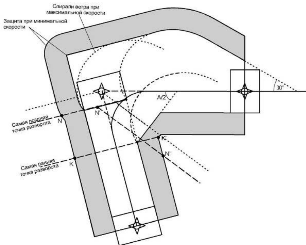
Рисунок III-2-2-4 - Линия N-N'-N": разворот в точке пути "флай-бай" под углом > 90^\circ
