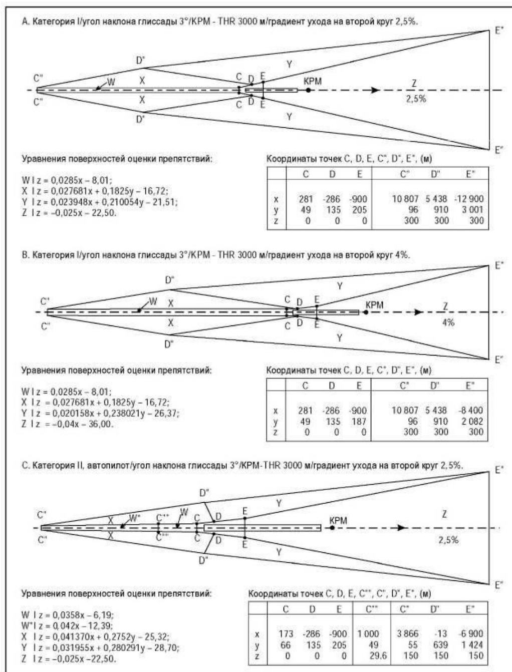
Рисунок II-1-1-11 - Типичные контуры OAS для ВС стандартных размеров
