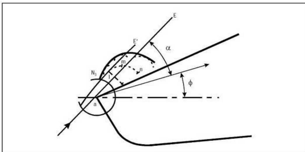
Диаграмма I-4-3-Доб С-2 - Защита входа I в разворот на посадочную прямую
