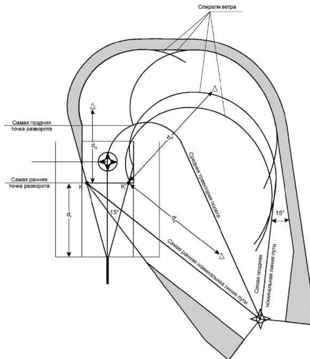
Рисунок III-2-2-7 - Разворот в точке пути "флайовер", после которого следует участок DF. Большой угол разворота
