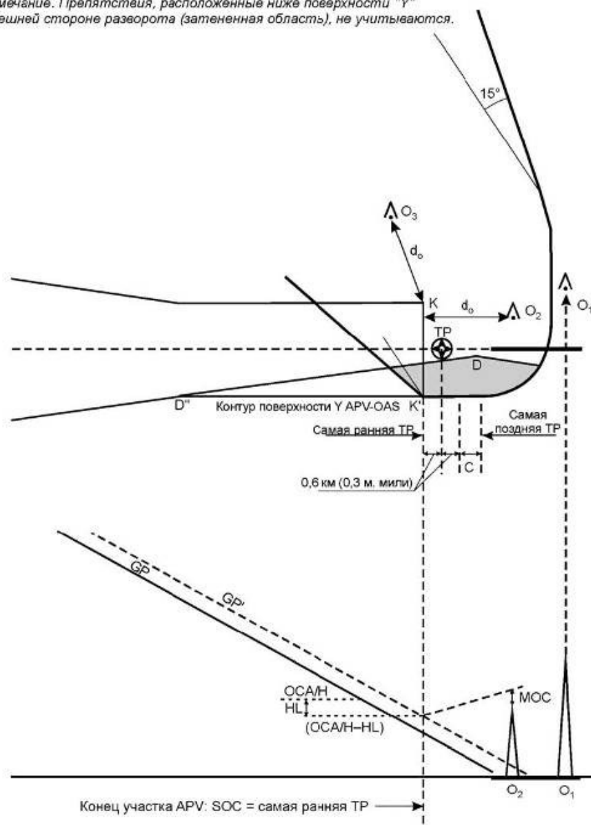
Рисунок III-3-5-10 - Разворот в заданной ТР (точка пути "флайвер") после порога ВПП
