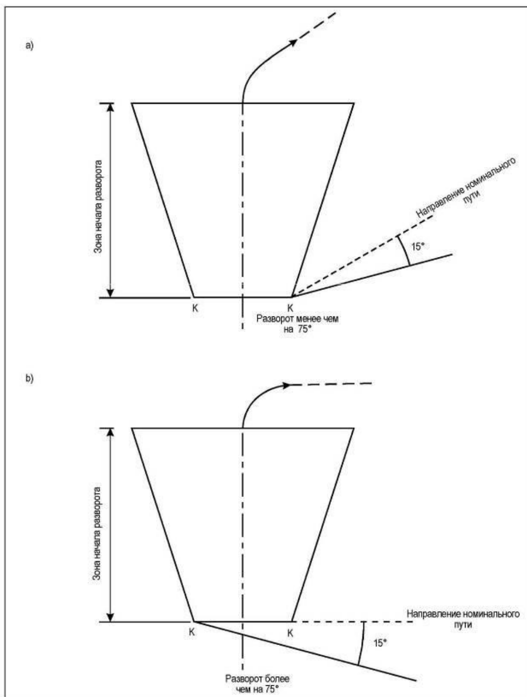
Рисунок 1-2-3-1 - Защита внутренней границы разворота
