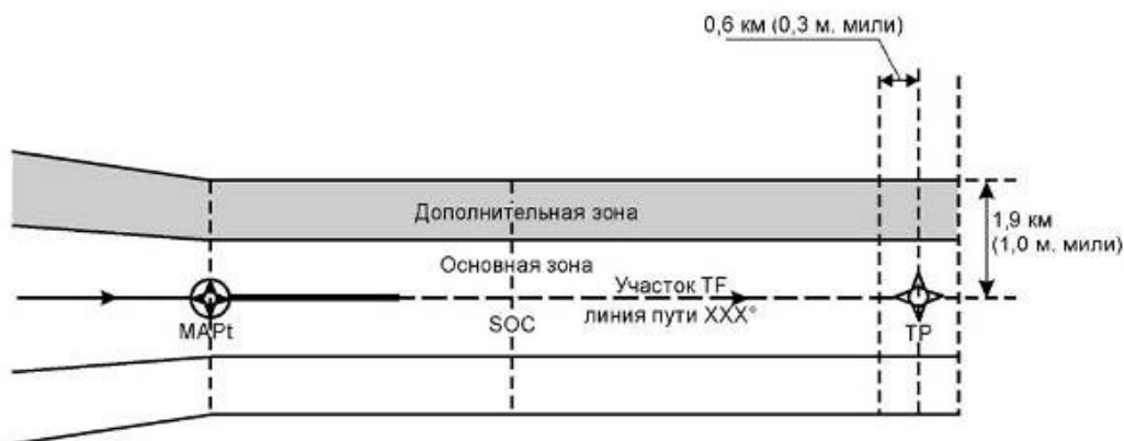
Рисунок III-3-3-4 - Участок ухода на второй круг по прямой применительно к SBAS
