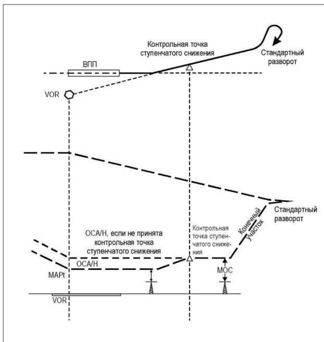
Рисунок II-2-3-2 - Контрольная точка ступенчатого снижения с двойной ОСА/Н
