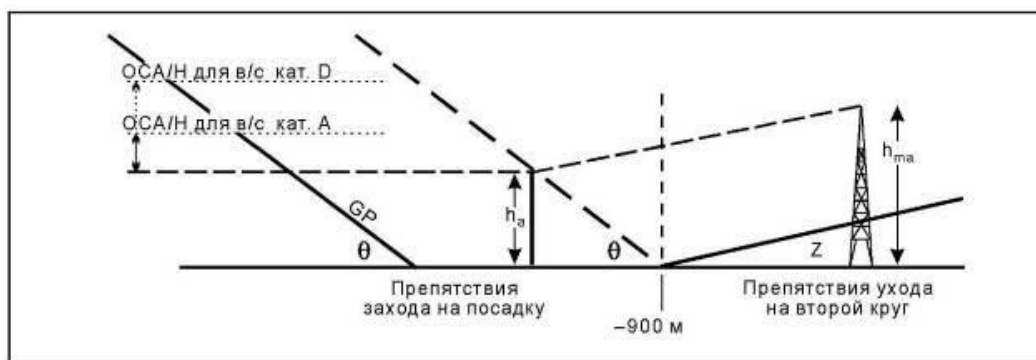
Рисунок II-1-3-14 - Препятствие ухода на второй круг, расположенное за дальностью - 900 м
