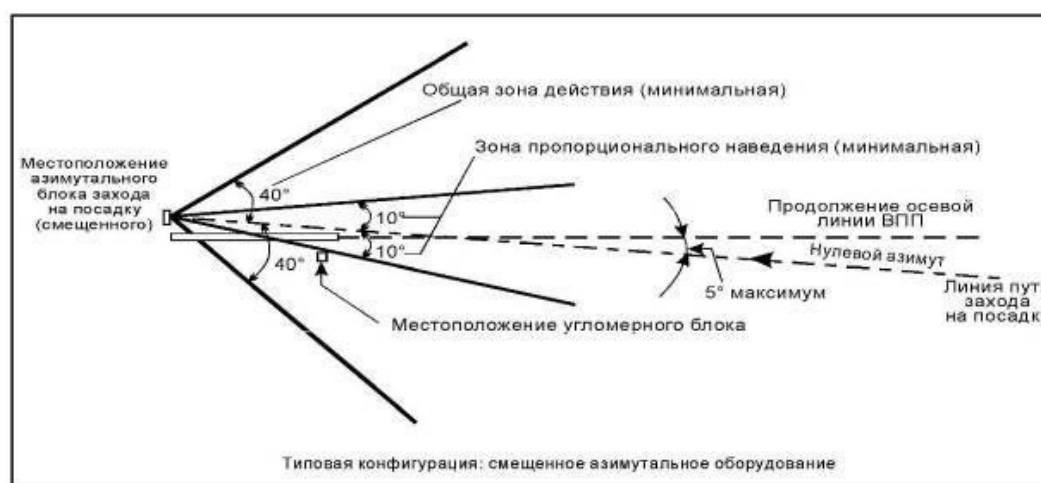
Рисунок II-1-4-1 - Конфигурация, пригодная для применения критериев MLS
