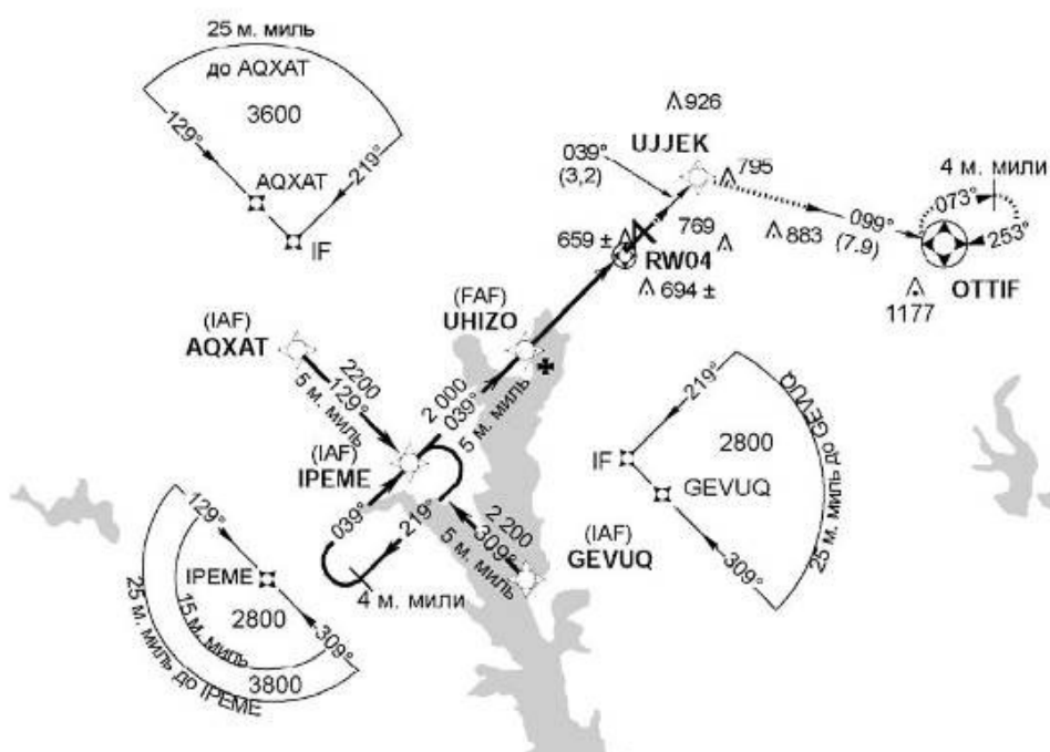
Рисунок III-2-4-5 - Пиктограммы образного расположения ТАА без центрального начального этапа
