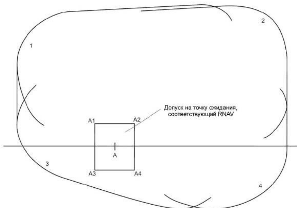
Рисунок III-3-7-Доб А-3 - Основная зона RNAV для системы RNAV с функцией ожидания
