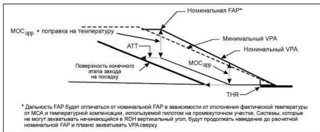
Рисунок III-3-4-4 - Поверхность конечного этапа захода на посадку с применением VNAV и минимальный VPA
