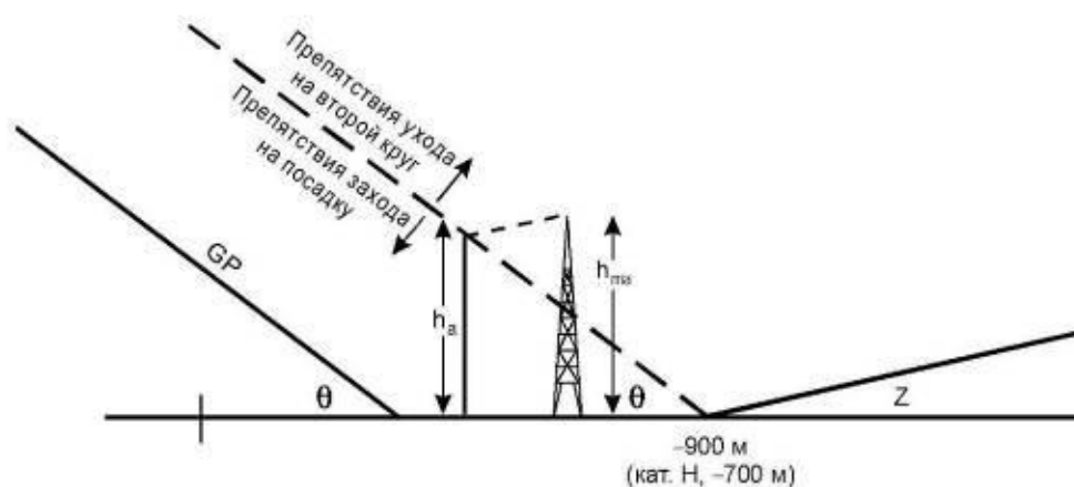
Рисунок III-3-6-13 - Препятствие ухода на второй круг, расположенное до дальности - 900 м
