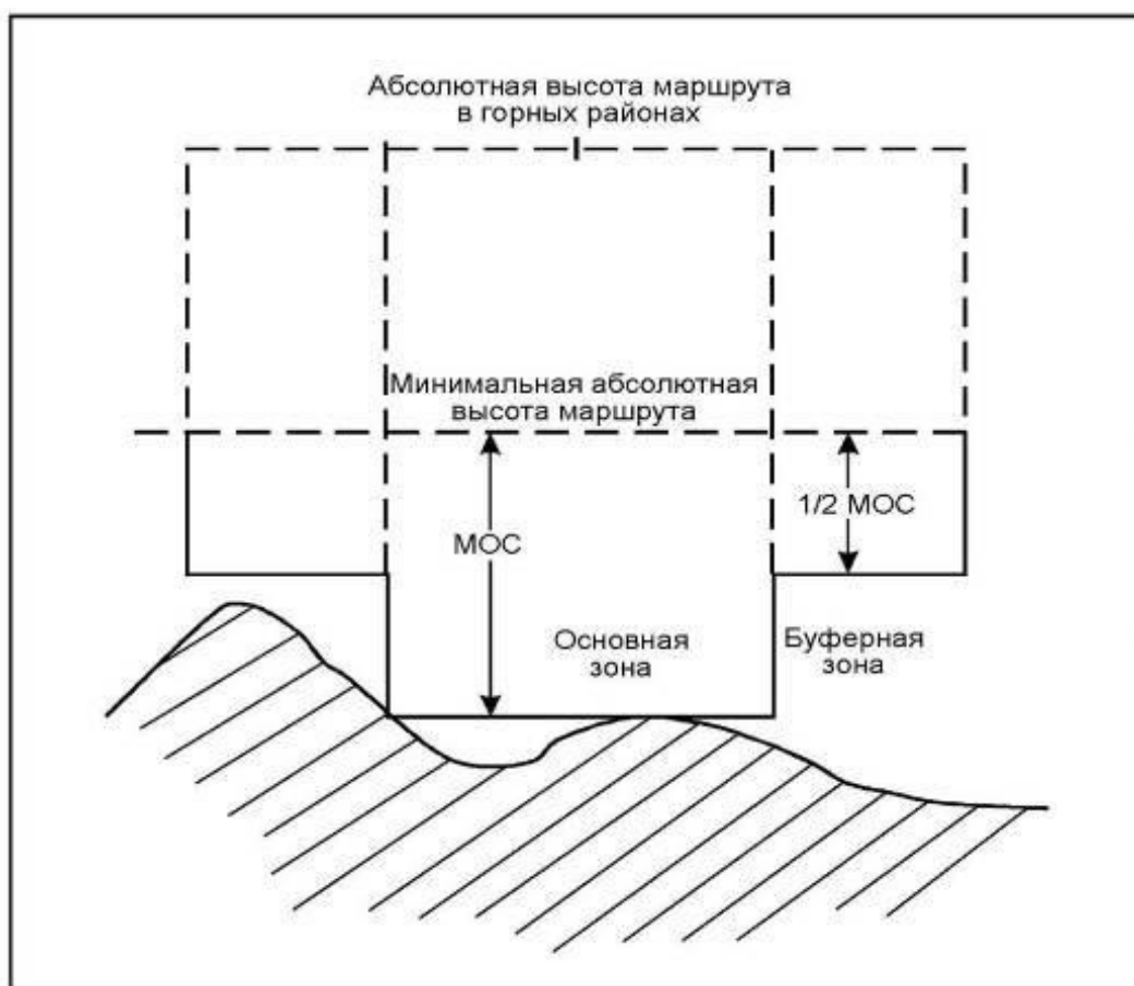
Рисунок II-3-1-1 - МОС при полете по маршруту: основная и буферная зоны
