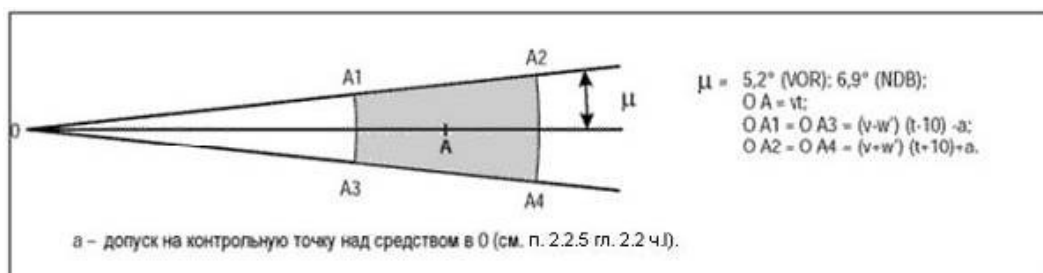
Рисунок I-4-3-Доб С-1 - VOR или NDB в 0: время от 0 до A
