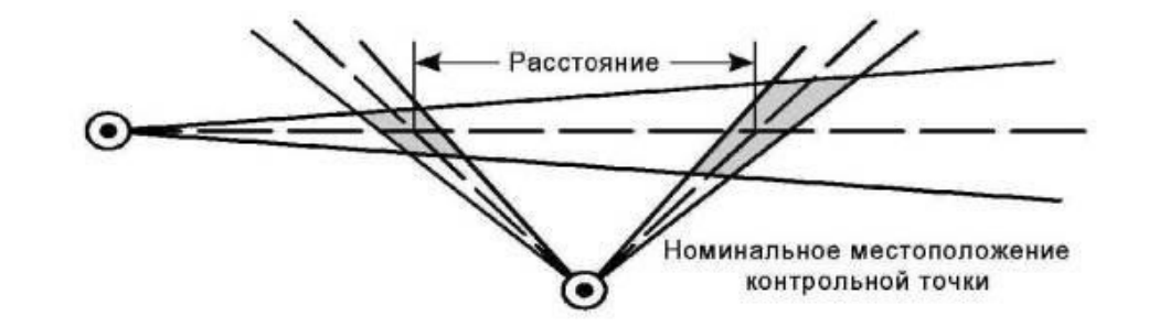
Рисунок 1-2-2-8 - Расстояние между контрольными точками
