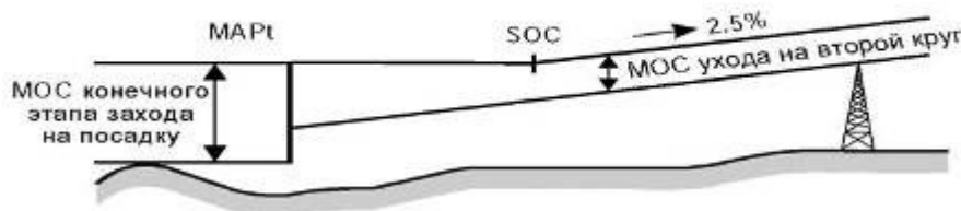
Рисунок I-4-6-5. Случай, когда продолжение поверхности ухода на второй круг полностью перекрывает начальный этап ухода на второй круг
