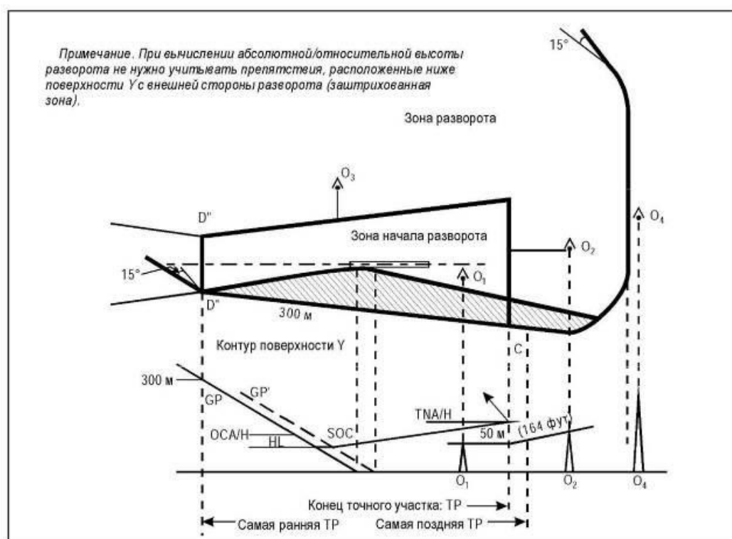
Рисунок II-1-1-17 - Разворот на заданной абсолютной высоте
