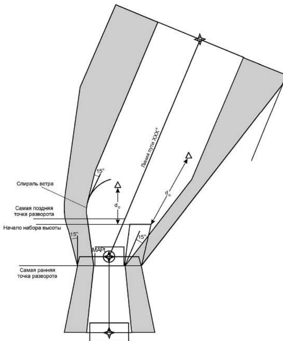
Рисунок III-2-2-12 - Разворот при уходе на второй круг в МАРt, после которого следует участок TF или CF
