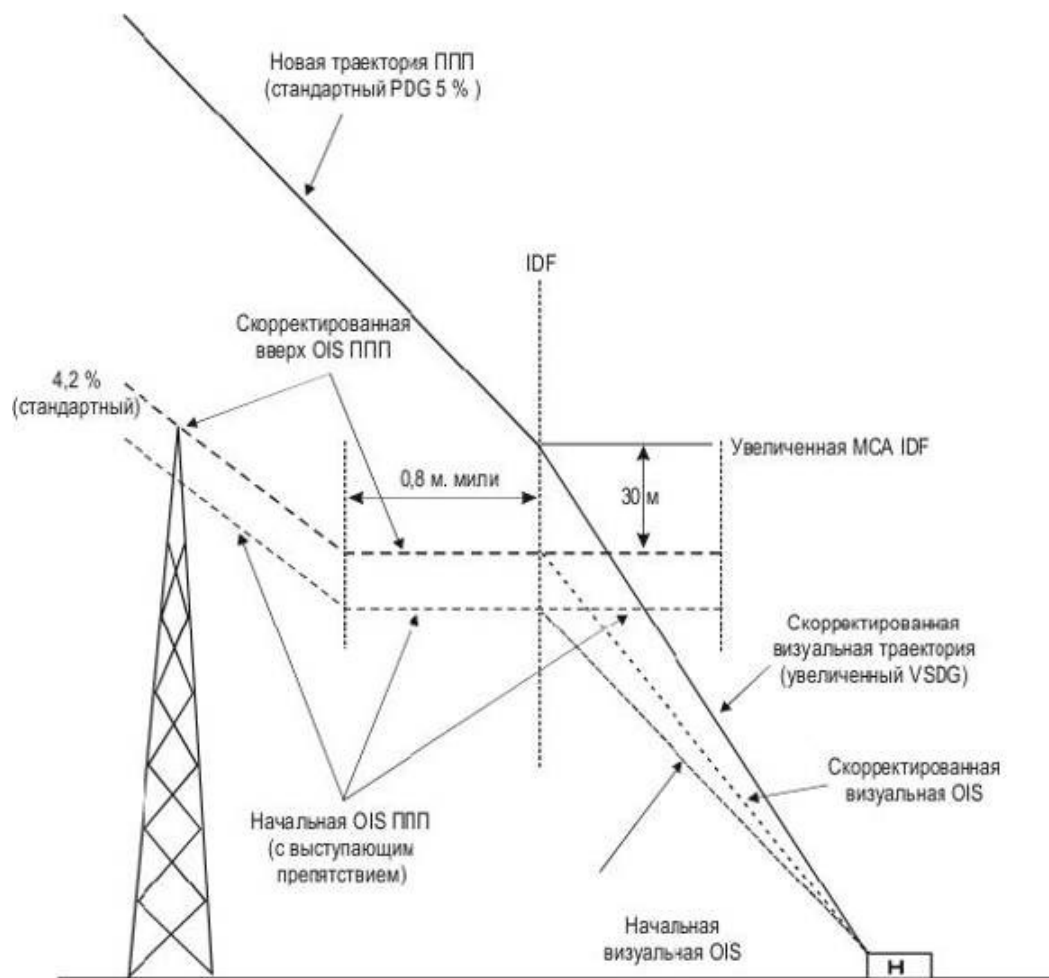
Рисунок IV-1-4 - Компенсация возвышения препятствия на участке полета по приборам путем увеличения MCA IDF
