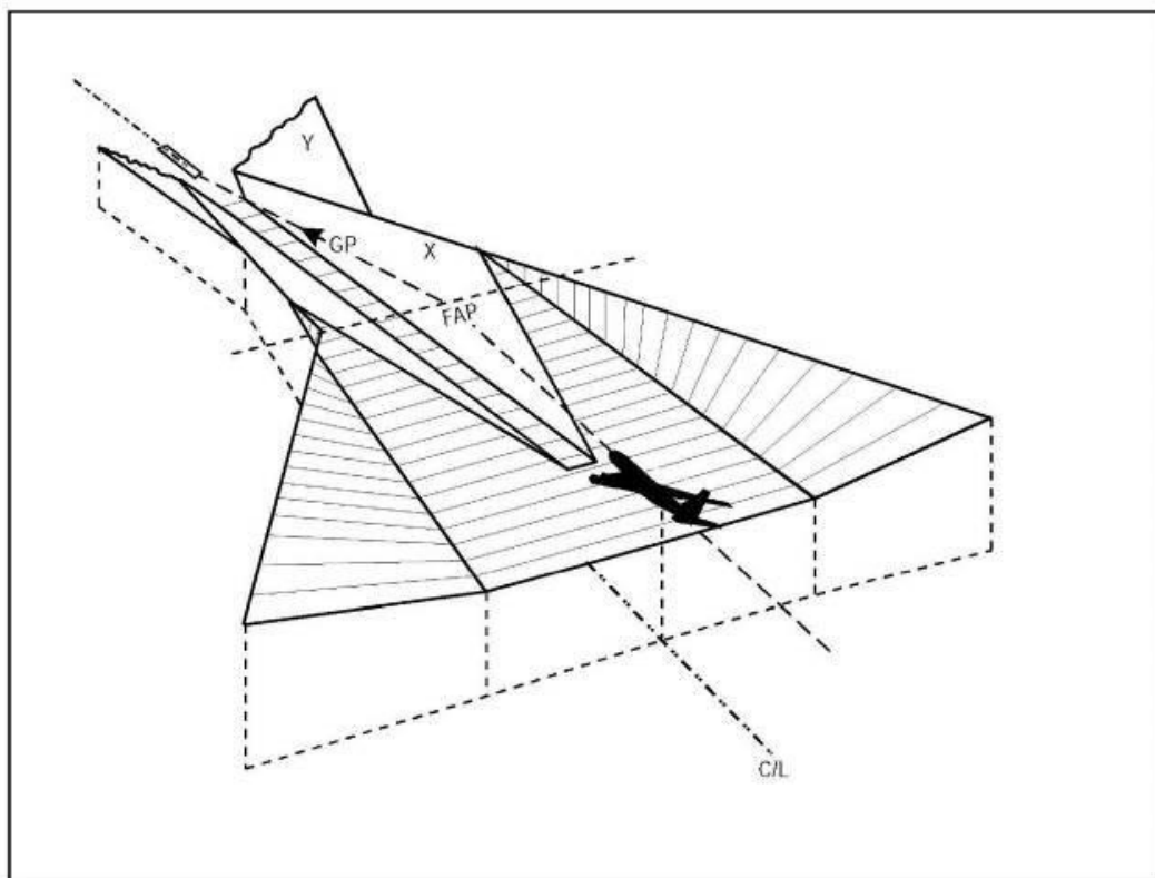
Рисунок II-1-3-2 - Сопряжение конечного участка захода на посадку с предшествующим участком: вид в перспективе
