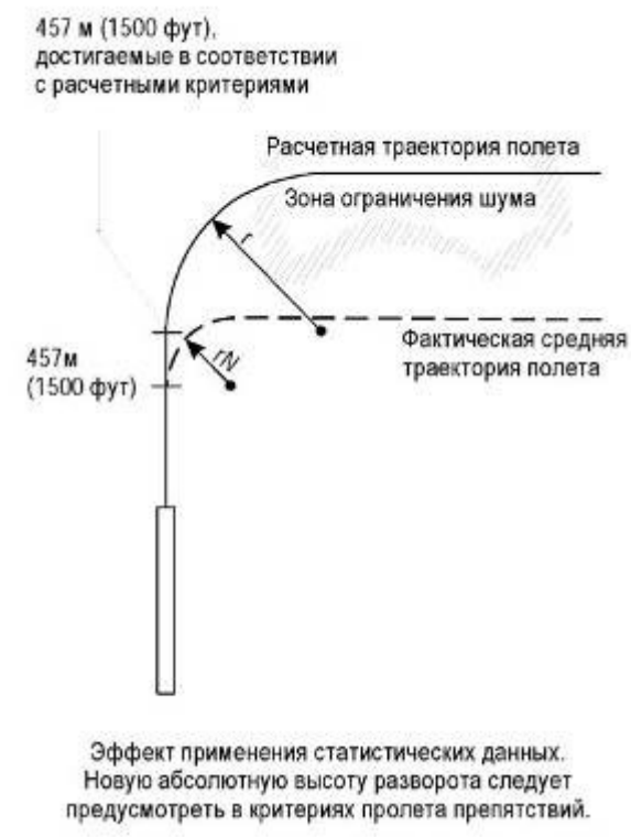
Рисунок I-3-3-Доб-2 - Разворот на заданной абсолютной высоте разворота. Схема с применением статистических данных
