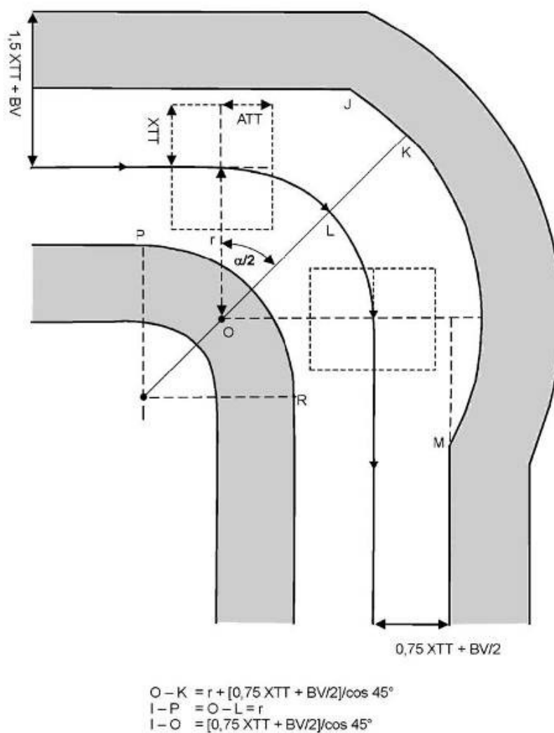
Рисунок III-2-2-13 - Защита разворота RF
