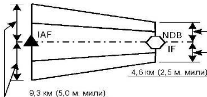
Рисунок I-4-3-Доб В-4 - Случай, когда IAF находится на расстоянии менее или равном 25,5 км (13,8 м. мили) от NDB
