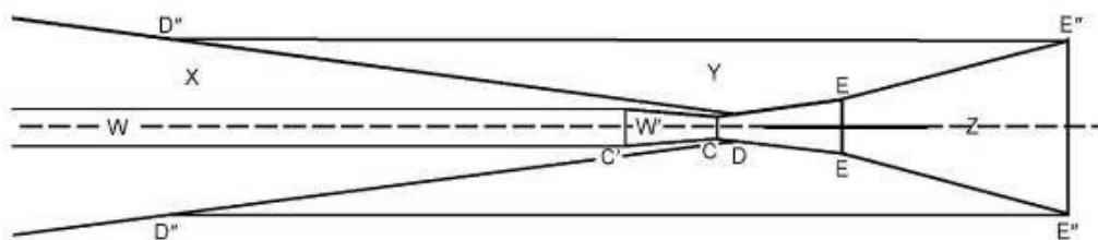
Рисунок III-3-5-5 - Типичные контуры APV I-OAS SBAS для воздушных судов стандартного размера
