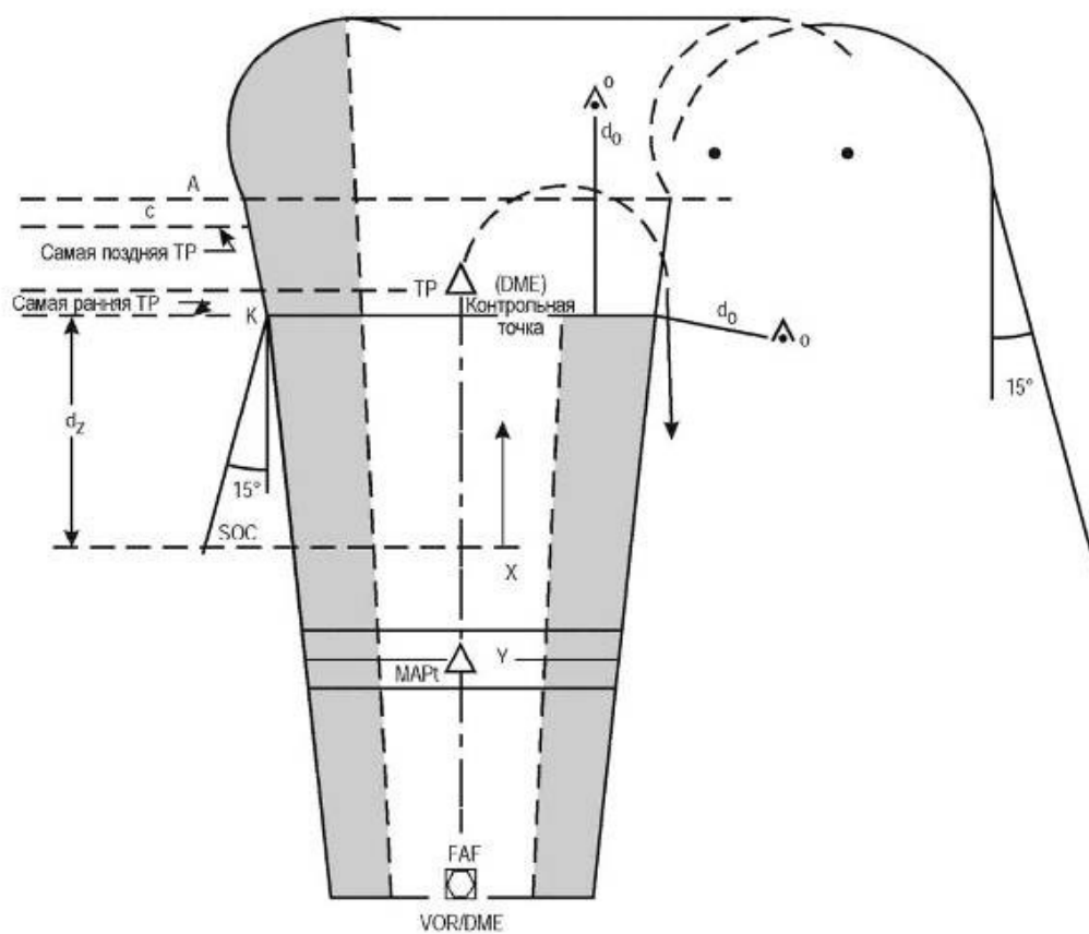
Рисунок I-4-6-16 - Уход на второй круг с разворотом на 180^\circ при наличии DME в качестве контрольной точки TP
