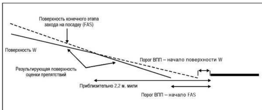
Рисунок III-3-4-5 - Вид поверхности оценки препятствий сбоку для защиты воздушных судов, оборудованных вертикальной угловой шкалой
