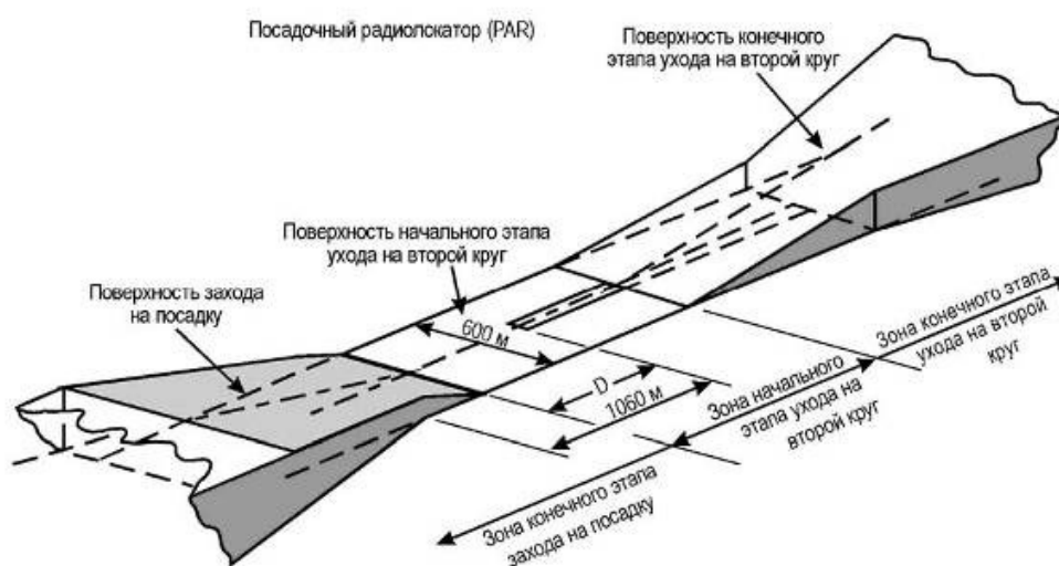
Рисунок II-1-5-2 - Зоны и поверхности конечного этапа захода на посадку и ухода на второй круг
