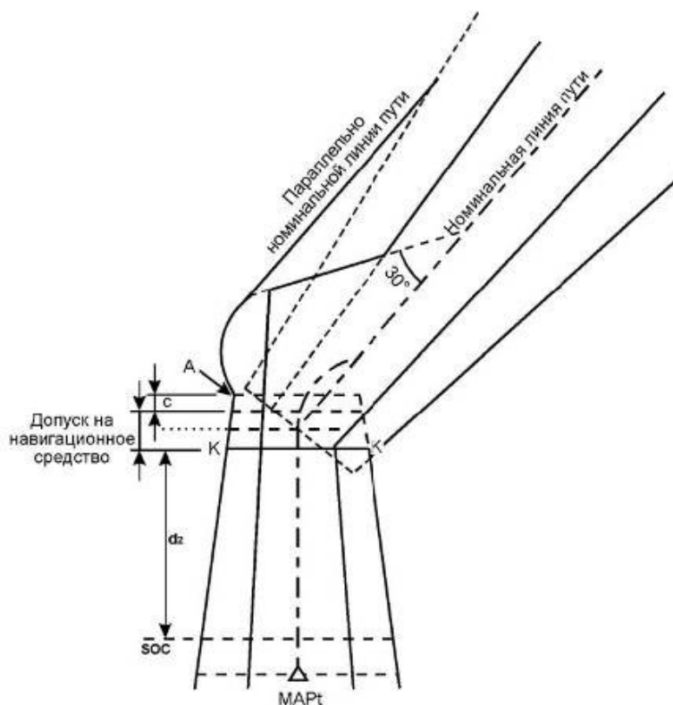
Рисунок I-4-6-19 - Уход на второй круг с разворотом над навигационным средством
