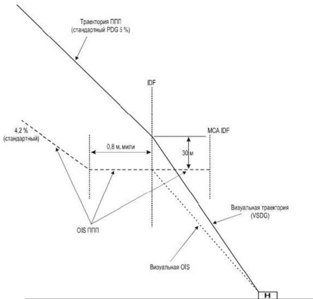
Рисунок IV-1-1 - Вертикальное сопряжение визуального участка OIS и ППП
