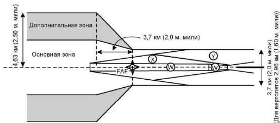
Рисунок. III-3-5-1b) - Зона промежуточного участка захода на посадку (полностью основанная на SBAS). FAF ближе к порогу ВПП (ширина поверхности X в FAF меньше чем 3,7 км (2 м. мили))
