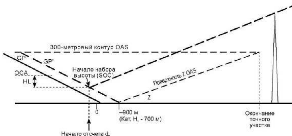
Рисунок III-3-6-15 - Запас высоты над препятствиями при уходе на второй круг по прямой
