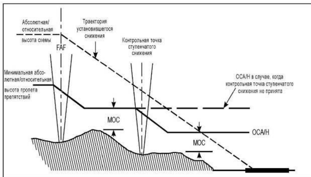
Рисунок 1-2-2-10 - Контрольная точка ступенчатого снижения с двойной ОСА/Н
