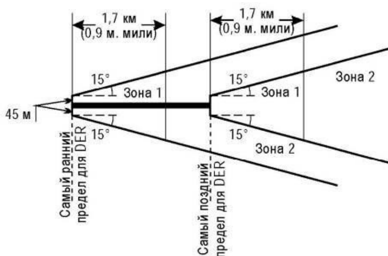
Рисунок 1-3-2-1 - Начало схемы вылета: вертолеты
