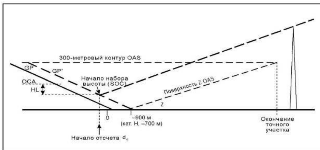
Рисунок II-1-1-16 - Запас высоты над препятствиями при уходе на второй круг по прямой
