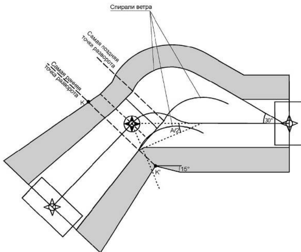
Рисунок III-2-2-3 - Разворот в точке пути "флайовер" с участком TF после разворота: дополнительная зона внутри на внутренней стороне разворота
