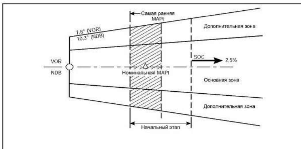
Рисунок I-4-6-6 - Зона ухода на второй круг по прямой
