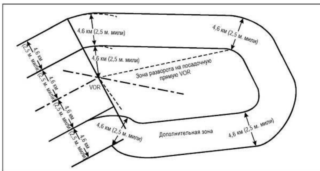
Рисунок I-4-3-Доб С-7 - Сопряжение зон начальных участков и зон разворота на посадочную прямую
