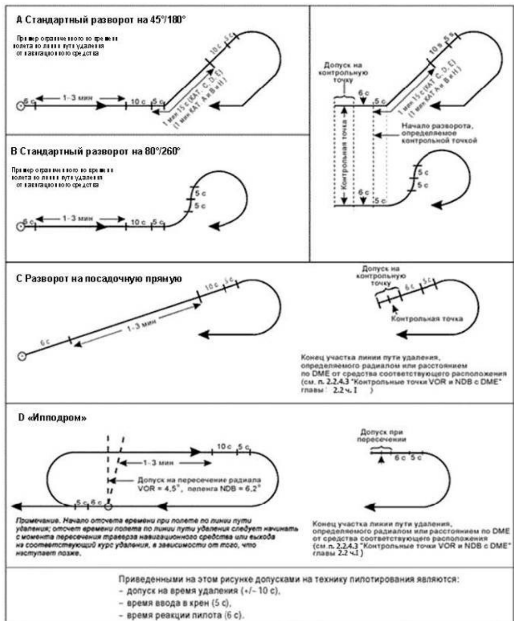
Рисунок I-4-3-8 - Применение допусков на технику пилотирования
