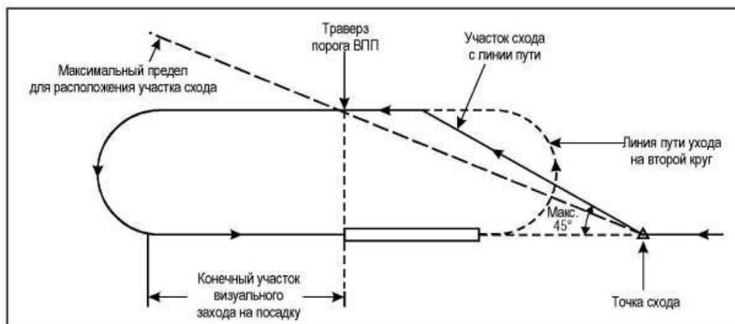
Рисунок I-4-7-Доб-2 - Общий случай стандартной линии пути
