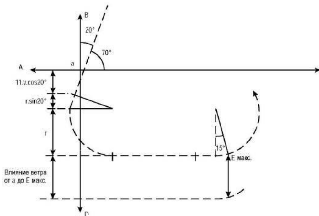
Рисунок III-3-7-Доб А-2 б) - Ожидание с применением RNAV. Расчет YE
