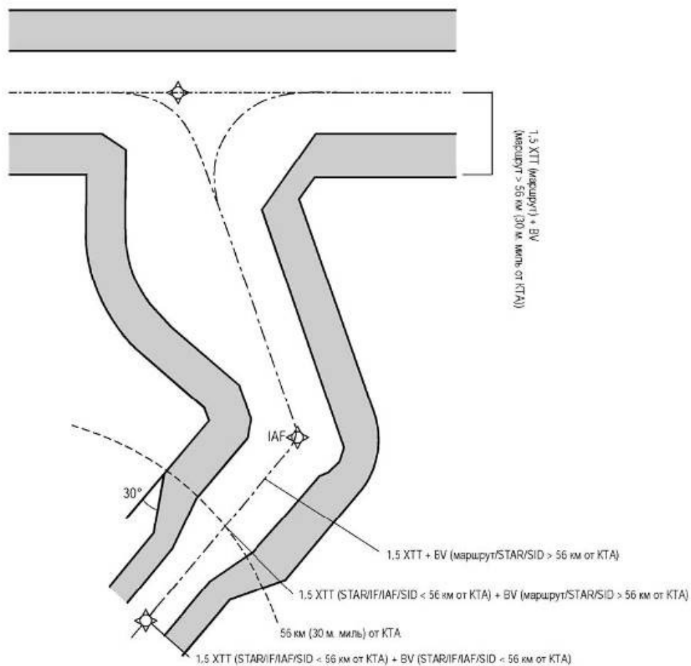
Рисунок III-3-2-1 - Прибытие. IAF находится на расстоянии, превышающем или равном 56 км (30 м. миль) от КТА
