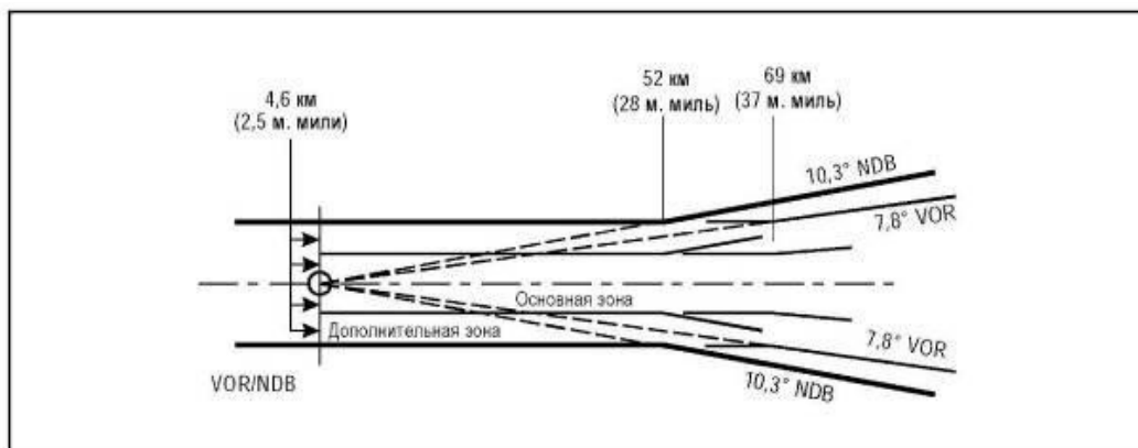
Рисунок I-4-3-3 - Зона начального этапа захода на посадку с прямолинейными линиями пути
