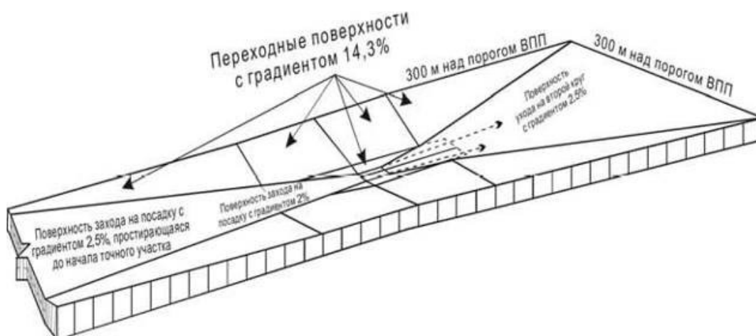
Рисунок II-1-1-6 - Основные поверхности ILS (пп. 1.1.4.7.2 гл. 1.1)
