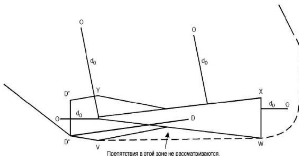
Рисунок II-1-1-Доб А-7 - Измерение расстояний d_0 до препятствий (разворот более чем на 75^\circ )
