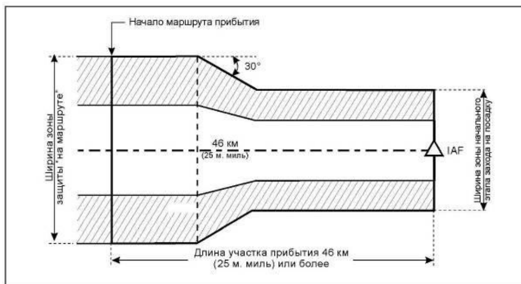
Рисунок I-4-2-1 - Участок прибытия: зона защиты (длина участка прибытия 46 км (25 м. миль) или более)
