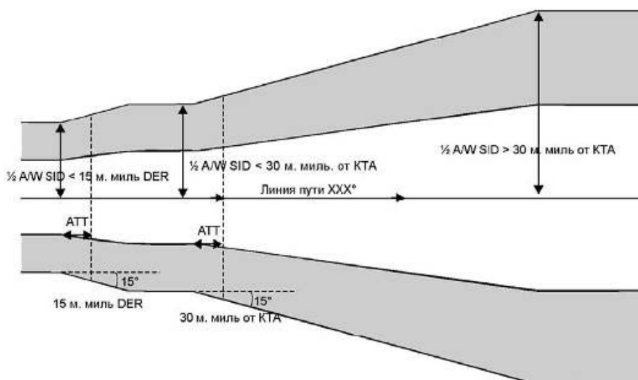
Рисунок III-1-1-2 - Слияние в точках сопряжения этапов полета: вылеты
