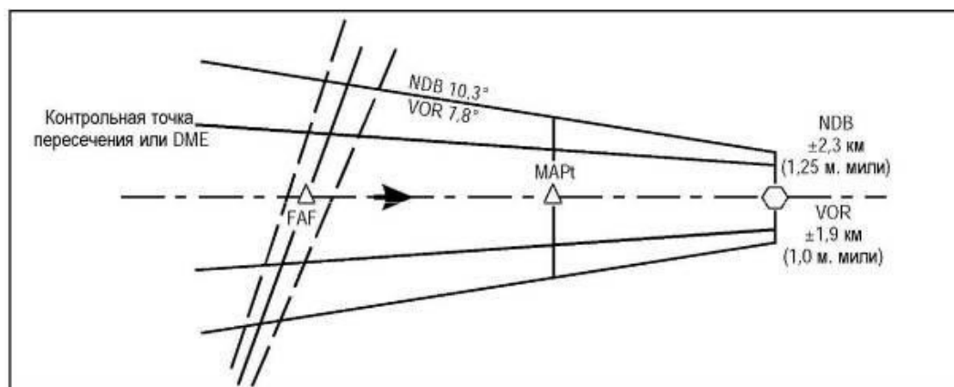
Рисунок I-4-6-9 - Пример зоны в случае продолжения использования при уходе на второй круг наведения по
