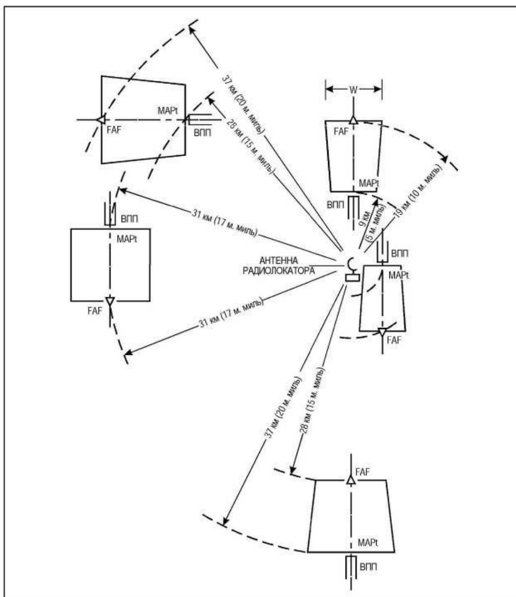
Рисунок II-2-6-2 - Примеры конечного этапа захода на посадку по обзорному радиолокатору
