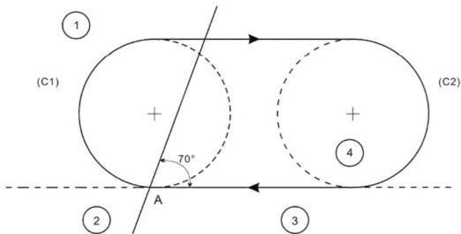
Рисунок III-3-7-Доб В-1 - Секторы входа
