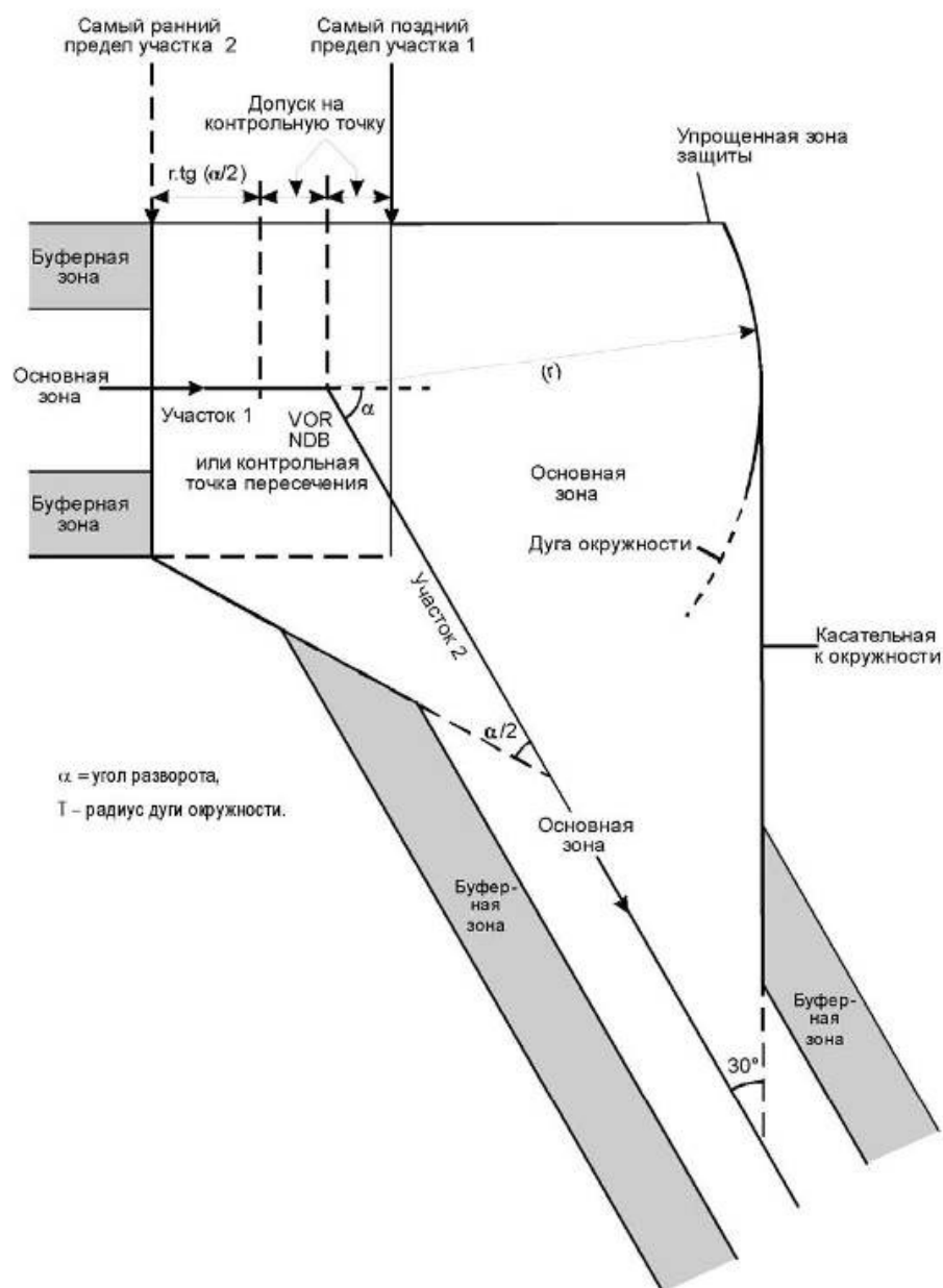
Рисунок II-3-1-5 - Разворот над навигационным средством или в контрольной точке пересечения
