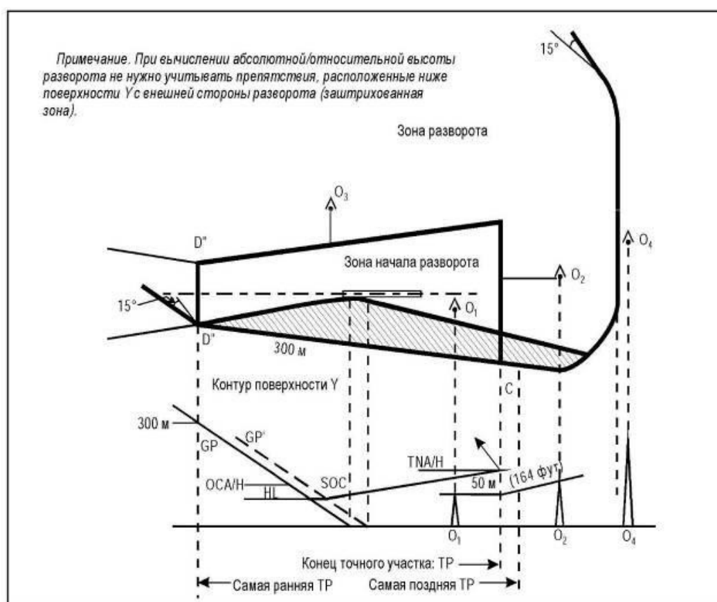
Рисунок II-1-3-18 - Разворот на заданной абсолютной высоте
