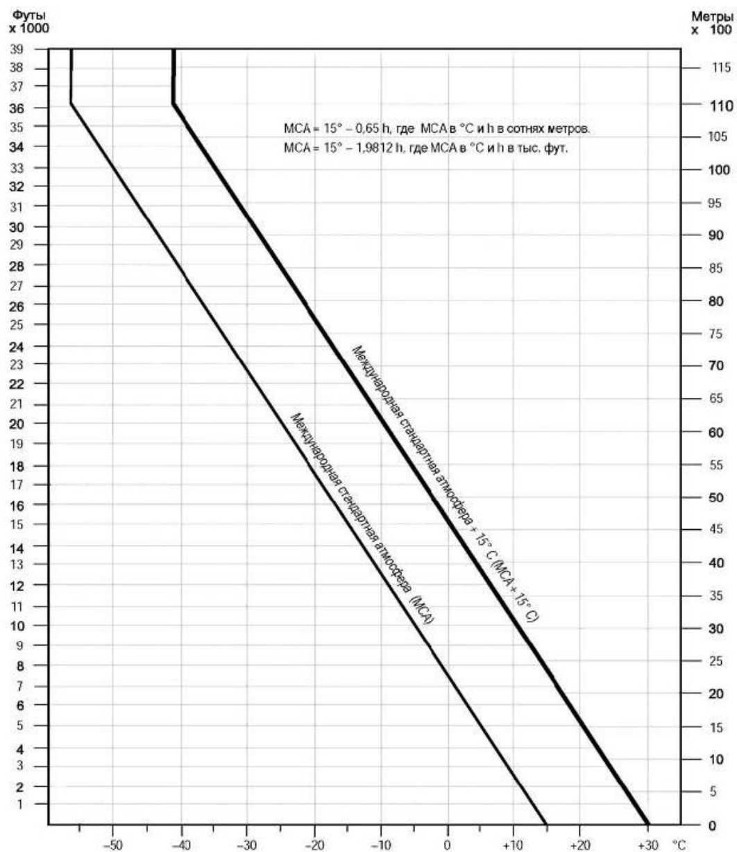
Рисунок II-4-1-Доб А-5 - Зависимость температуры от абсолютной высоты
