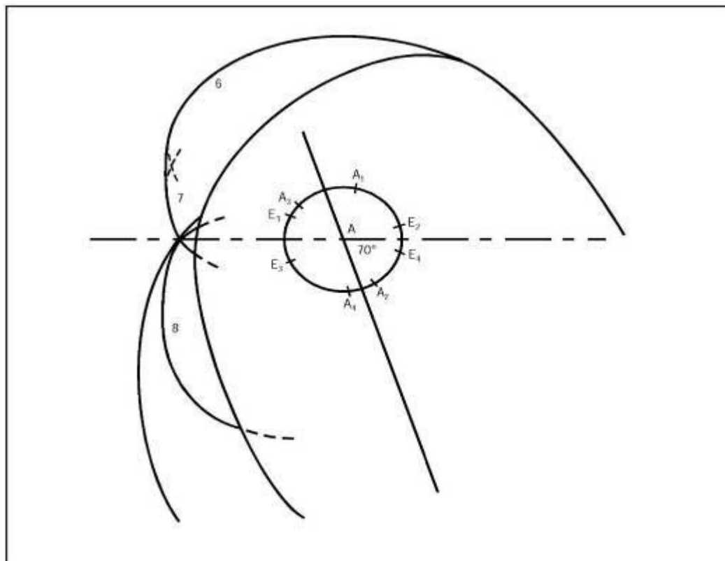
Диаграмма I-4-3-Доб С-11 - Построение зоны входа ось шаблона составляет угол 70^\circ относительно оси схемы
