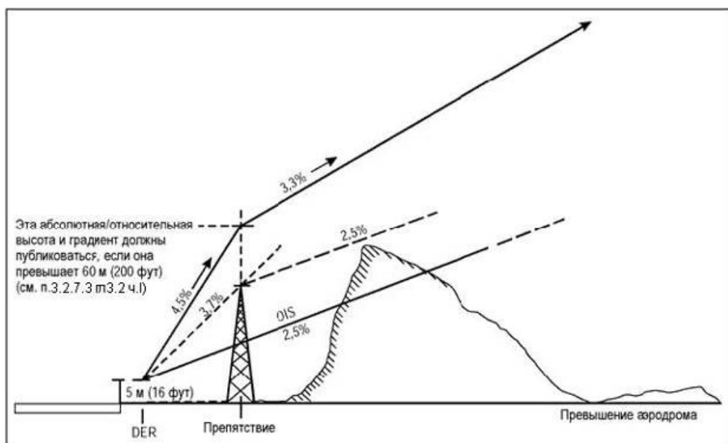
Рисунок 1-3-2-2 - Расчетный градиент схемы
