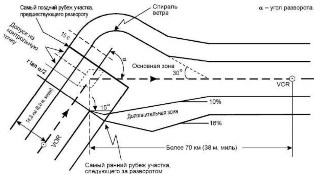
Рисунок II-3-1-Доб А-3 - Разворот над навигационным средством
