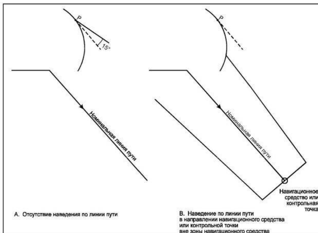
Рисунок 1-2-3-3 а) и б) - Построение внешней границы разворота после точки Р
