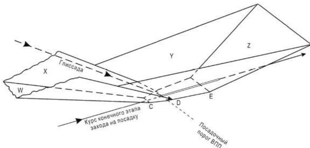
Рисунок III-3-6-8 - Иллюстрация поверхностей оценки препятствий ILS для полетов по GBAS: вид в перспективе
