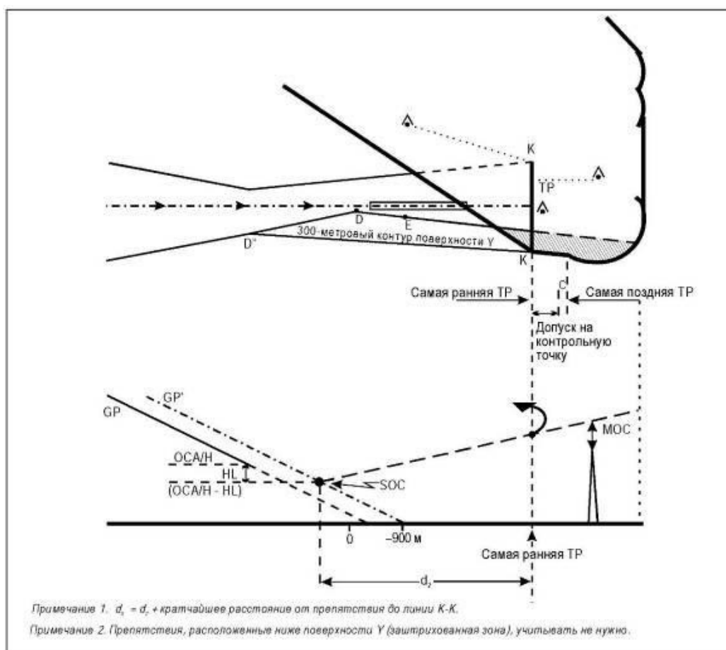
Рисунок II-1-1-18 - Разворот в заданной TR (при наличии контрольной точки TR)
