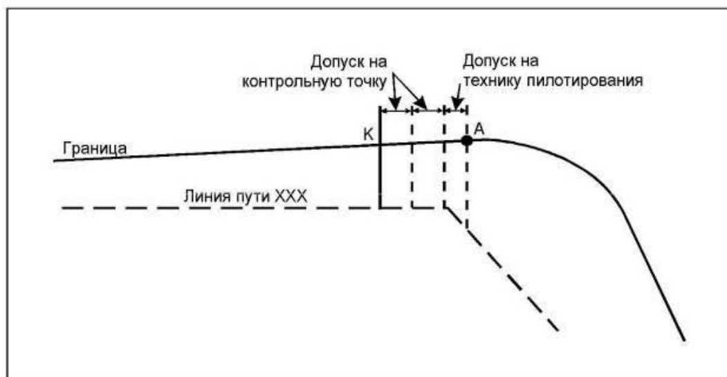
Рисунок 1-2-3-2 - Начало построения внешней границы
