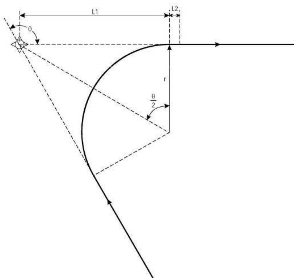
Рисунок III-2-1-8 - Минимальное расстояние стабилизации: точка пути "флай-бай"
