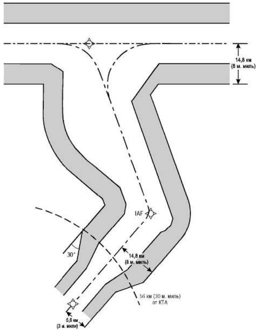
Рисунок I-4-2-5 - Критерии прибытия по GNSS, IAF за пределами 56 км (30 м. миль) от КТА
