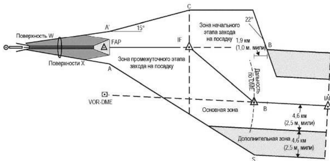
Рисунок I-4-3-Доб А-6 - Построение зон защиты зон в схеме типа S VOR/DME
