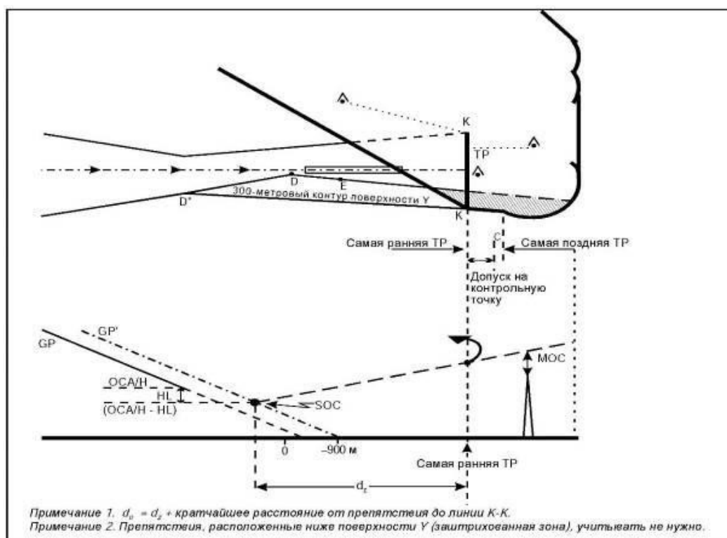
Рисунок II-1-3-19 - Разворот в заданной TP (при наличии контрольной точки TP)
