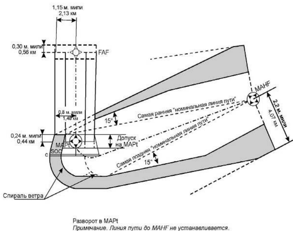
Рисунок IV-2-3 - Уход на второй круг с разворотом на угол, превышающий 90°
