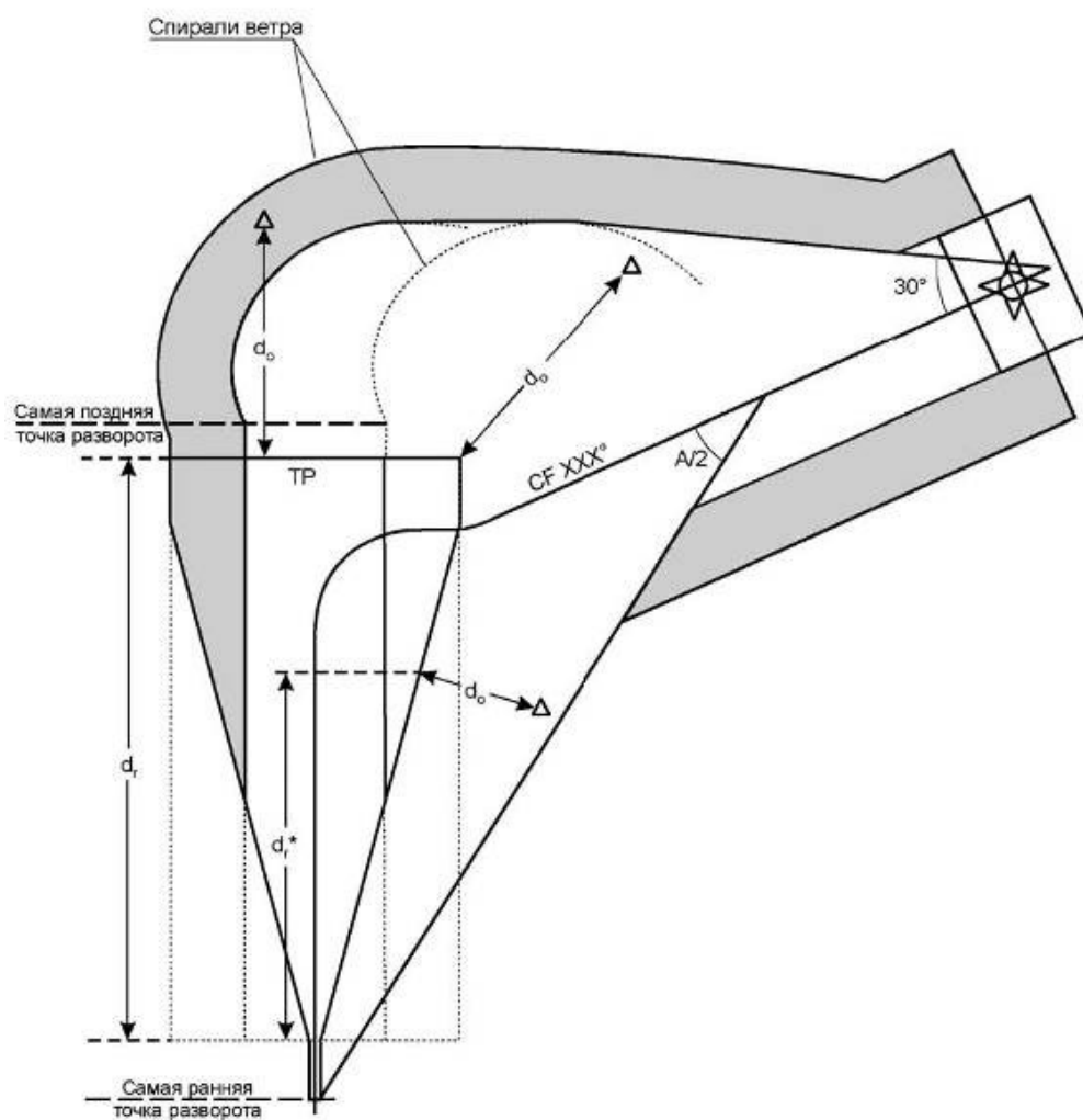
Рисунок III-2-2-8 - Разворот на абсолютной / относительной высоте, после которого следует участок CF
