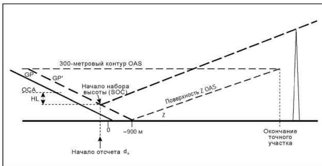
Рисунок II-1-3-17 - Запас высоты над препятствиями при уходе на второй круг по прямой
