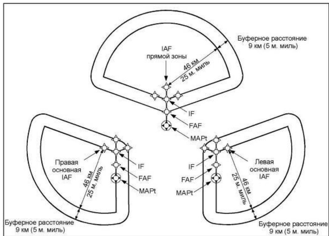
Рисунок III-2-4-1 - Y-образная конфигурация зон ТАА
