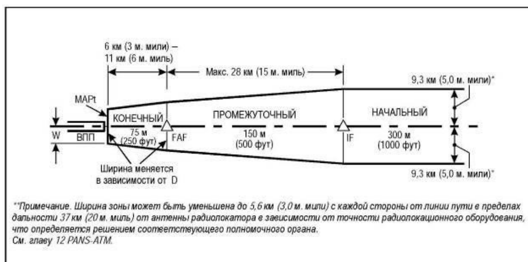
Рисунок II-2-6-1 - Участки захода на посадку по обзорному радиолокатору
