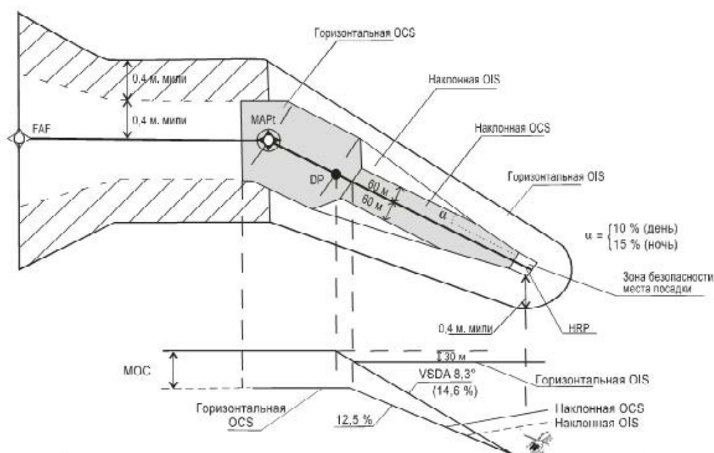
Рисунок IV-2-8 - Прямой VS с DP и с изменением курса на 30° в MAPt
