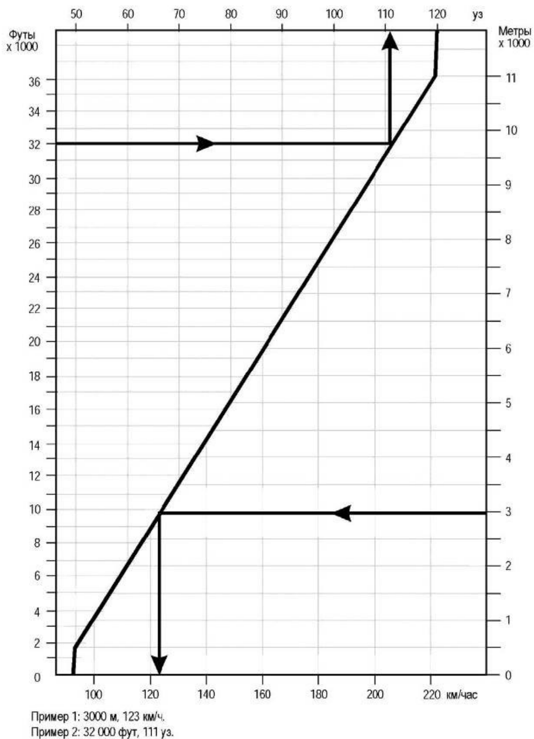
Рисунок II-4-1-Доб А-4 - Зависимость скорости учитываемого ветра от абсолютной высоты
