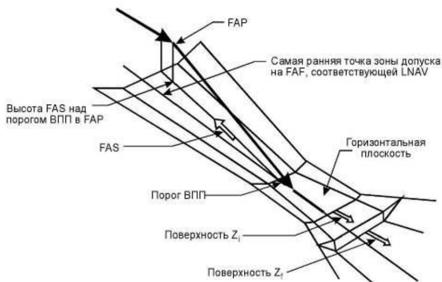
Рисунок III-3-4-3 - Изображение поверхностей APV OAS
