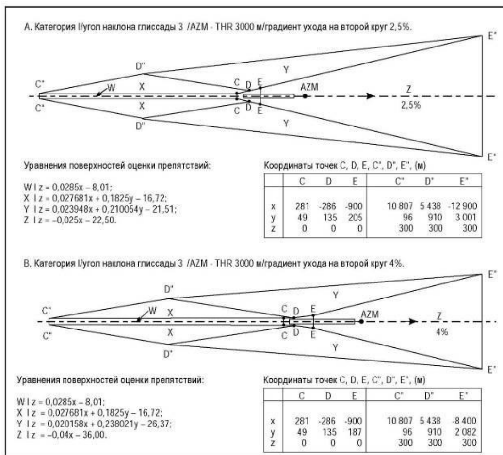
Рисунок II-1-3-12 - Типичные контуры OAS для ВС стандартных размеров
