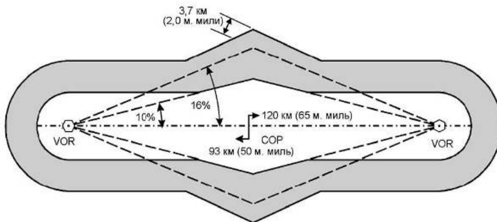
Рисунок II-3-1-7 - Смещенная точка переключения. Пример с двумя VOR
