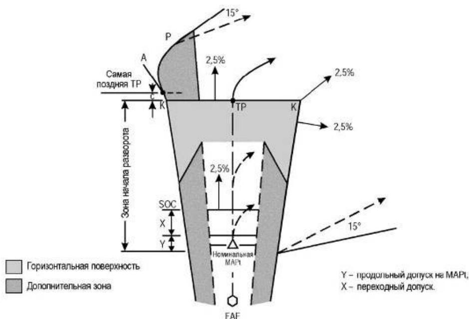
Рисунок I-4-6-11 - Разворот на абсолютной высоте менее чем на 75°
