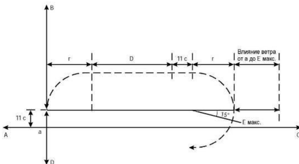
Рисунок III-3-7-Доб А-2 а) - Ожидание с применением RNAV. Расчет XE
