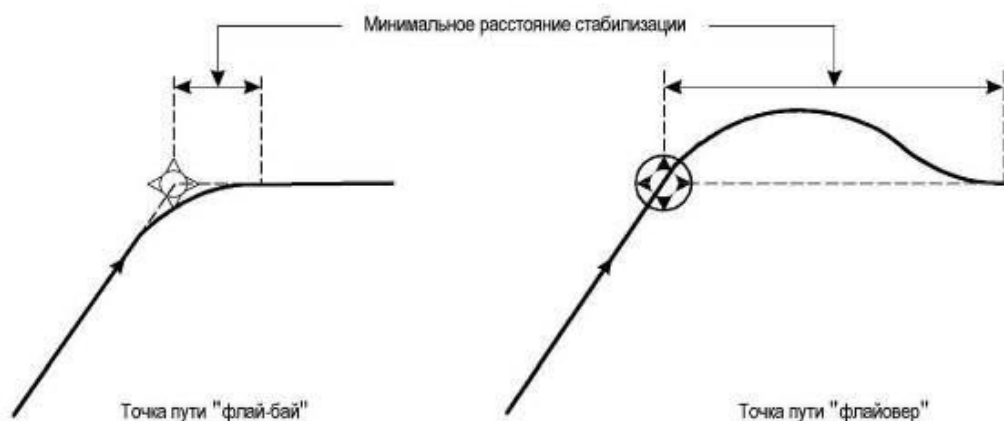
Рисунок III-2-1-1 - Определение минимального расстояния стабилизации
