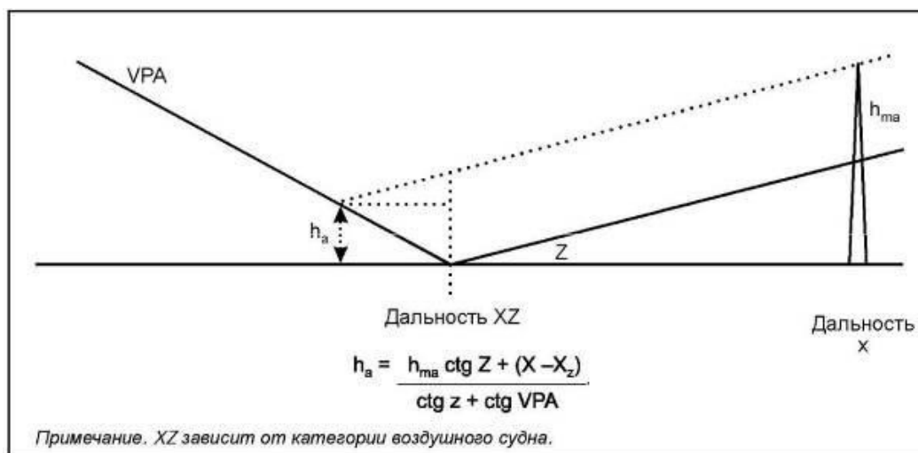
Рисунок III-3-4-80020 - Расчет h_a по h_{ma}
