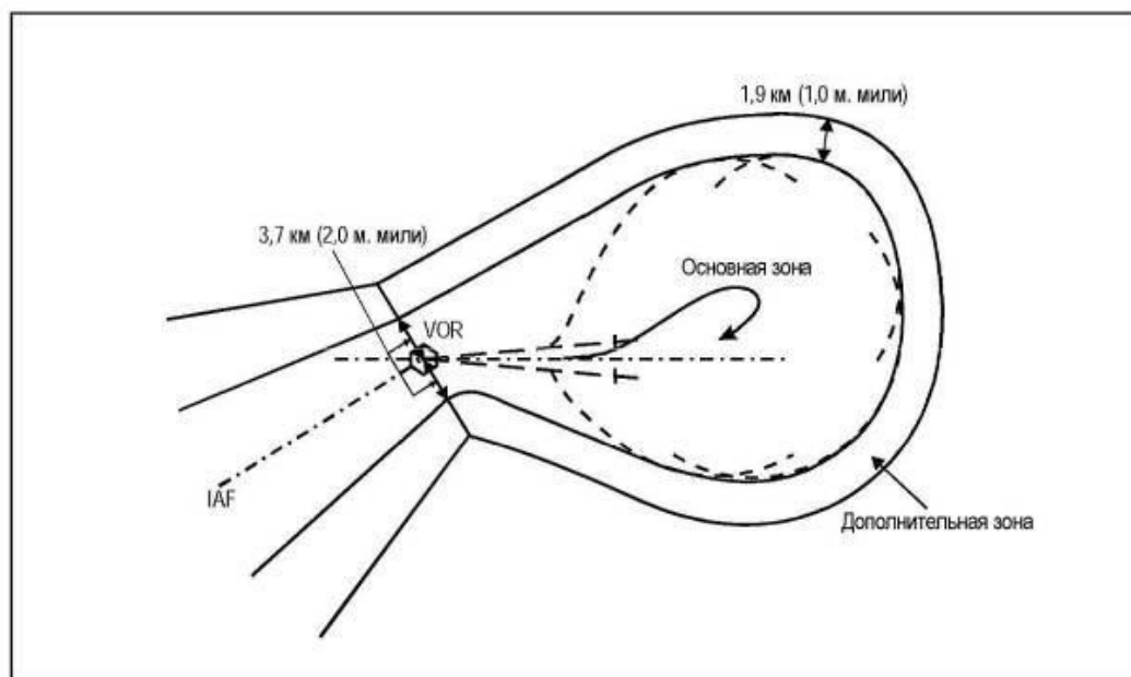
Рисунок I-4-3-Доб В-6 - Сопряжение основной и дополнительных зон начального участка захода на посадку и обратной схемы (пример с VOR)
