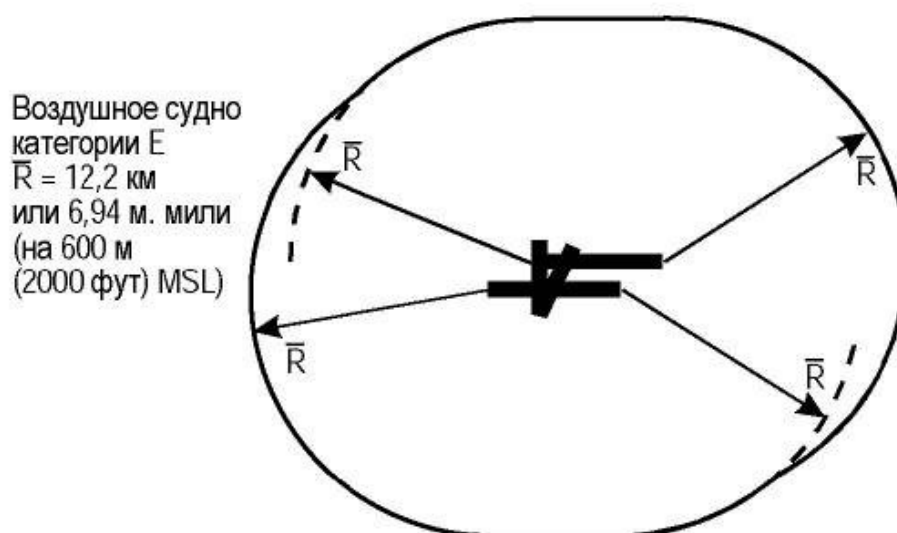
Рисунок I-4-7-1 - Построение зоны визуального маневрирования (полета по кругу)
