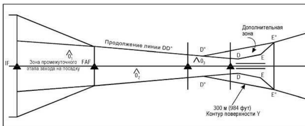
Рисунок II-2-2-1 - Схема только для азимутального оборудования. Зоны
