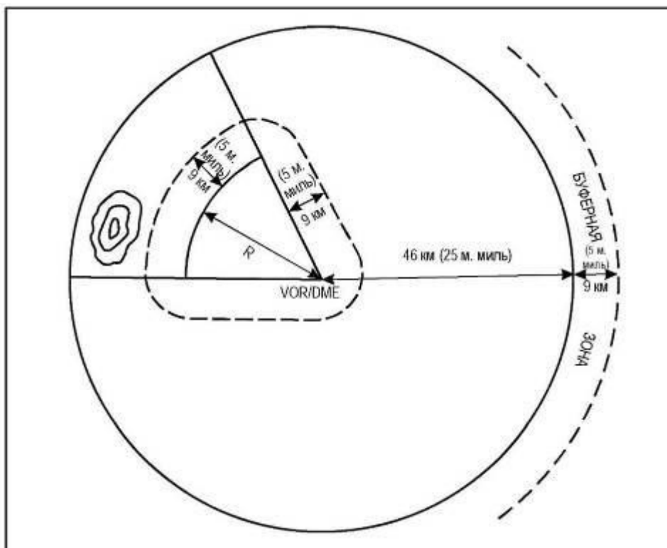
Рисунок I-4-8-2 - Вариант подсекторов VOR/DME, границы которых определяются дугой DME
