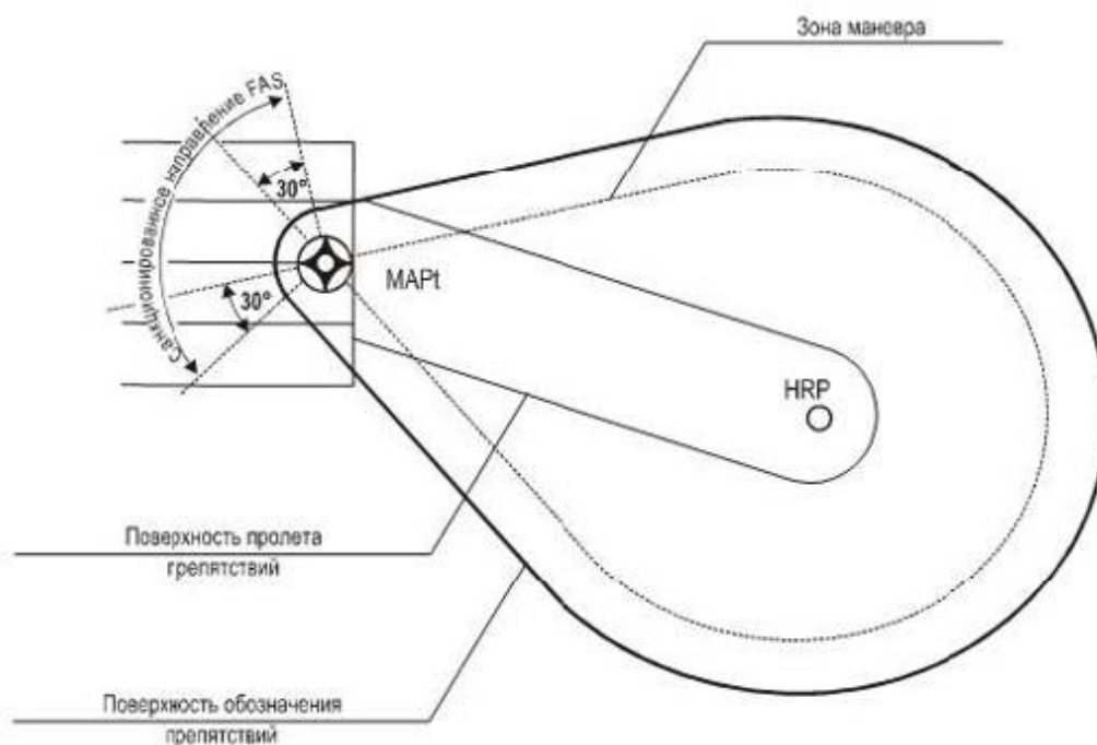
Рисунок IV-2-15 - Представление горизонтальной OIS и горизонтальной OCS с учетом поверхности захода на посадку с любых направлений
