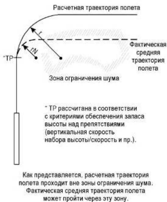
Рисунок I-3-3-Доб-3 - Разворот в заданной ТР. Схема без применения статистических данных
