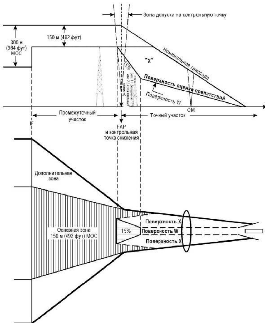
Рисунок II-1-1-2 - Конечная контрольная точка захода на посадку, определяемая контрольной точкой снижения, расположенной в точке конечного этапа захода на посадку
