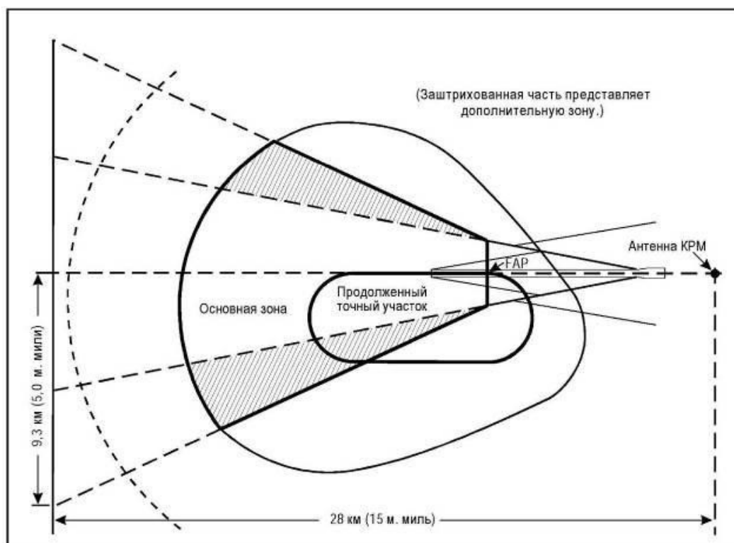
Рисунок II-1-1-4 - Зона промежуточного этапа захода на посадку. Заход на посадку по ILS с использованием обратной схемы или схемы "ипподром"
