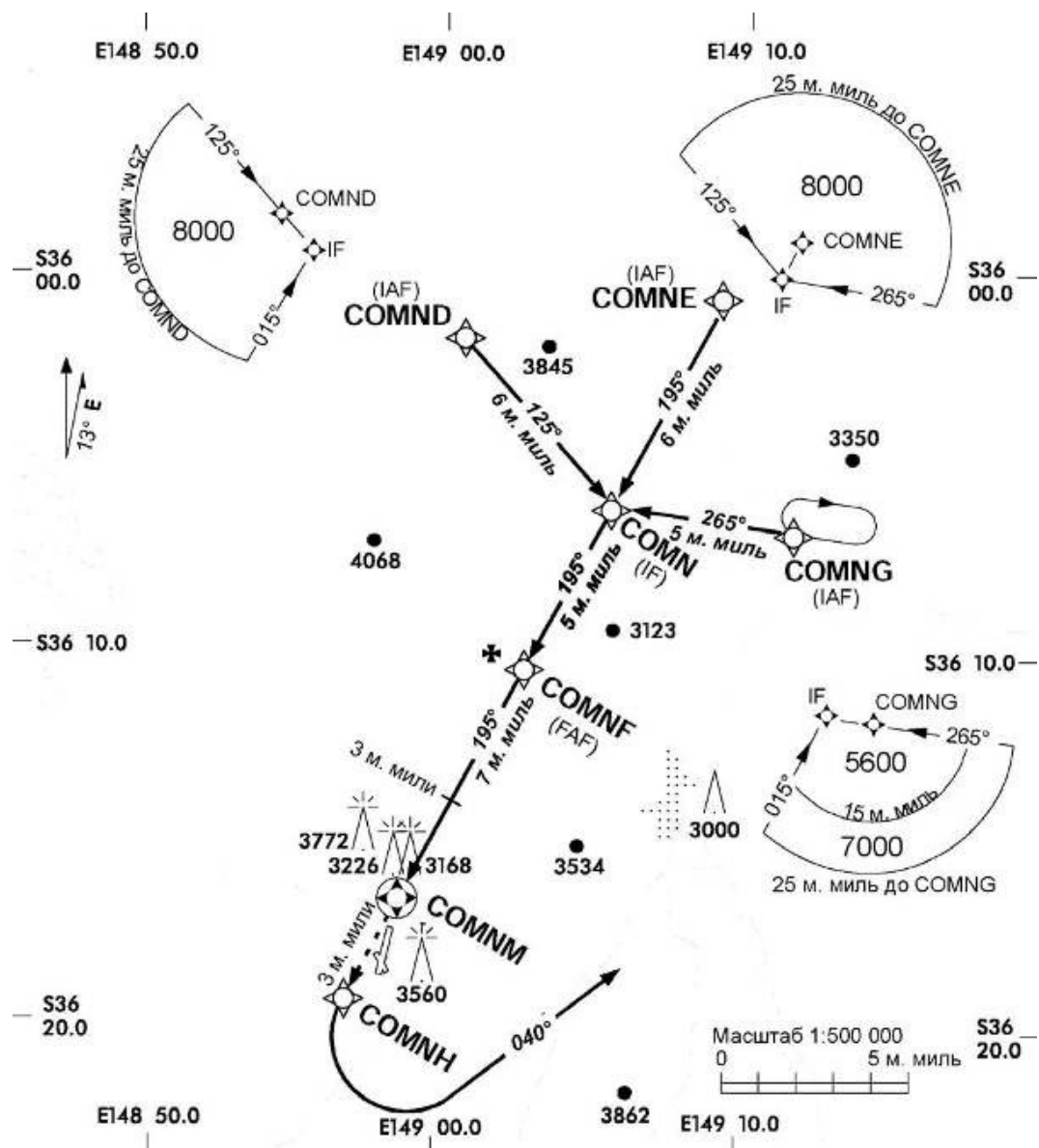
Рисунок III-2-4-3 - Пиктограммы Y-образного расположения ТАА
