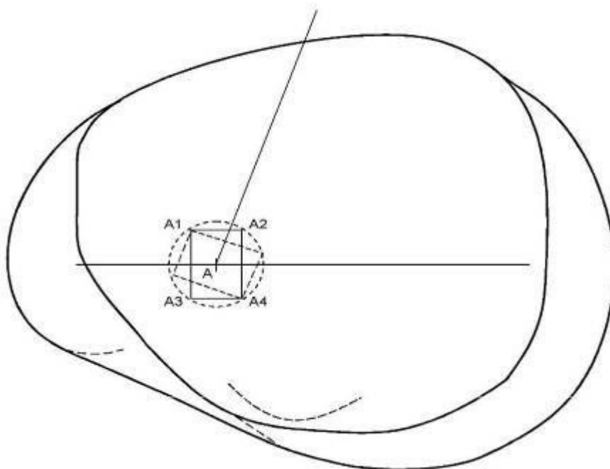
Рисунок III-3-7-Доб А-8 - Зона ожидания RNAV, включая защиту схем входа для системы RNAV без функции ожидания. Участок удаления определяется по времени
