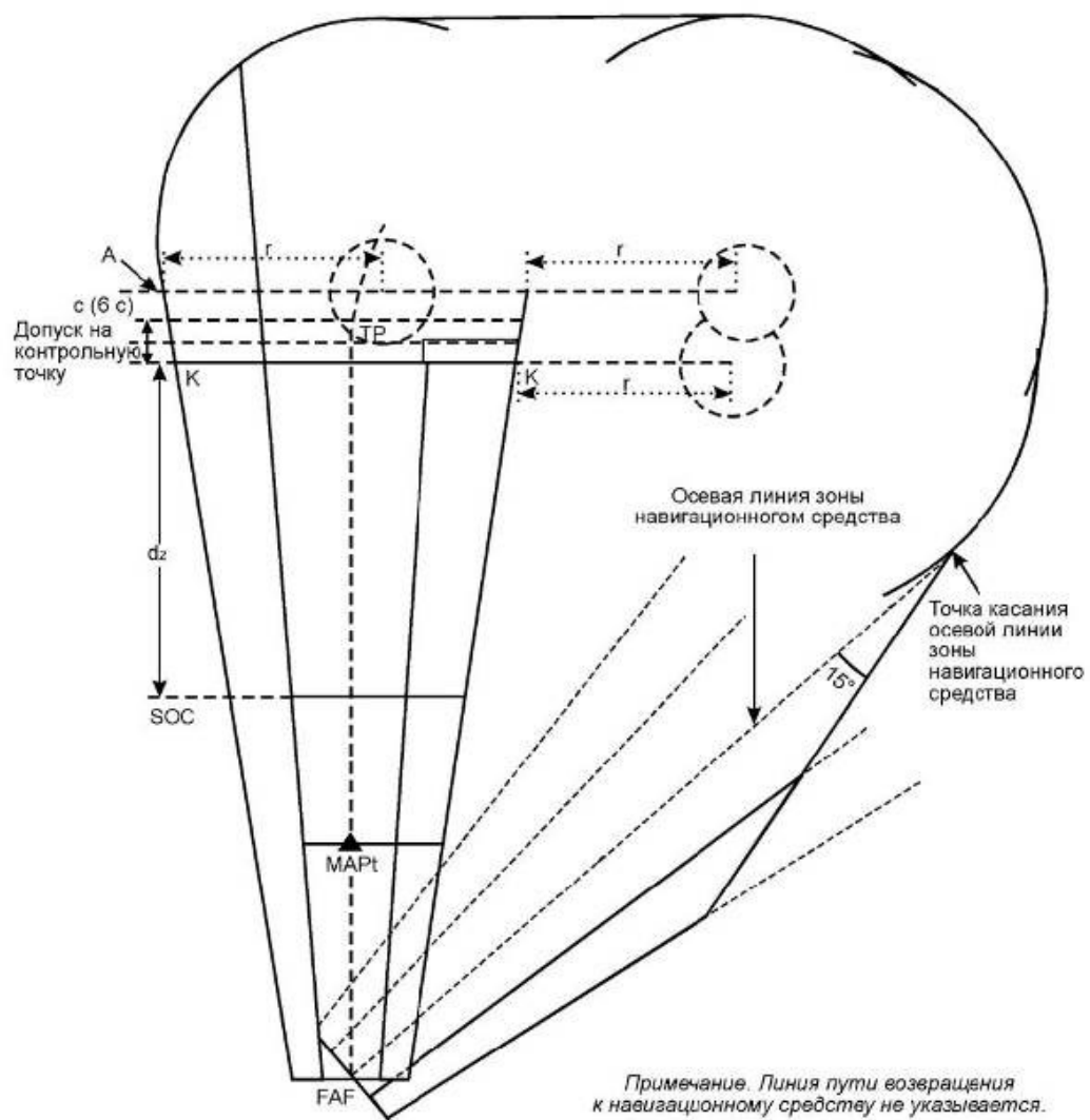
Рисунок I-4-6-18 - Уход на второй круг с разворотом с контрольной точкой TP и возвращением к FAF без линии пути возвращения
