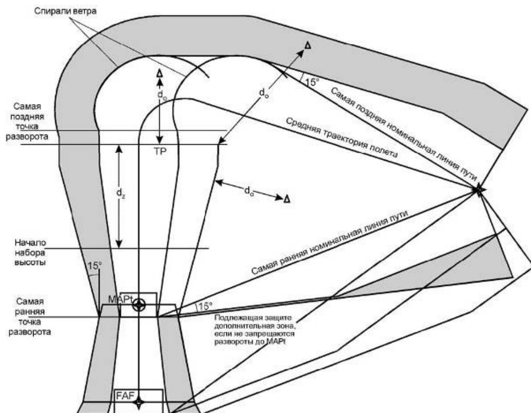
Рисунок III-2-2-10 - Разворот на абсолютной / относительной высоте при уходе на второй круг, после которого следует участок DF
