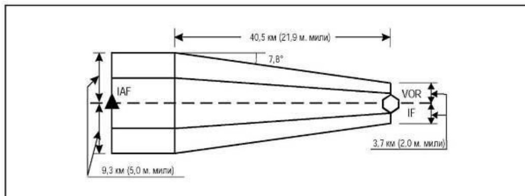
Рисунок I-4-3-Доб В-1 - Случай, когда IAF находится на расстоянии более 40, 5 км (21,9 м. мили) от VOR
