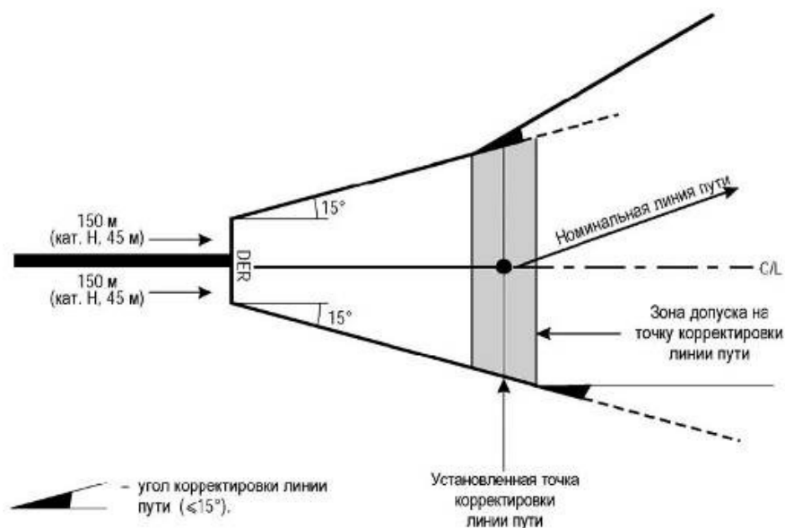
Рисунок I-3-3-3 - Зона вылета по прямой с установленной первой точкой корректировки линии пути
