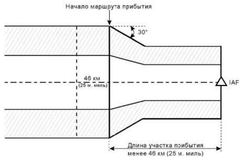
Рисунок I-4-2-2 - Участок прибытия: зона защиты (длина участка прибытия менее 46 км (25 м. миль))
