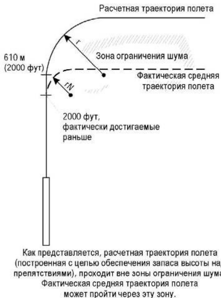
Рисунок I-3-3-Доб-1 - Разворот на заданной абсолютной высоте разворота. Схема без применения статистических данных
