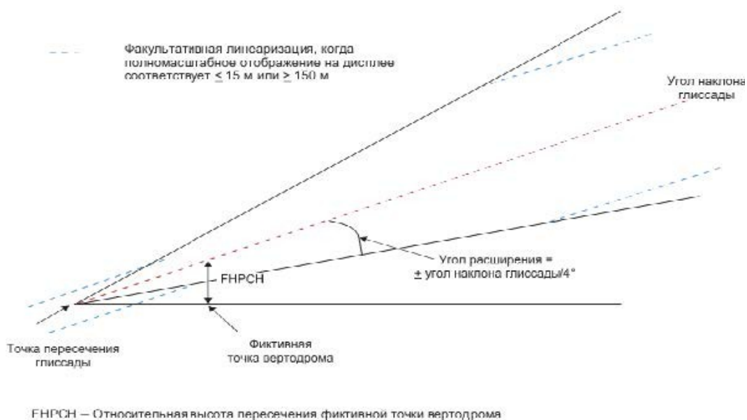
Рисунок IV-3-Доб-А-2 - Ориентация фиктивной точки вертодрома и масштабирование изображения на дисплее по вертикали
