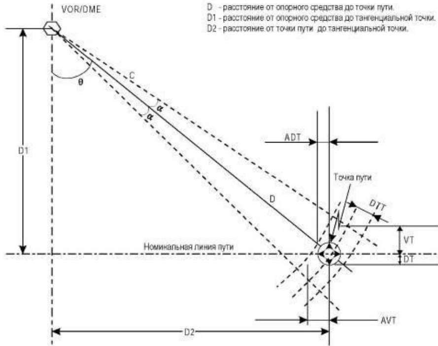
Рисунок III-1-4-2 - Вычисление допусков на точки пути
