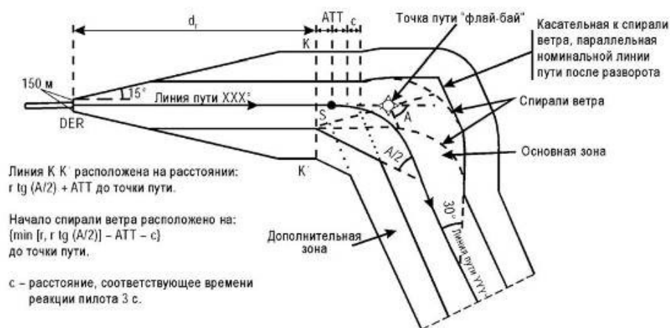
Рисунок III-3-1-3 - Разворот в точке пути "флай-бай"
