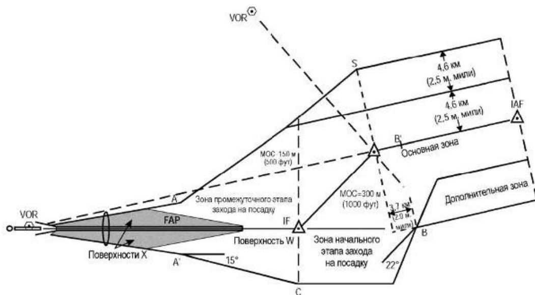
Рис. I-4-3-Доб А-5 - Построение зон защиты в схеме типа S VOR/VOR
