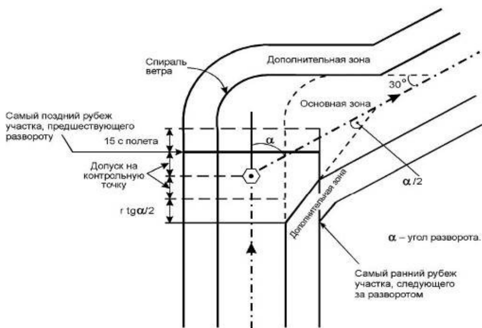
Рисунок II-3-1-Доб А-3 - Разворот над навигационным средством
