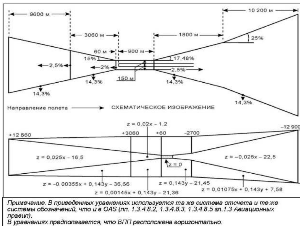
Рисунок II-1-3-8 - Уравнения поверхностей: основные поверхности ILS
