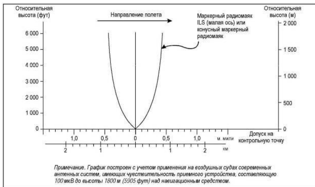
Рисунок I-2-2-2 - Зона действия маркерного радиомаяка ILS или конусного маркерного радиомаяка
