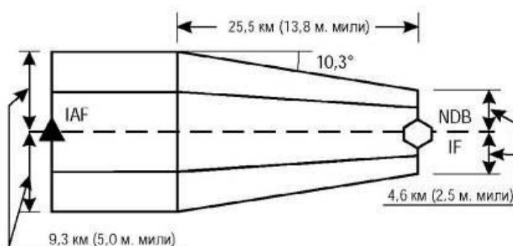
Рисунок I-4-3-Доб В-3 - Случай, когда IAF находится на расстоянии более 25,5 км (13,8 м. мили) от NDB
