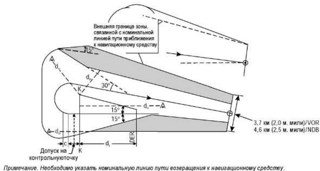
Рисунок I-3-3-12 - Вылет с разворотом. Разворот на угол более 90°
