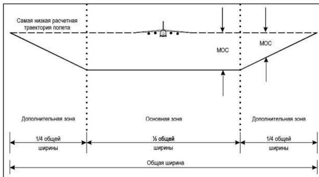
Рисунок 1-2-1-1 - Поперечное сечение зоны прямолинейного участка, включающей основную и дополнительную зоны
