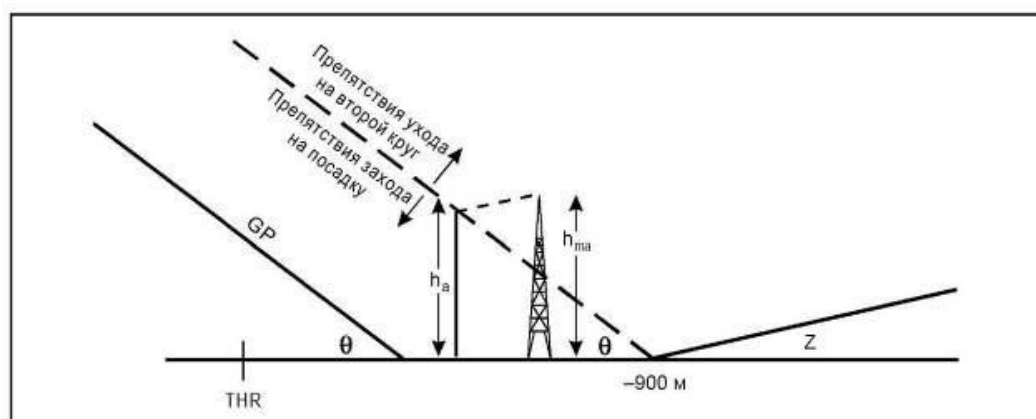
Рисунок II-1-3-15 - Препятствие ухода на второй круг, расположенное до дальности - 900 м
