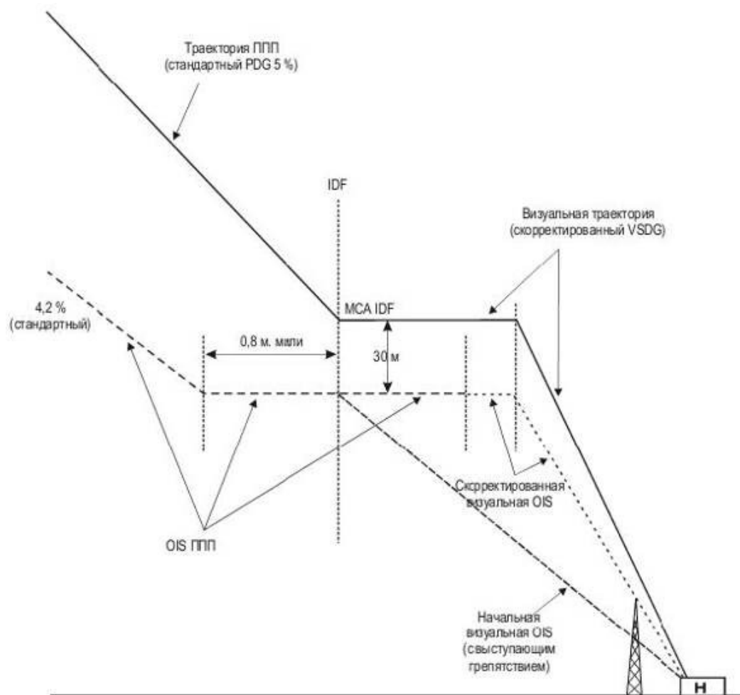
Рисунок IV-1-3 - Компенсация возвышения препятствия над OIS путем увеличения VSDG
