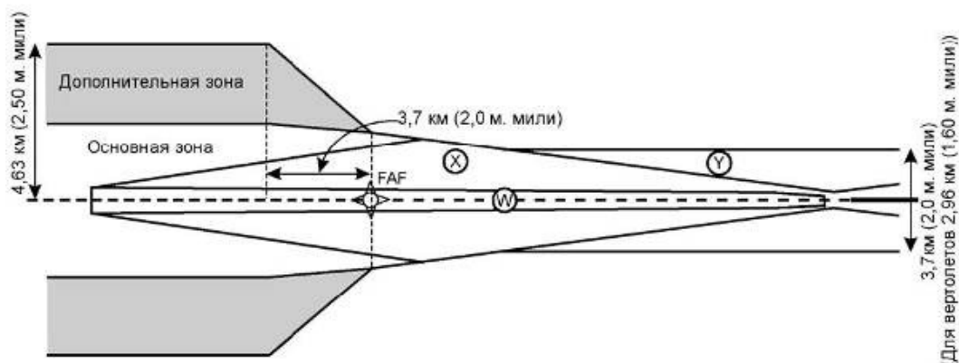
Рисунок III-3-5-1a) - Зона промежуточного участка захода на посадку (полностью основанная на SBAS). FAF дальше от порога ВПП (ширина поверхности X в FAF больше чем 3,7 км (2 м. мили))
