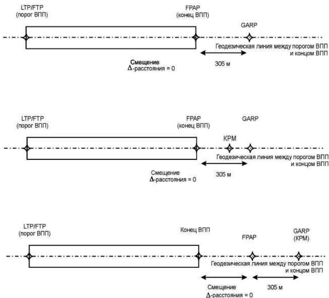
Рисунок III-2-6-1 - Местоположение FPAP (отсутствие ILS для захода на посадку)
