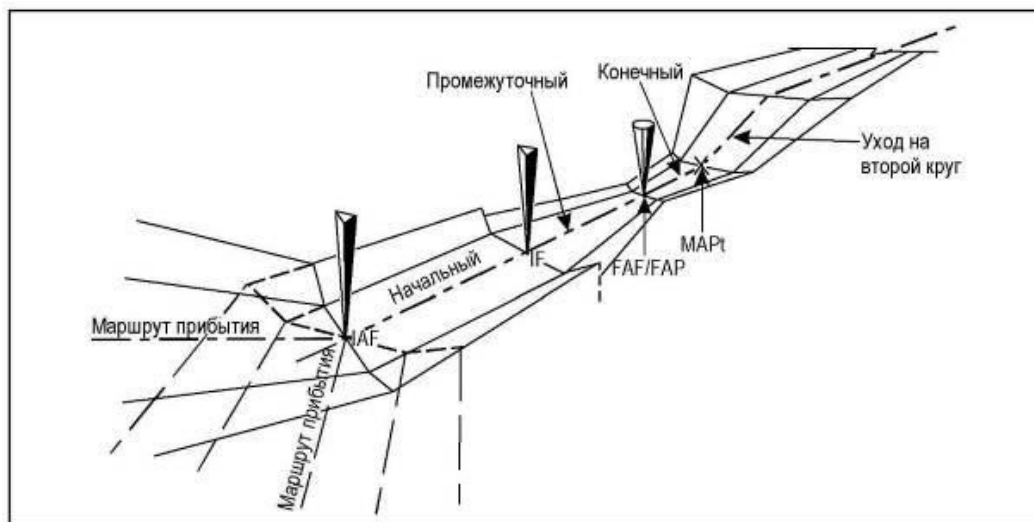
Рисунок I-4-1-1 - Участки схемы захода на посадку по приборам
