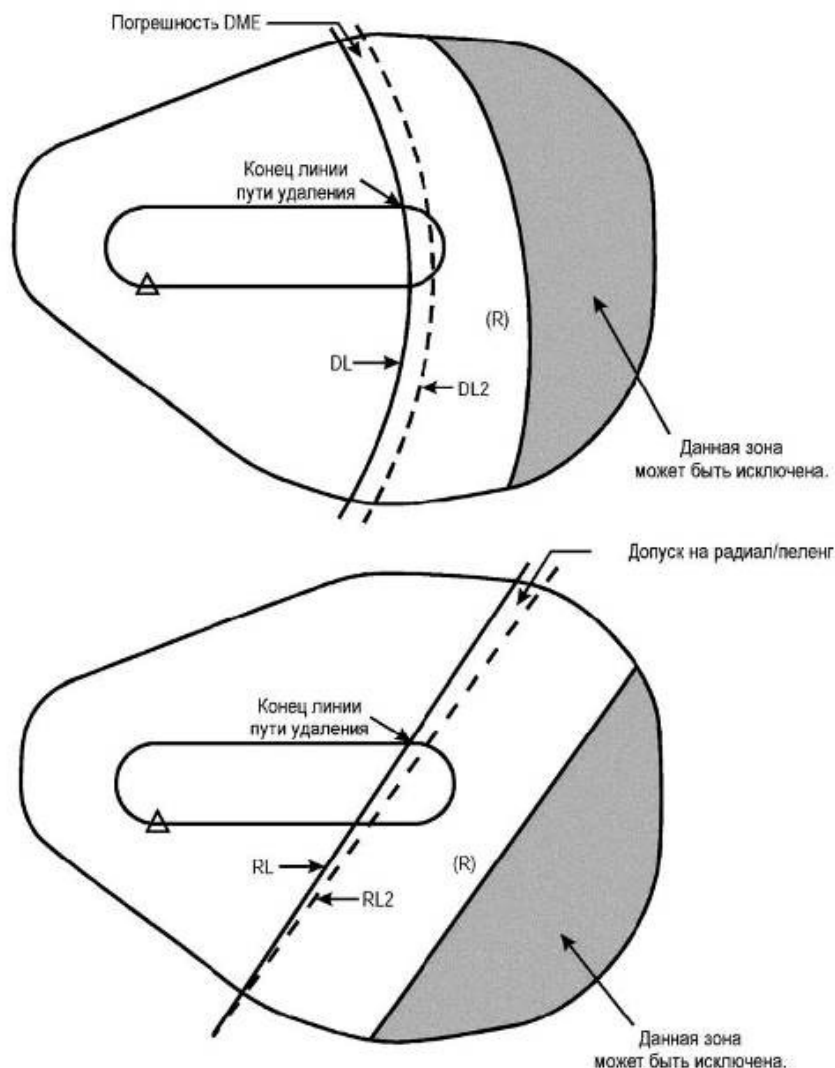
Рисунок I-4-3-Доб С-15 - Пример уменьшения зоны с помощью DME или радиала или пеленга пересечения
