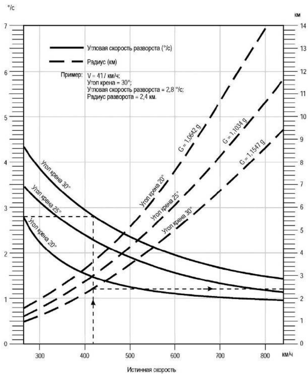
Рисунок II-4-1-Доб А-1 - Угол крена, угловая скорость разворота, радиус разворота и величины g при измерении скорости (в единицах СИ)
