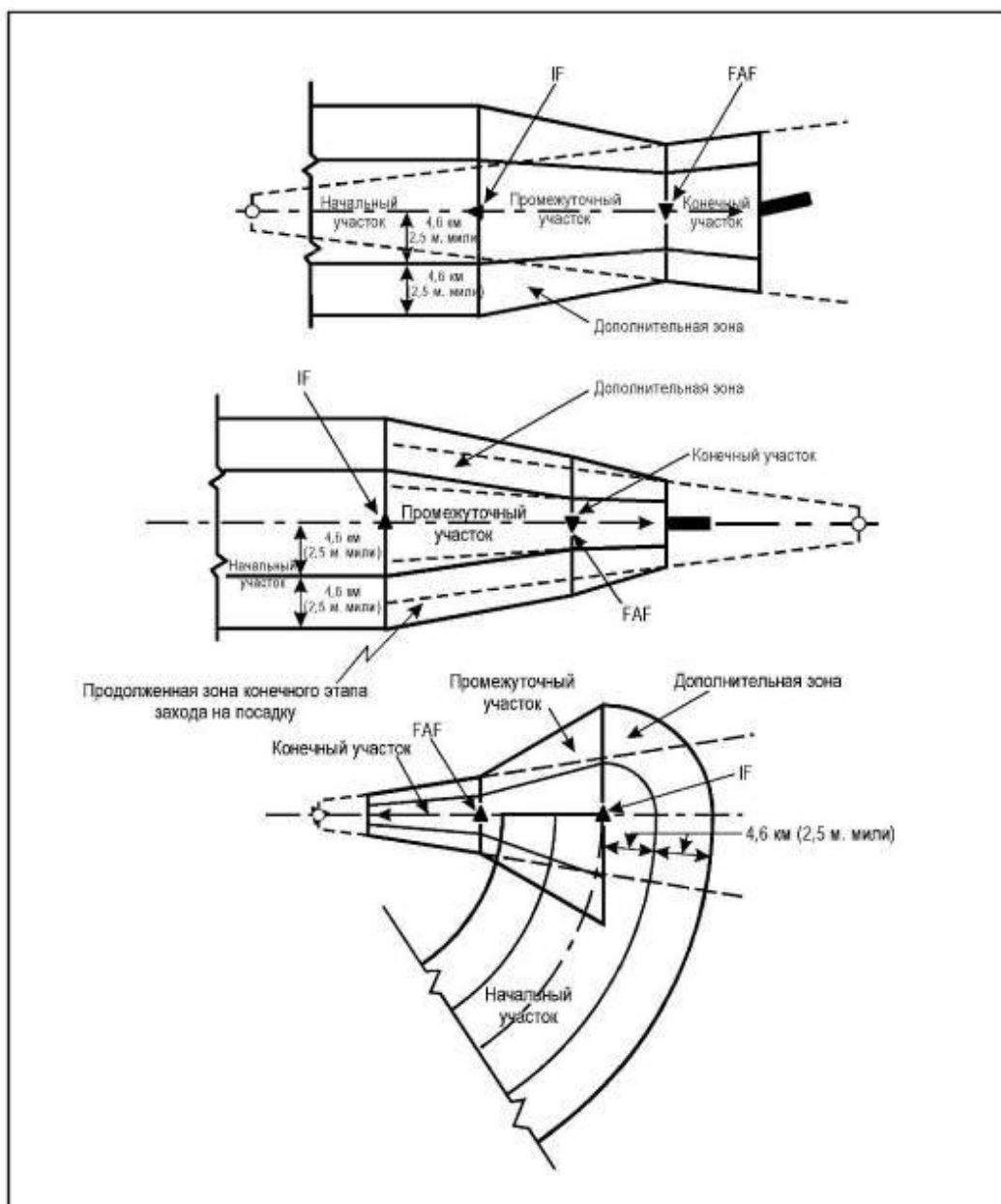
Рисунок I-4-3-2 - Типичные участки (вид сверху)
