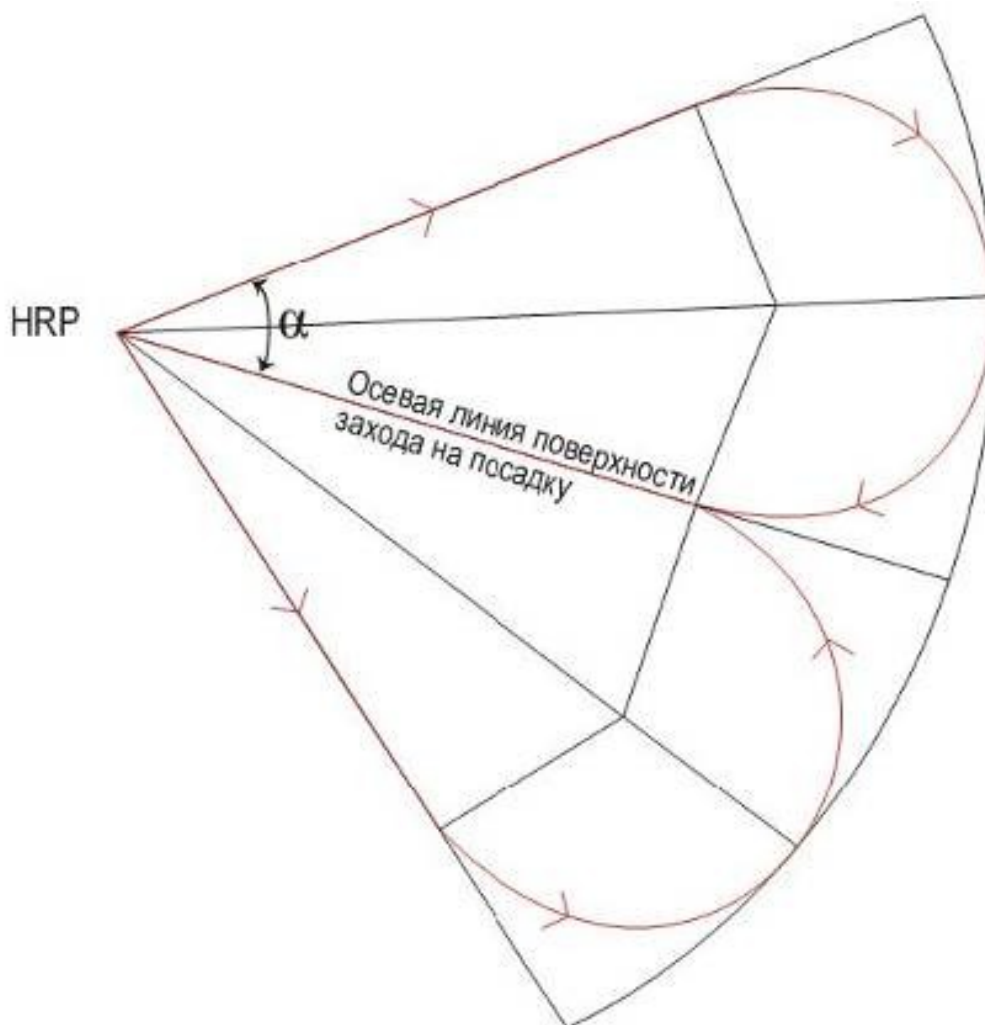
Рисунок IV-2-12 - "Зона разворота на посадочную прямую"
