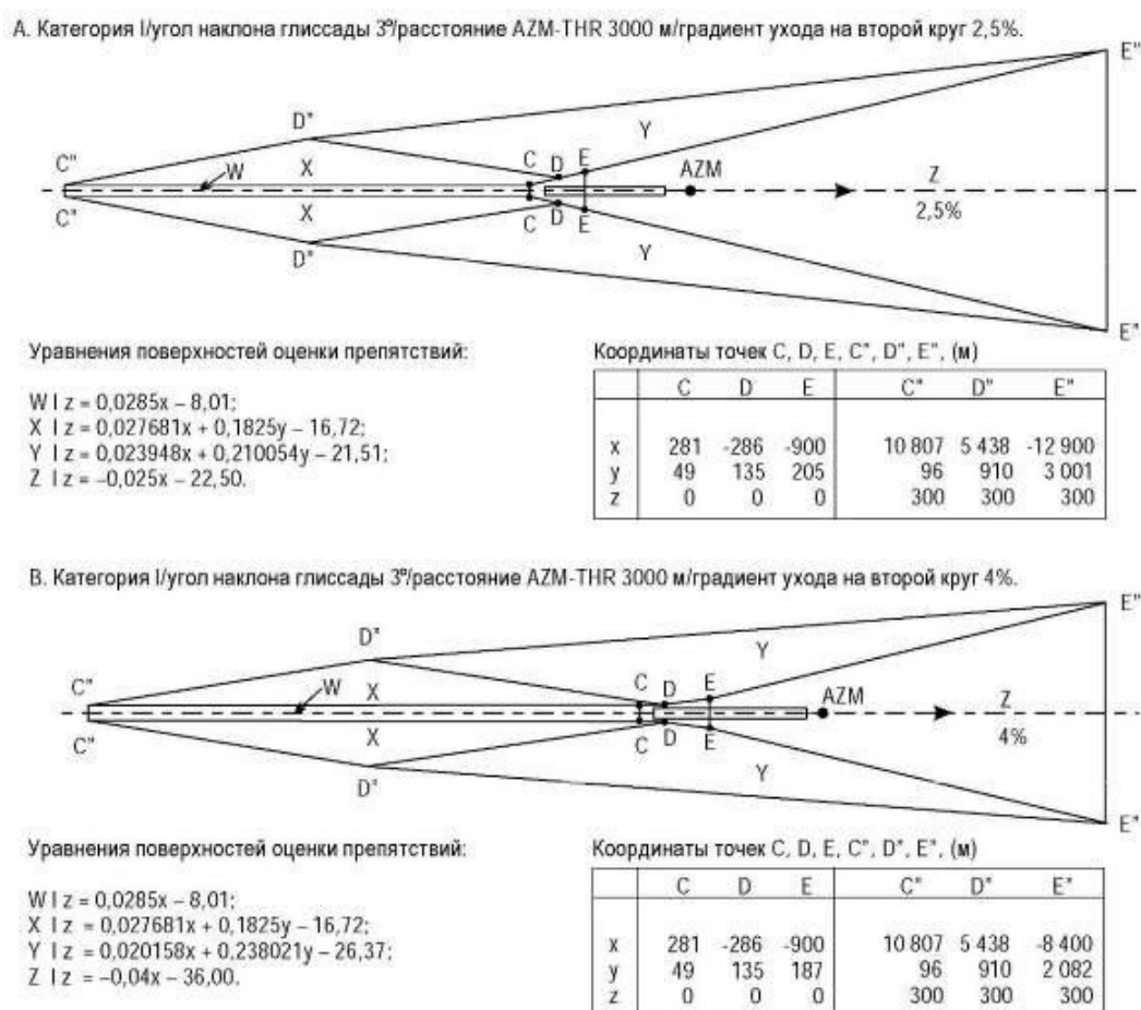
Рисунок III-3-6-10 - Типичные контуры OAS для воздушных судов стандартных размеров
