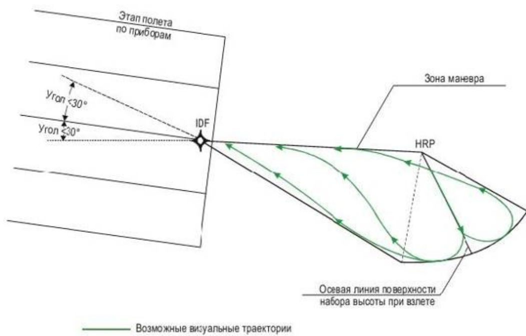
Рисунок IV-1-5 - Представление возможных траекторий на визуальном участке маневрирования, определяющих "зону маневрирования" для заданной осевой линии поверхности набора высоты при взлете
