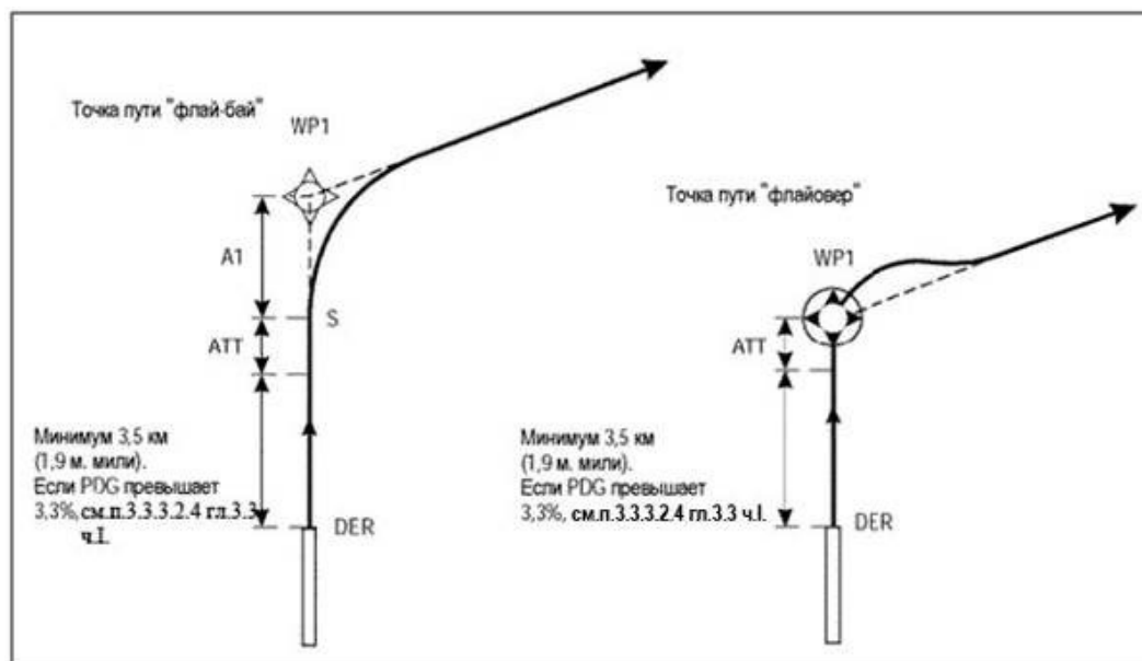
Рисунок III-2-1-6 - Минимальное расстояние стабилизации. DER - первая точка пути
