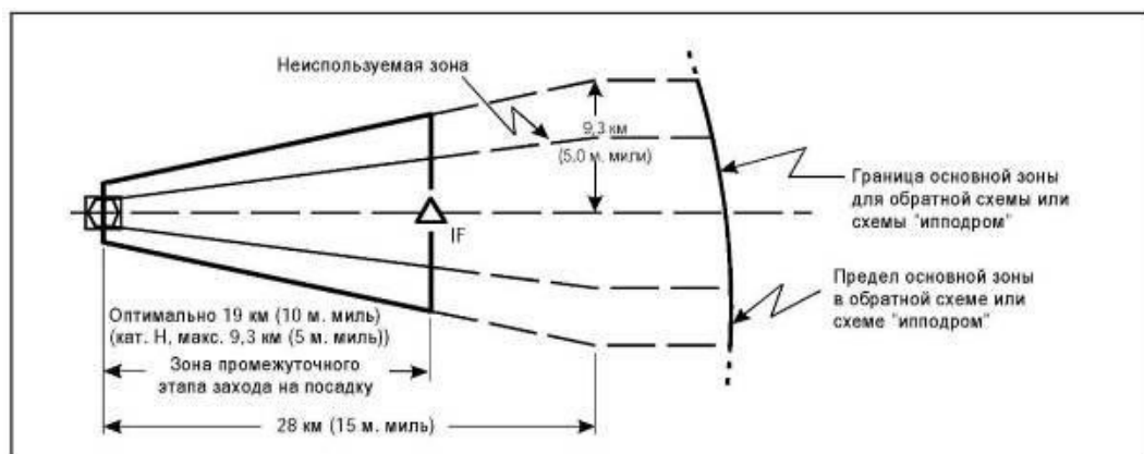
Рисунок I-4-4-1 - Зона промежуточного этапа захода на посадку в пределах обратной схемы или схемы "ипподром" при наличии контрольной точки
