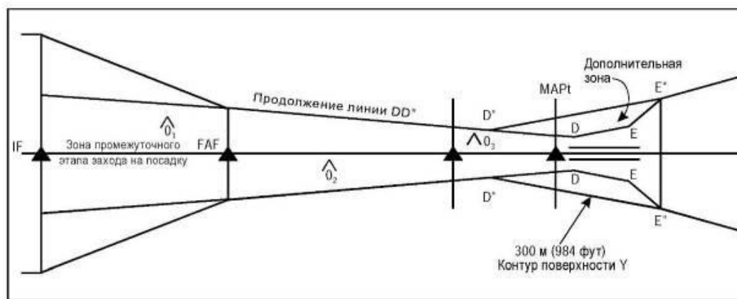
Рисунок II-2-1-1 - Схема только для курсового радиомаяка. Зоны
