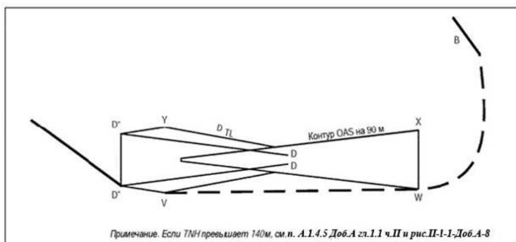
Рисунок II-1-1-Доб А-4 - Зона разворота (TNH = 90 м)
