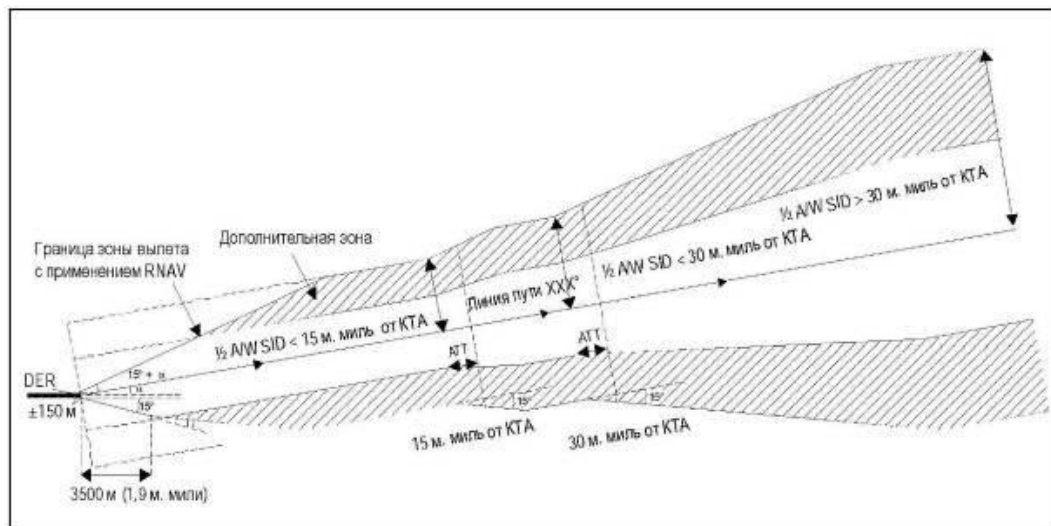
Рисунок III-3-1-1 - Вылет по прямой
