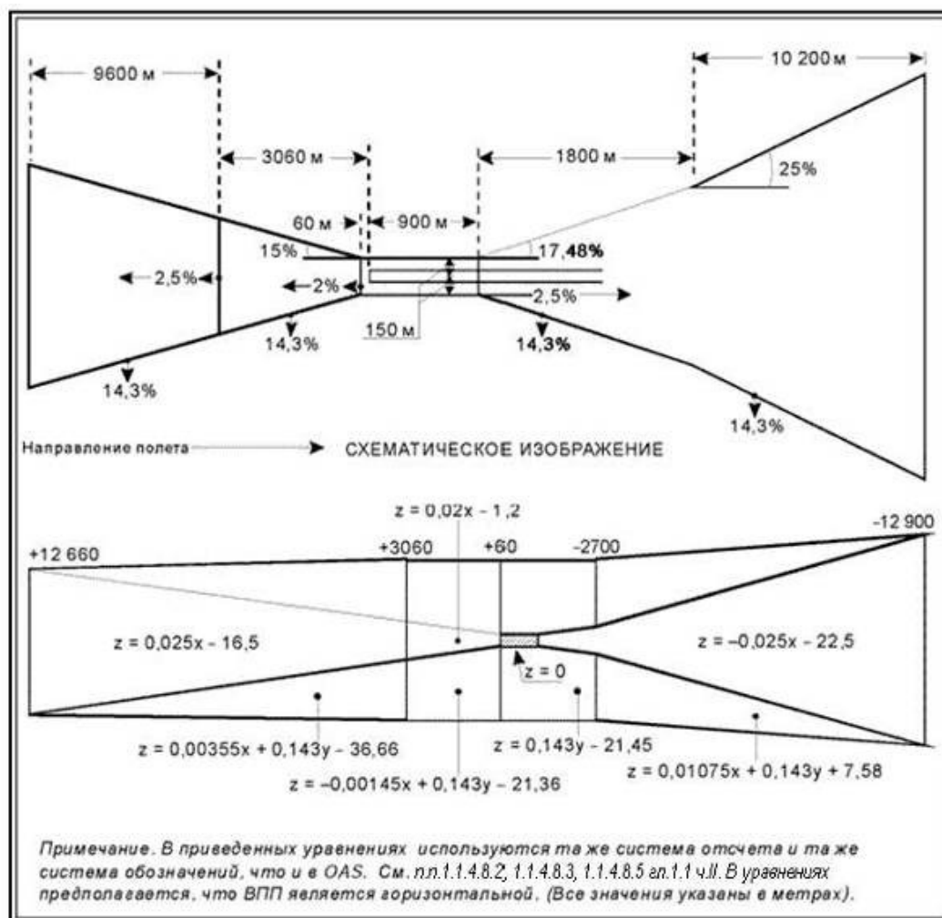
Рисунок II-1-1-7 - Уравнения поверхностей. Основные поверхности ILS
