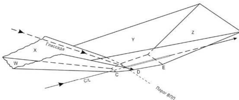
Рисунок II-1-3-10 - Поверхности оценки препятствий ILS. Вид в перспективе
