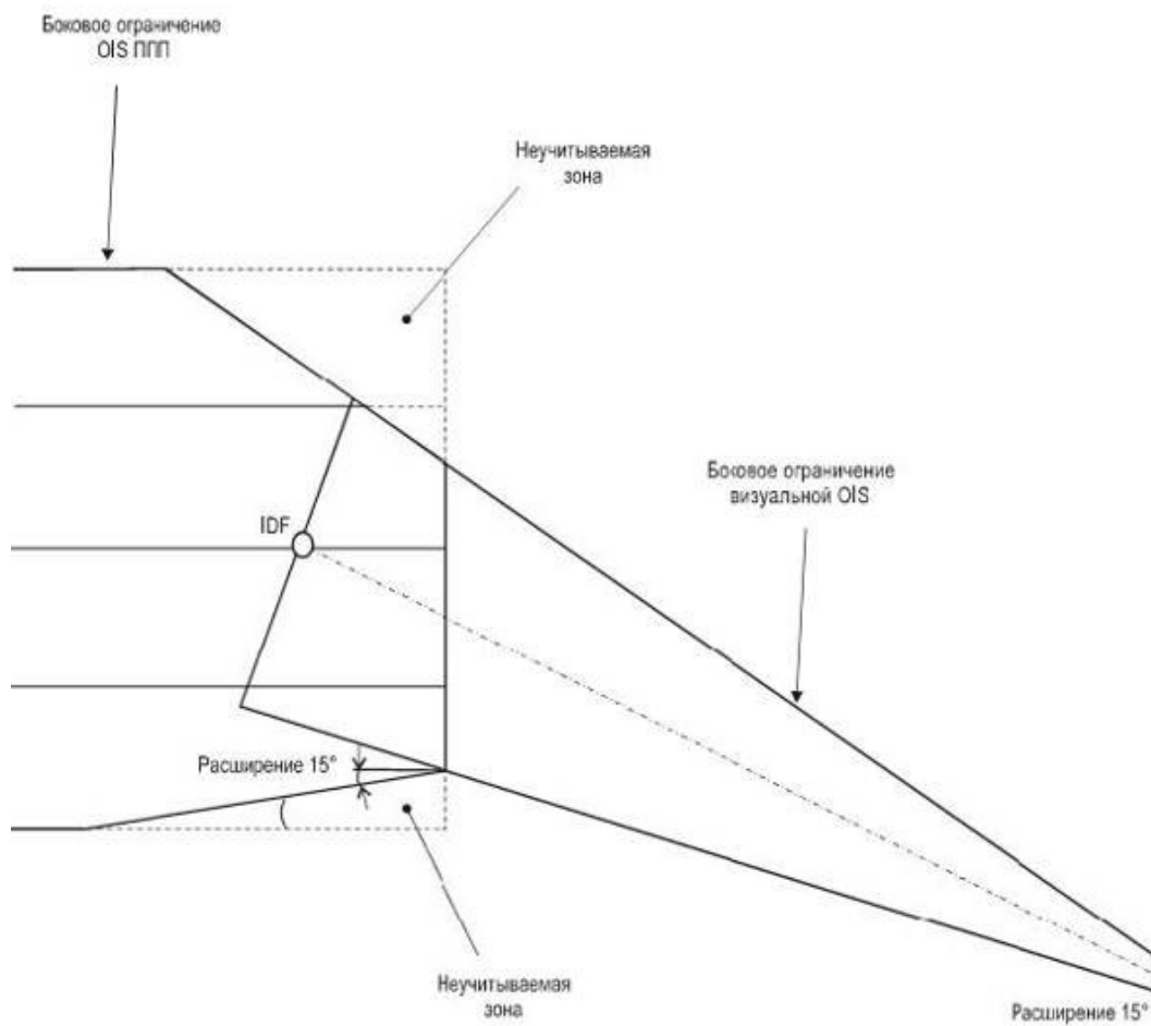
Рисунок IV-1-2 - Боковое сопряжение с изменением линии пути в IDF
