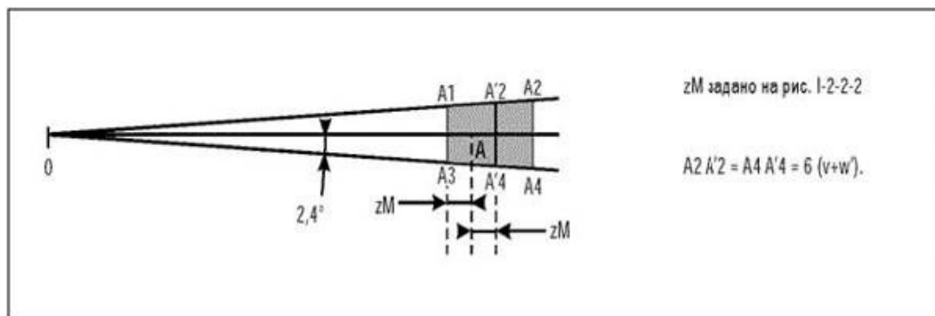
Рисунок I-4-3-Доб С-5 - Курсовой радиомаяк в 0 и маркерный радиомаяк в А
