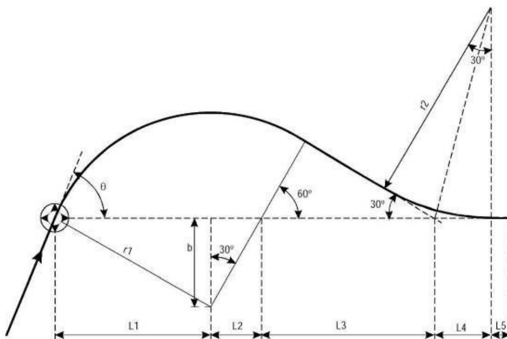
Рисунок III-2-1-7 - Минимальное расстояние стабилизации: точка пути "флайовер"
