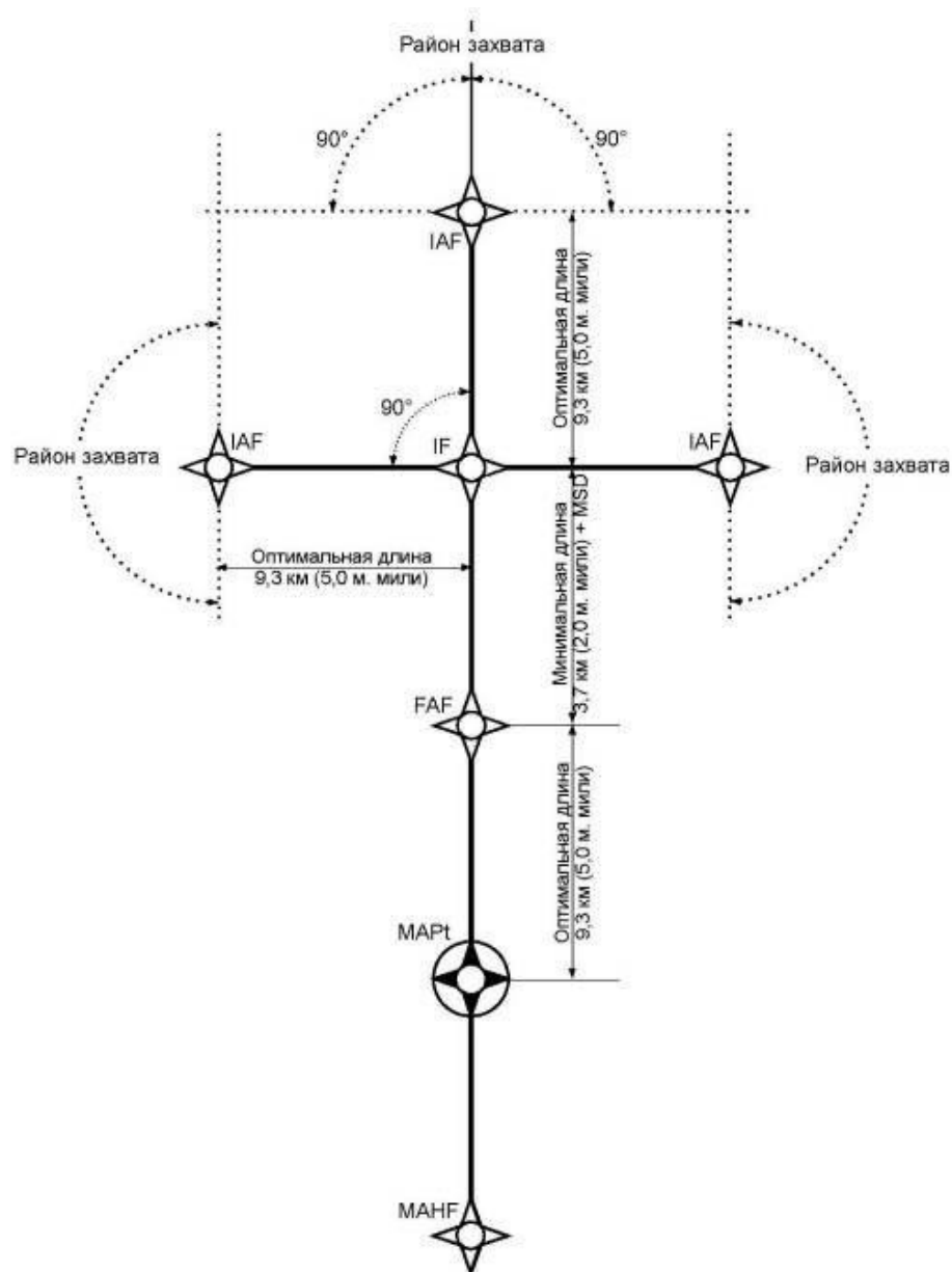
Рисунок III-2-3-1 - Общая Т-образная конфигурация
