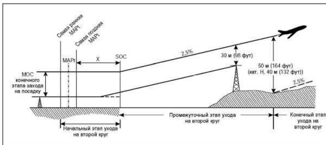
Рисунок I-4-6-4 - Запас высоты над препятствиями на конечном этапе ухода на второй круг
