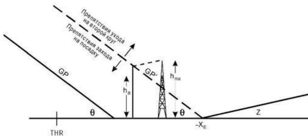
Рисунок III-3-5-7 - Препятствия ухода на второй круг до дальности - X E
