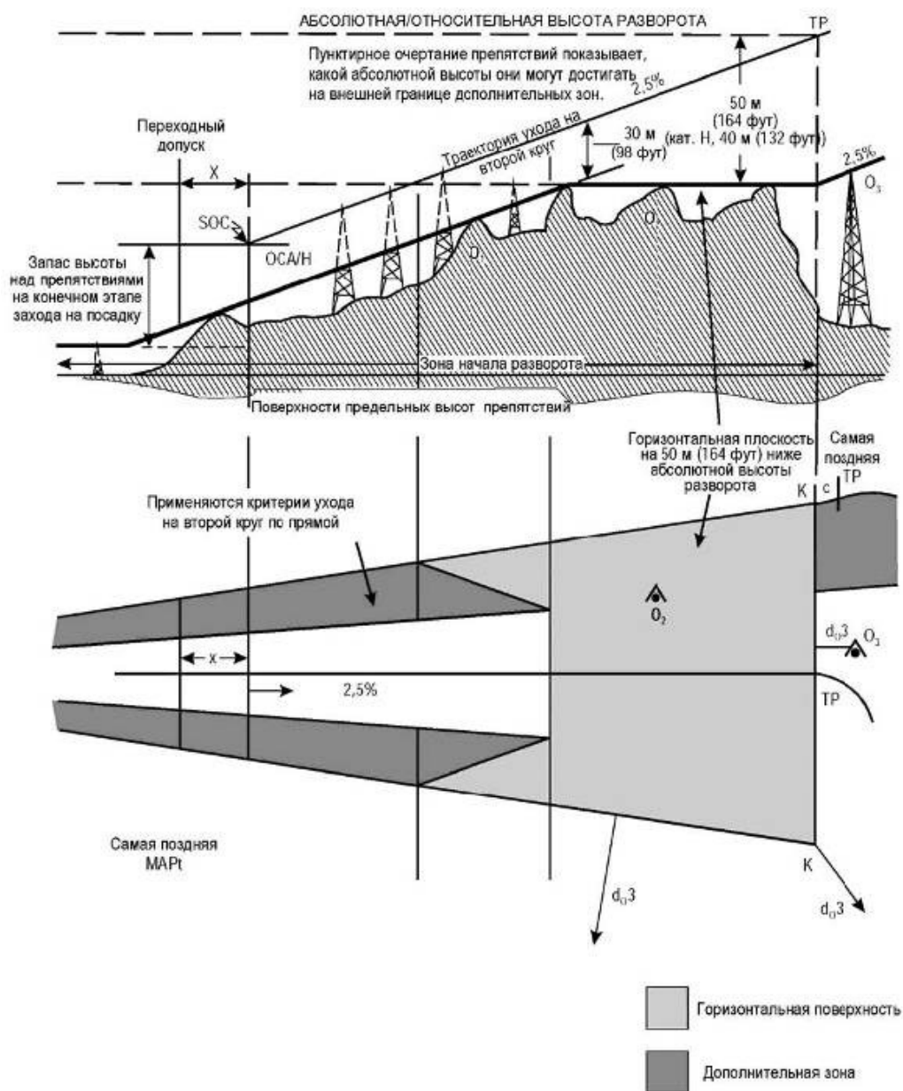
Рисунок I-4-6-13 - Запас высоты над препятствиями в пределах начала разворота
