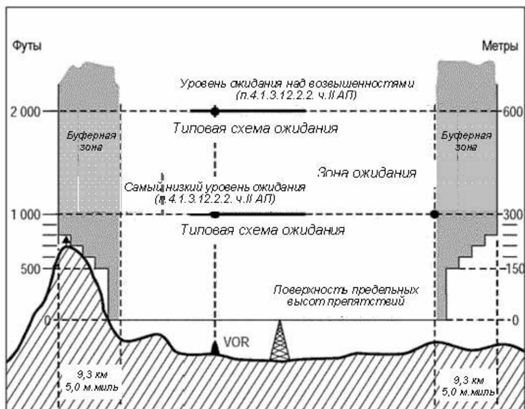
Рисунок II-4-1-5 - Зона ожидания для вертолетов до 1830м (6000 фут)
