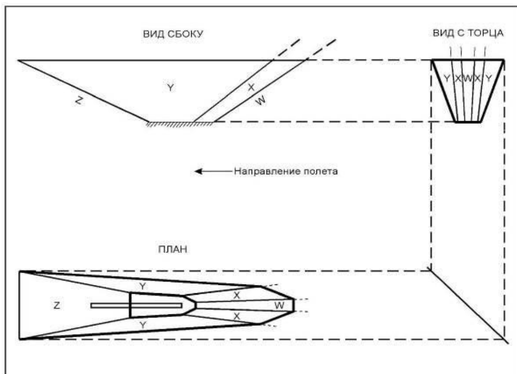
Рисунок II-1-3-9 - Поверхности оценки препятствий ILS
