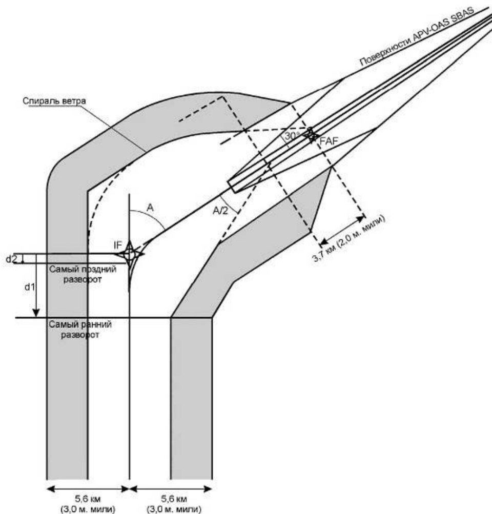
Рисунок III-3-2-4 - Разворот в точке пути "флай-бай" (SBAS)
