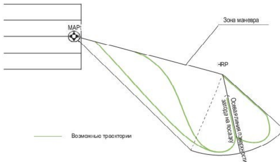
Рисунок IV-2-10 - Представление возможных траекторий, определяющих "зону маневра"
