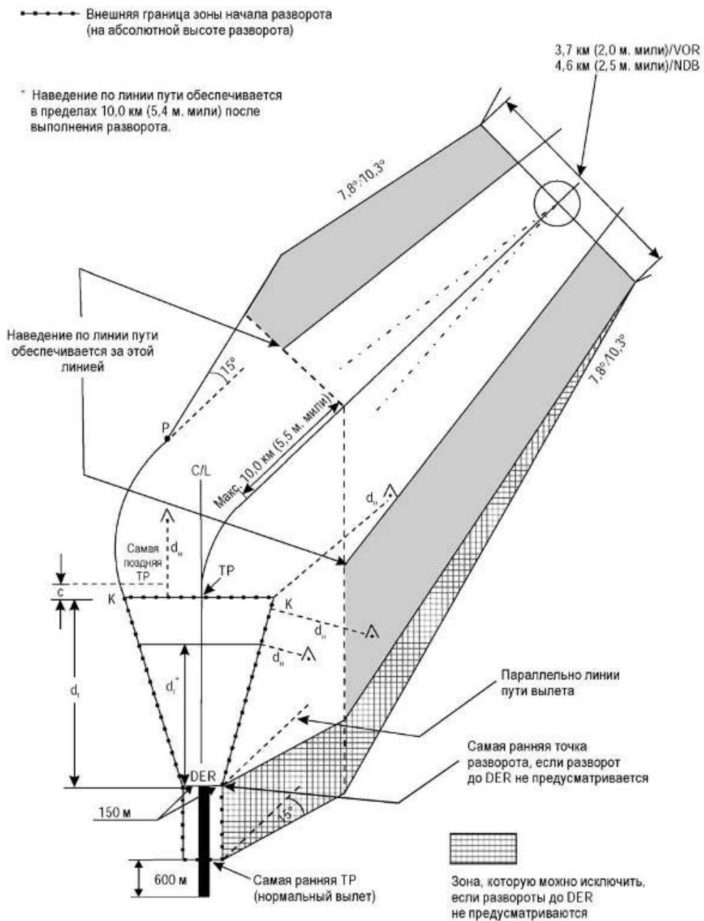
Рисунок I-3-3-9 - Вылет с разворотом: разворот на абсолютной высоте
