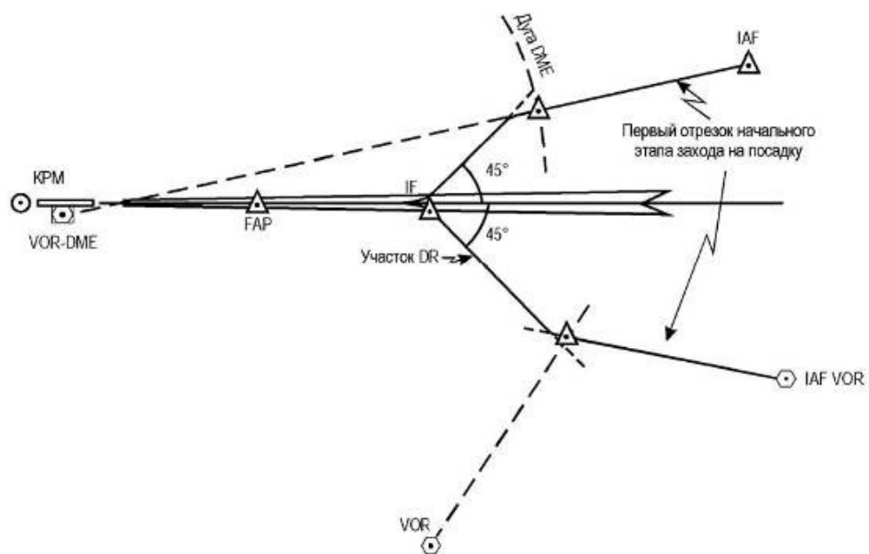
Рисунок I-4-3-Доб А-2 - Схема типа S
