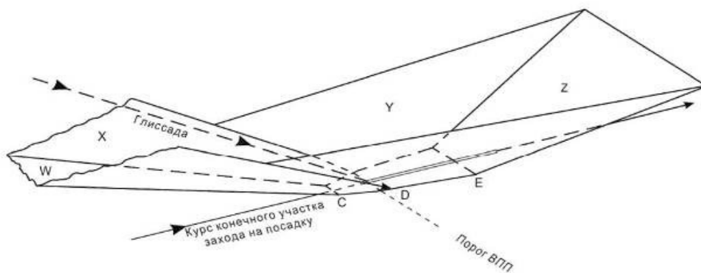
Рисунок II-1-1-9 - Поверхности оценки препятствий ILS. Вид в перспективе
