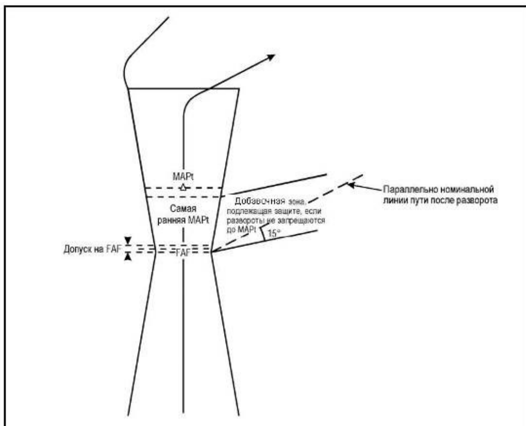
Рисунок I-4-6-14 - Ограничение ранних разворотов. Необходимость дополнительной защиты
