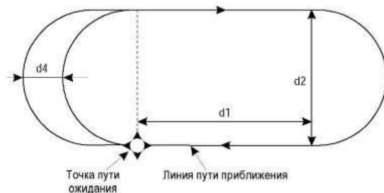
Рисунок III-3-7-3 - Максимальная линия пути при ожидании на основе RNP
