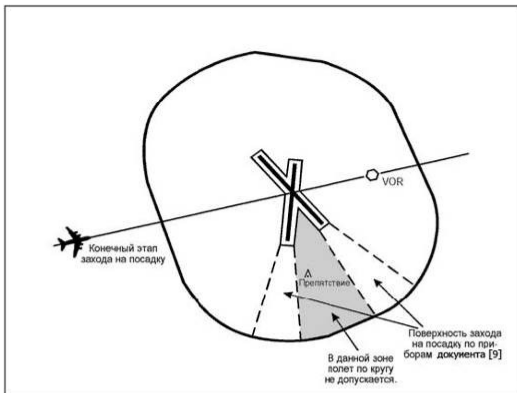
Рисунок I-4-7-4. Зона визуального маневрирования (полета по кругу). Запрет на полет по кругу
