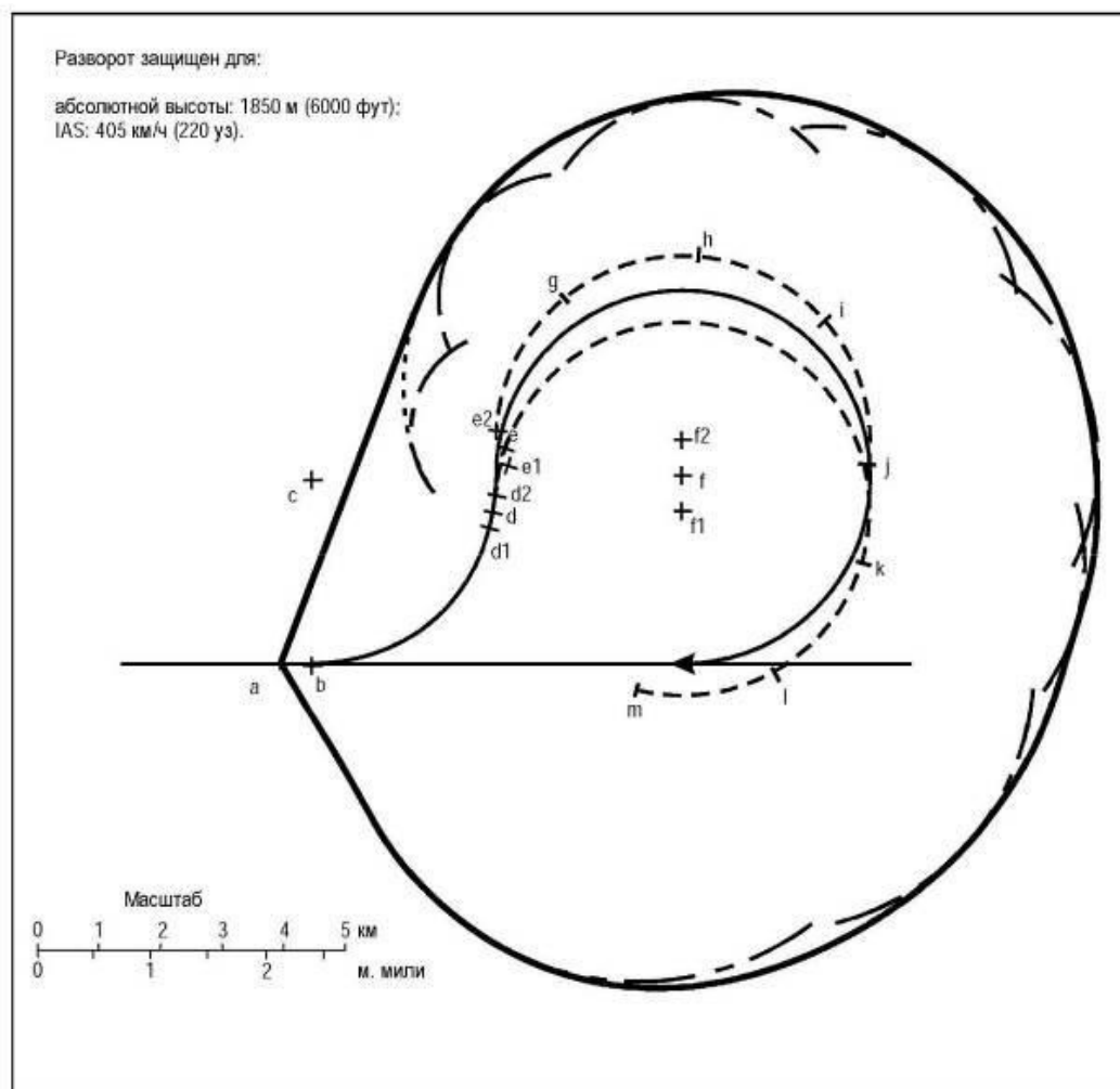
Диаграмма I-4-3-Доб С-4 - Шаблон стандартного разворота 80°-260°
