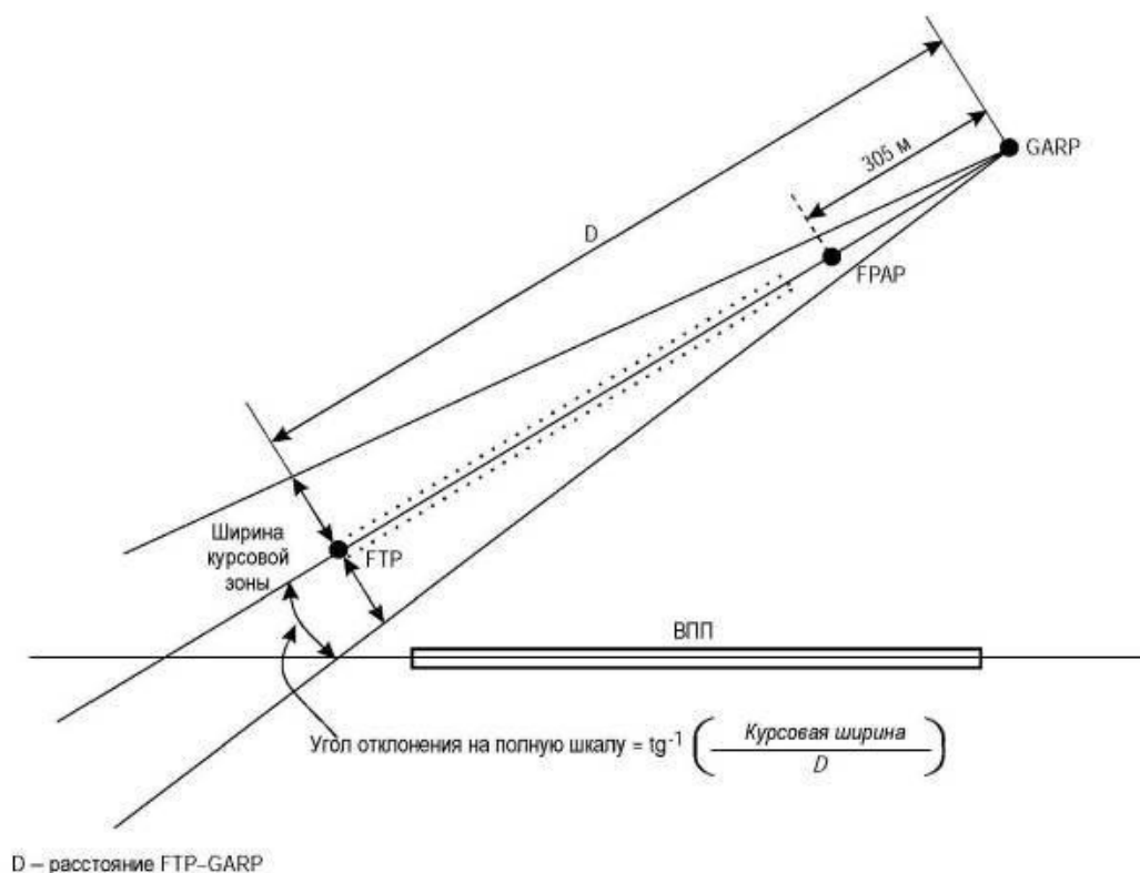
Рисунок III-3-6-18 - Выравнивание курса конечного этапа захода на посадку по GBAS категории I со смещенным азимутом
