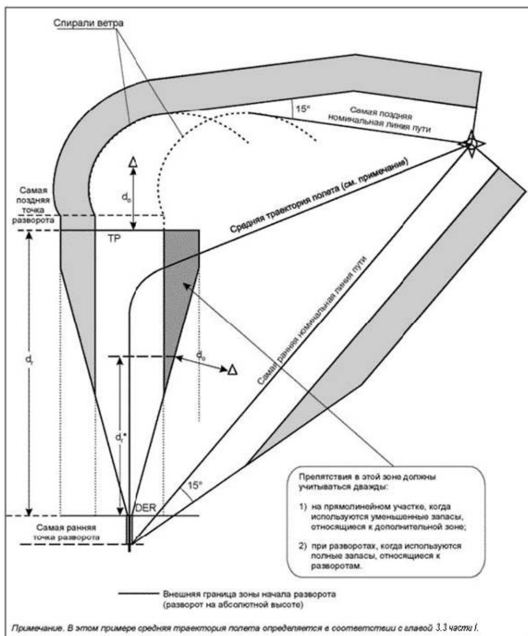
Рисунок III-3-1-5 - Разворот на абсолютной/относительной высоте в направлении точки пути
