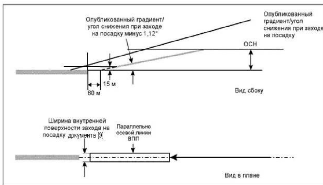
Рисунок I-4-5-7-а) - Поверхность визуального участка схемы с использованием курсового радиомаяка или бокового наведения с точностью курсового радиомаяка. Участок выровнен по осевой линии ВПП
