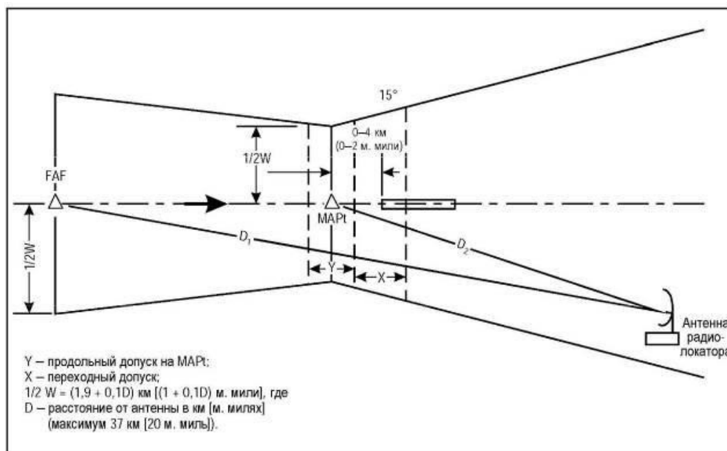
Рисунок II-2-6-3 - Заход на посадку по обзорному радиолокатору
