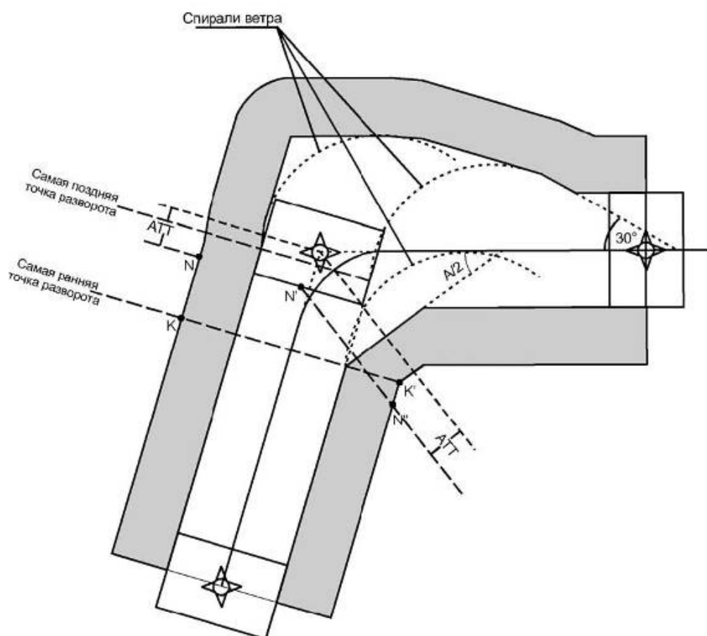
Рисунок III-2-2-2 - Разворот в точке пути "флай-бай": основная / дополнительная зоны вне разворота
