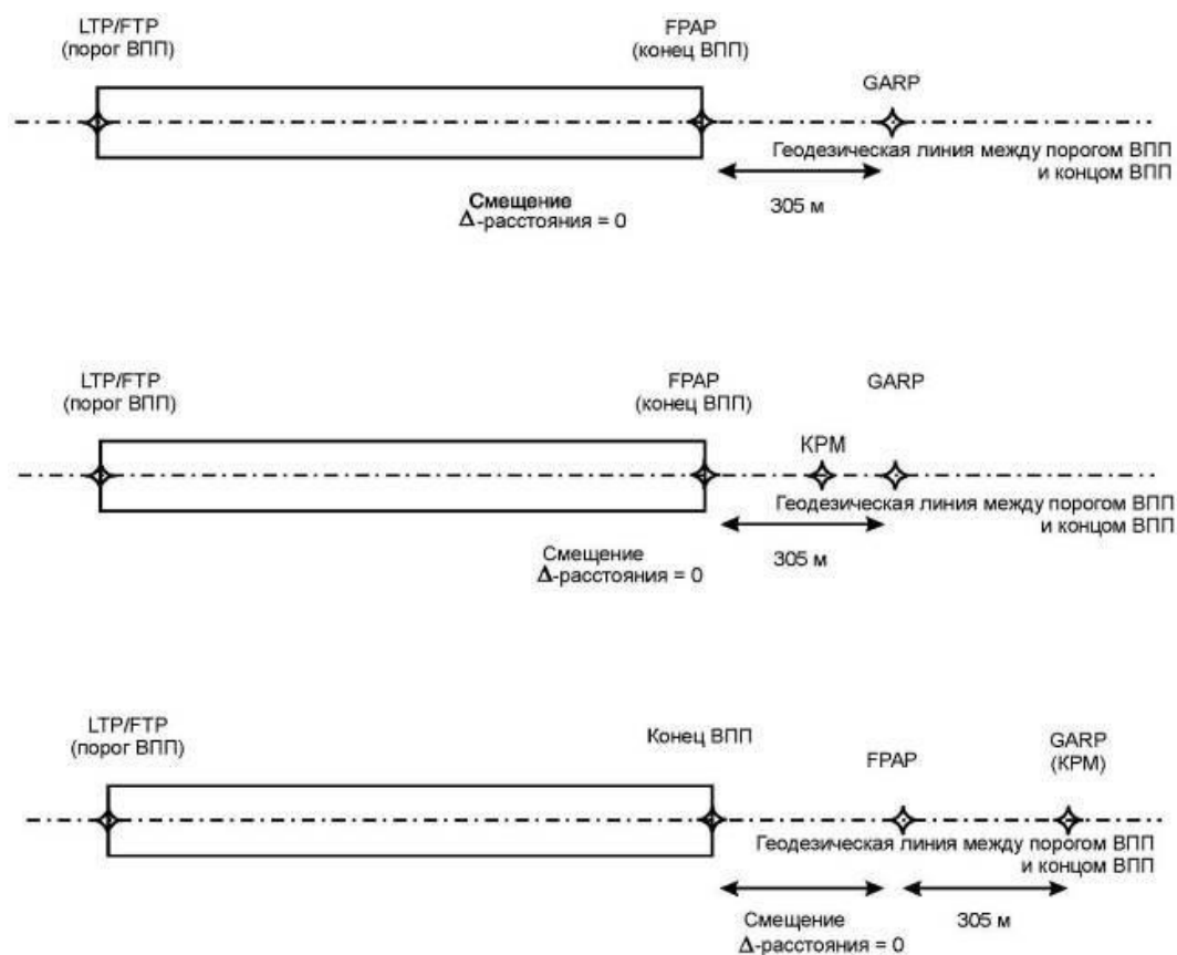
Рисунок III-2-6-2 - Местоположение FPAP (наличие ILS для захода на посадку и KPM в пределах 305 м от конца ВПП)
