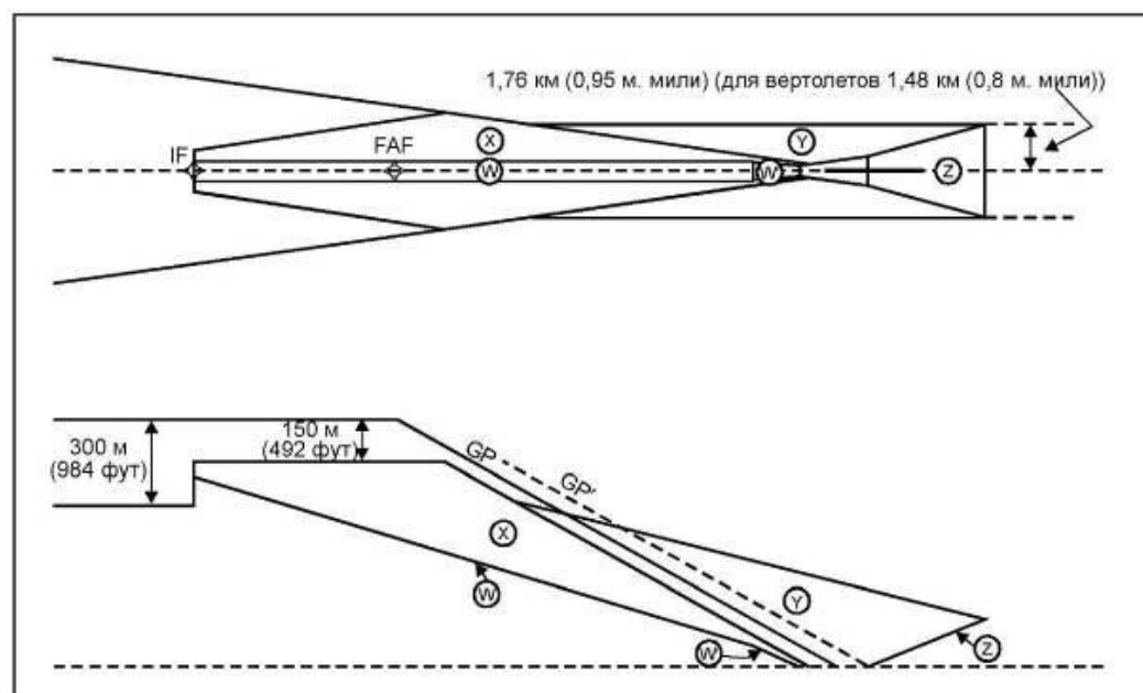
Рисунок III-3-5-2 - Иллюстрация APV-поверхностей оценки препятствий SBAS. Вид в плане и вид сбоку
