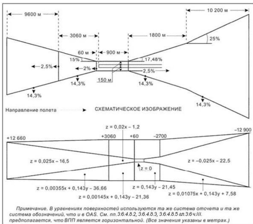
Рисунок III-3-6-6 - Уравнение поверхностей: основные поверхности ILS
