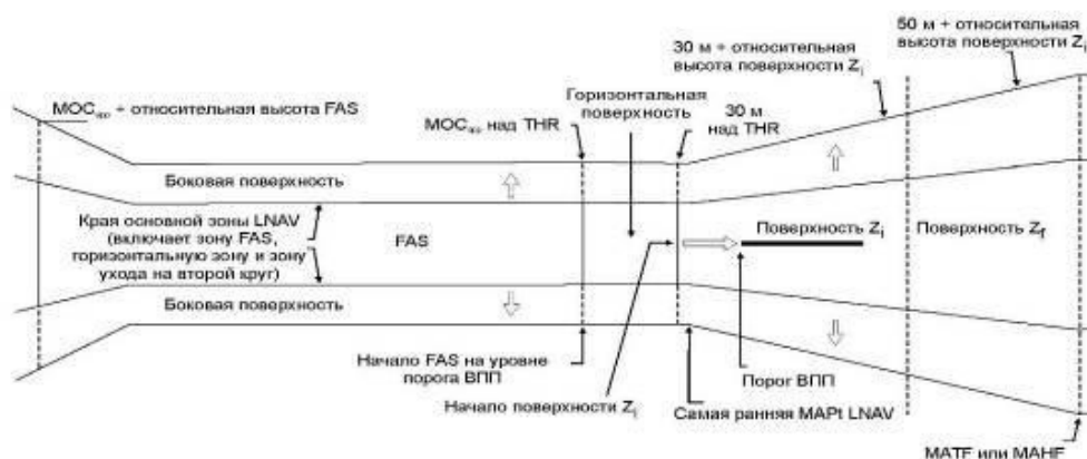
Рисунок III-3-4-1 - Зона APV/баро-VNAV. Вид APV OAS в плане
