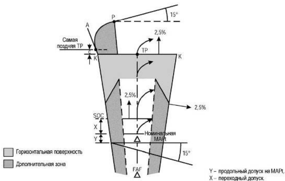
Рисунок I-4-6-12 - Разворот на абсолютной высоте более чем на 75°
