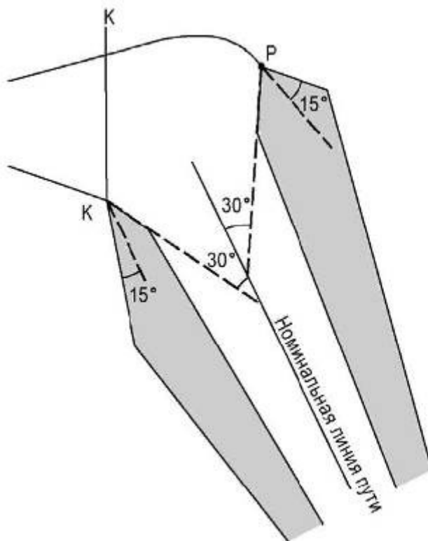
Рисунок 1-2-3-6 - Построение дополнительных зон при наличии дополнительного наведения по линии пути
