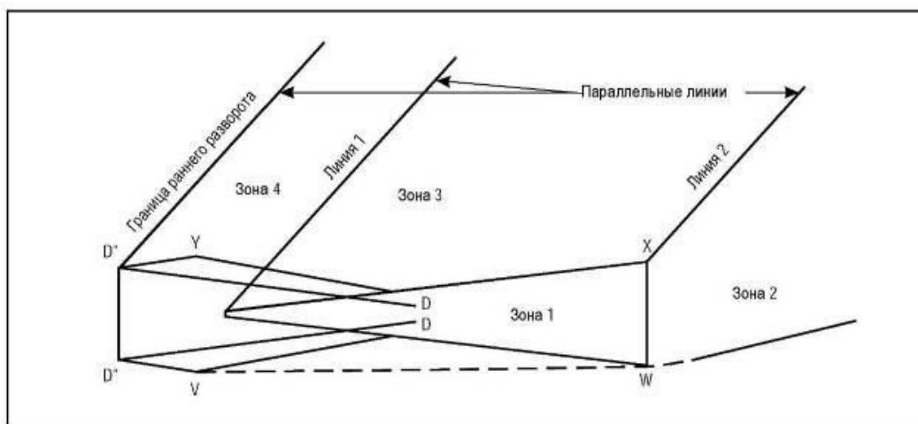
Рисунок II-1-1-Доб А-5 - Зоны применения запаса высоты над препятствиями (TNH = 90 м)
