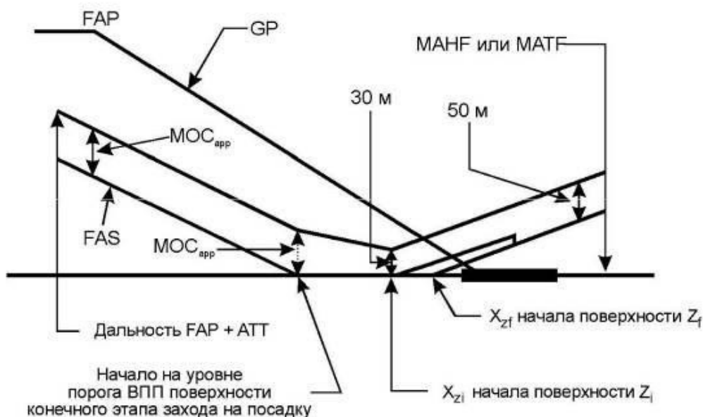
Рисунок III-3-4-2 - Баро-VNAV. Вид в профиль
