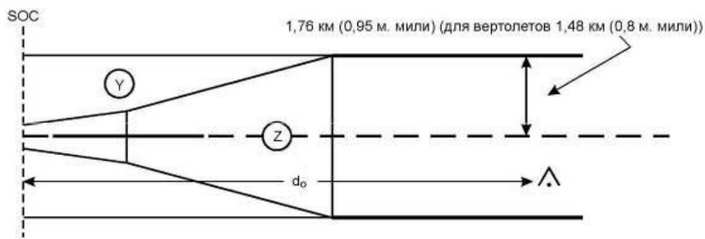
Рисунок III-3-5-8 - Конечный участок ухода на второй круг по прямой
