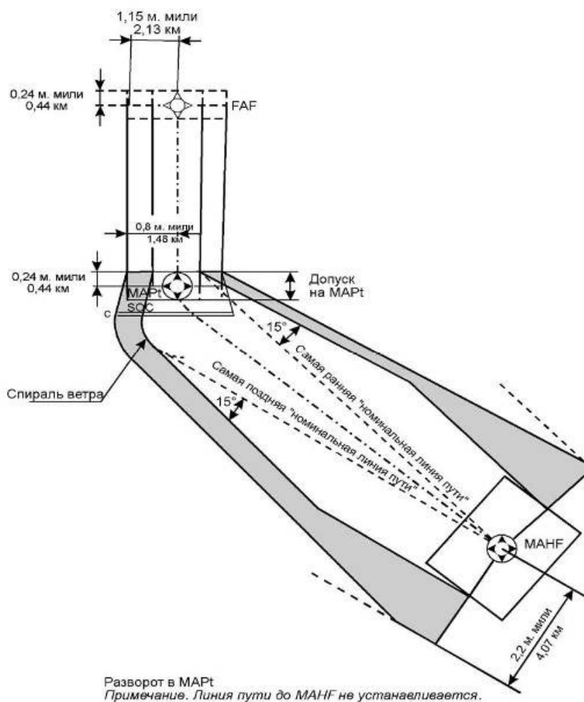
Рисунок IV-2-2 - Уход на второй круг с разворотом
