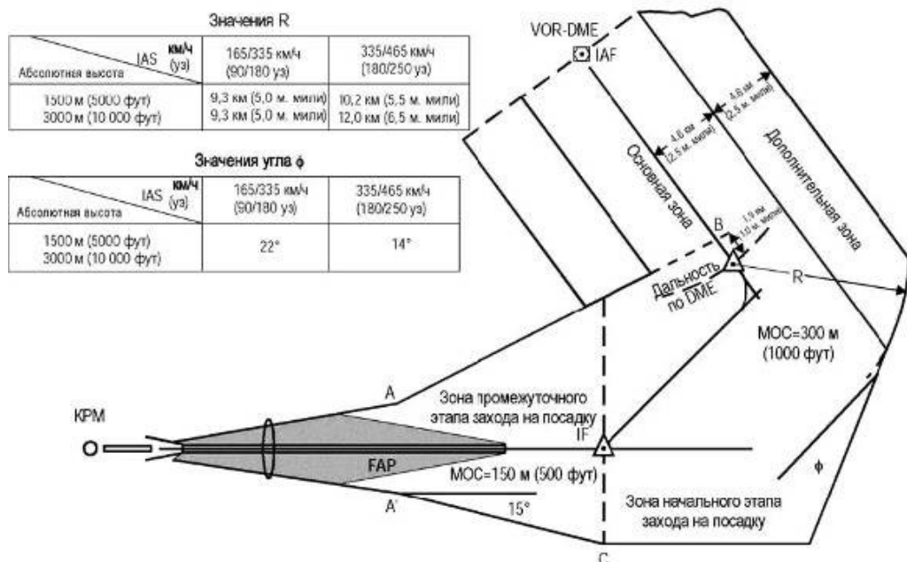
Рисунок I-4-3-Доб А-4 - Построение зон защиты в схеме типа U VOR/DME
