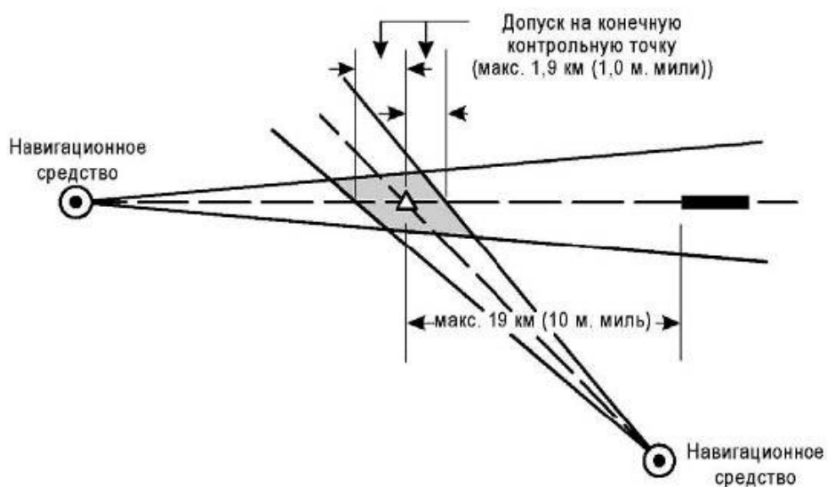
Рисунок 1-2-2-6 - Допуск на конечную контрольную точку захода на посадку (FAF)
