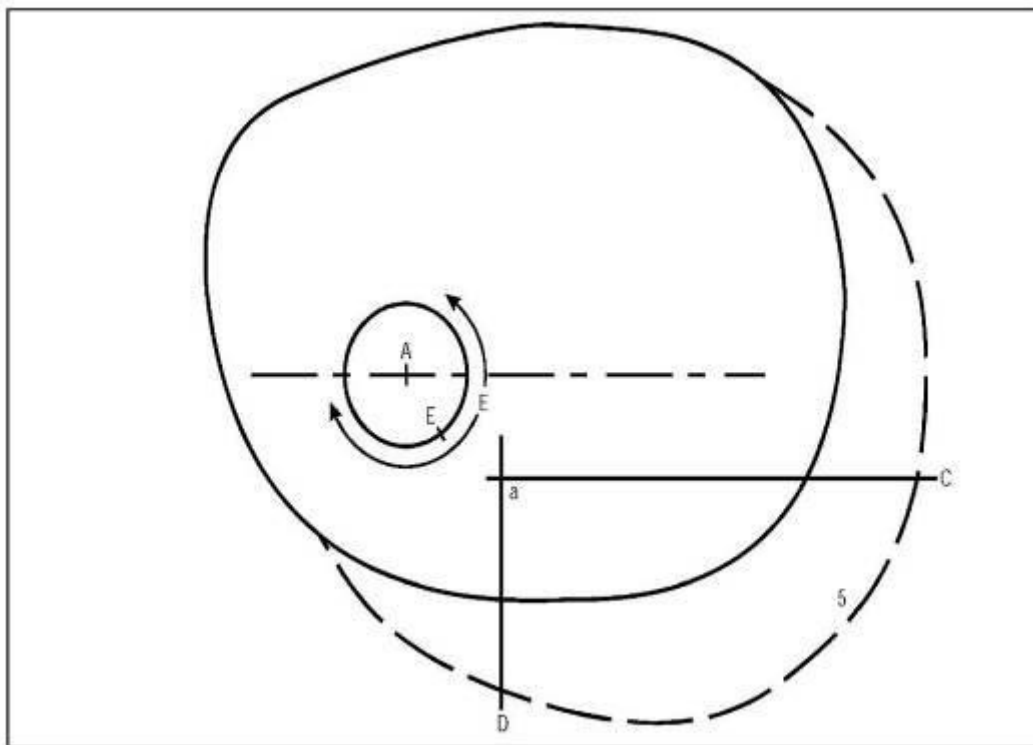
Диаграмма I-4-3-Доб С-10 - Построение зоны входа применение точки E, ось шаблона параллельна оси схемы
