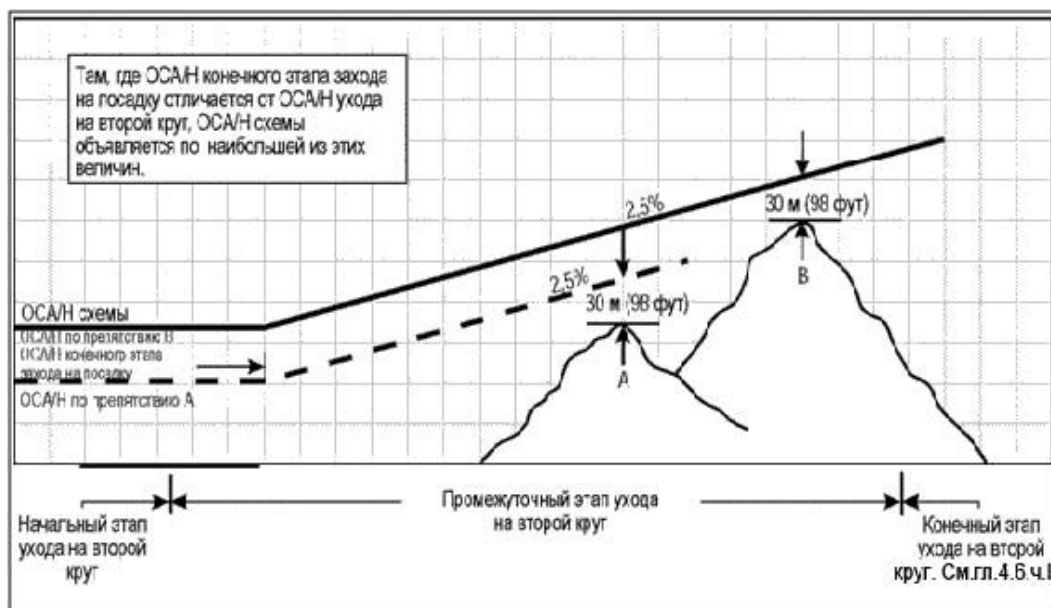
Рисунок II-1-5-5 - Определение OCA/H ухода на второй круг по PAR
