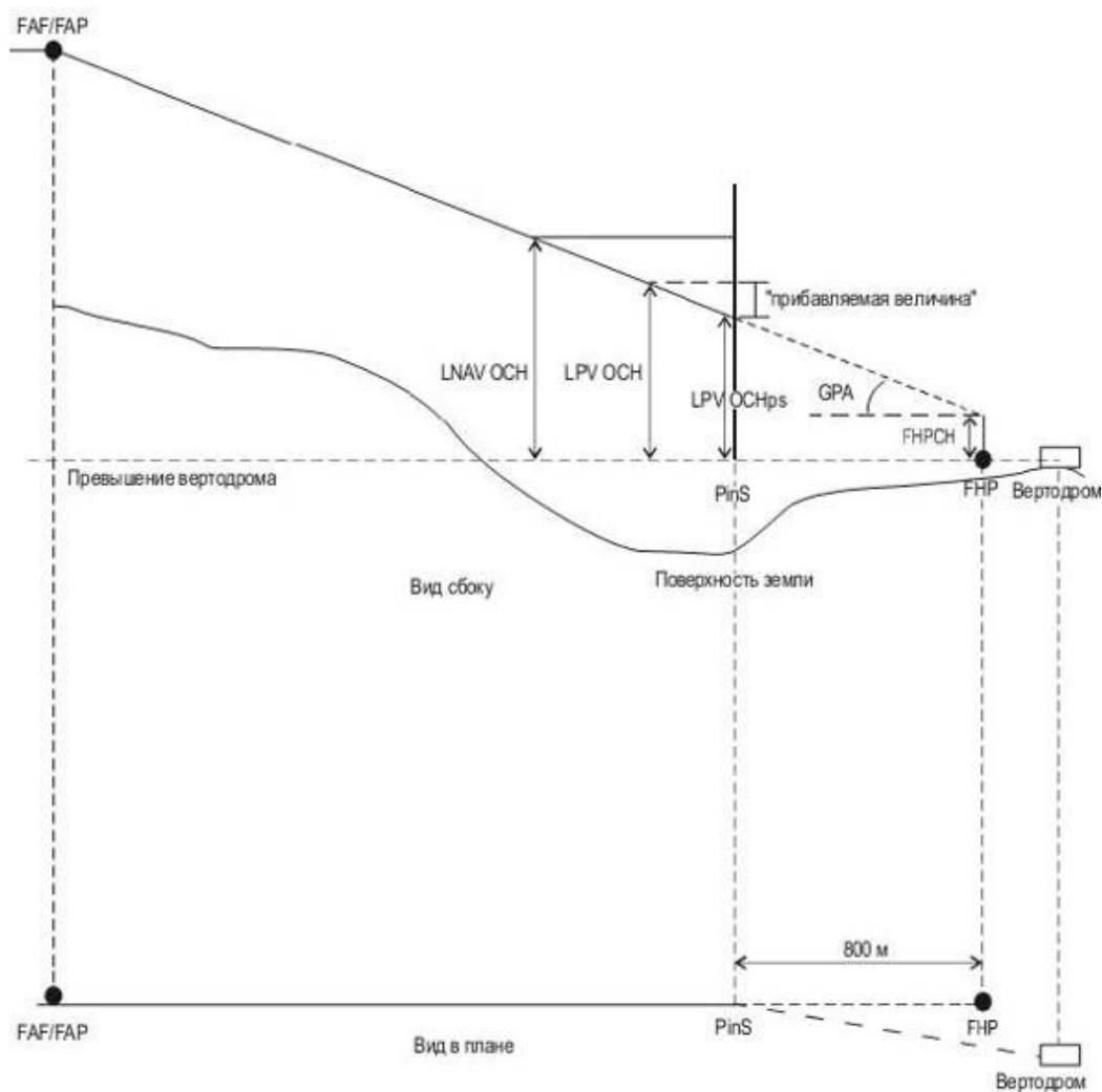
Рисунок IV-3-1 - Представление схемы захода на посадку RNP APCH до PinS с использованием минимумов LNAV и LPV
