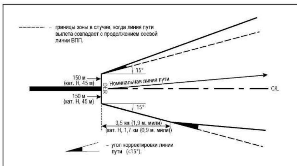
Рисунок I-3-3-2 - Зона вылета по прямой с корректировкой линии пути (точка корректировки линии пути не установлена)
