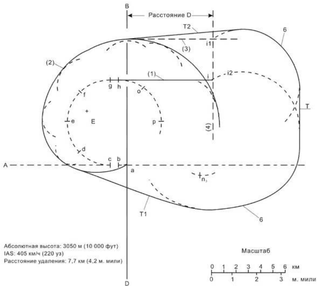
Рисунок III-3-7-Доб А-1 - Шаблон RNAV для систем RNAV с функцией ожидания
