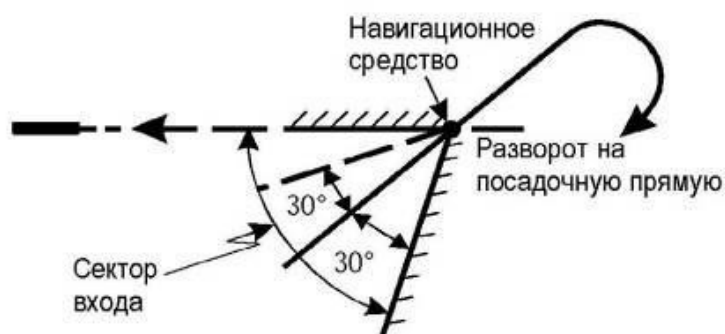
Рисунок I-4-3-5 - Вход в разворот на посадочную прямую
