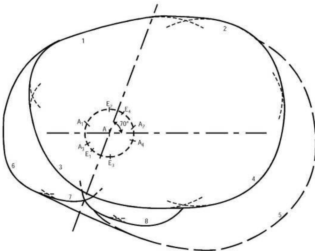
Диаграмма I-4-3-Доб С-12 - Основная зона с зонами входа с любого направления; схема для пролета над средством
