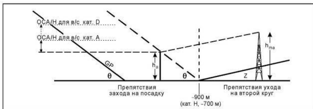
Рисунок II-1-1-13 - Препятствие ухода на второй круг, расположенное за дальностью - 900 м
