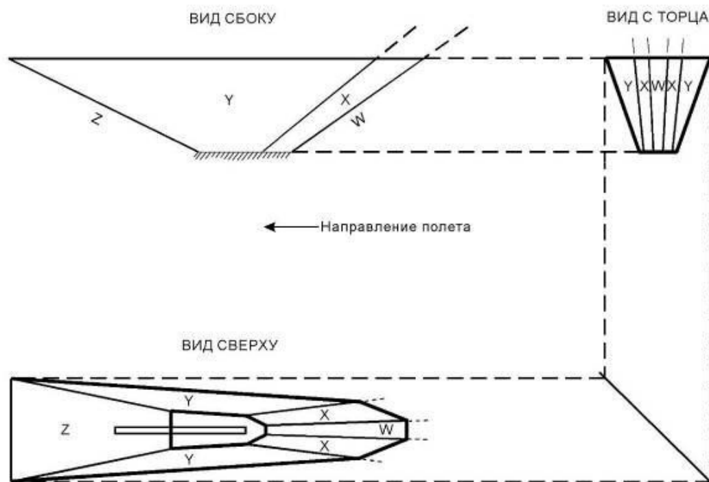
Рисунок III-3-6-7 - Поверхности оценки препятствий для ILS для полетов по GBAS
