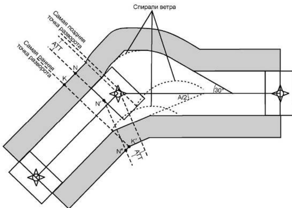
Рисунок III-2-2-5 - Линия N-N'-N": разворот в точке пути "флай-бай" под углом \leq 90^\circ
