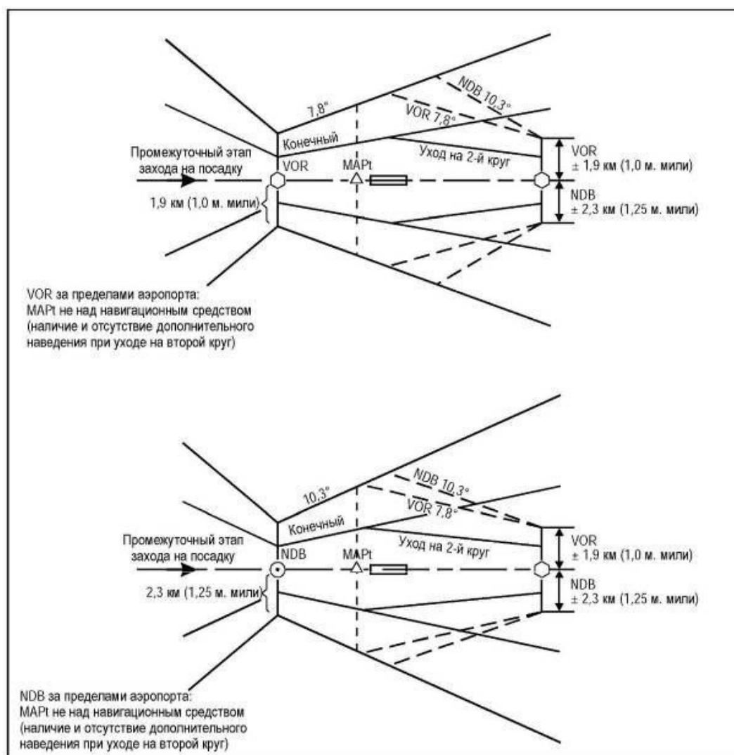
Рисунок I-4-6-8 - Зоны, соответствующие дополнительному наведению по направлению, в случае, когда MAPt находится не в месте расположения
