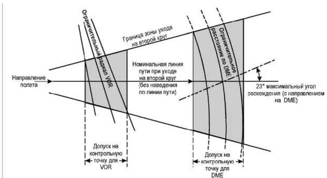
Рисунок 1-2-2-7 - Расчетные зоны допуска на контрольную точку для ограничительного радиала/азимута или расстояния по DME
