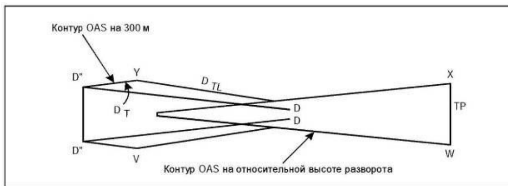
Рисунок II-1-1-Доб А-3 - Зона начала разворота (относительная высота разворота 90 м)
