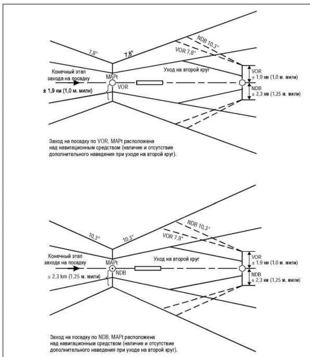
Рисунок I-4-6-7 - Зона, соответствующая дополнительному наведению, когда MAPt определяется навигационным средством
