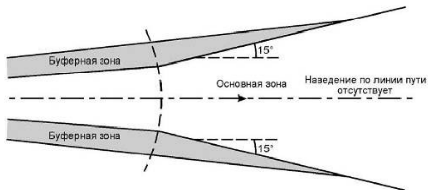
Рисунок II-3-1-8 - Зона без наведения по линии пути
