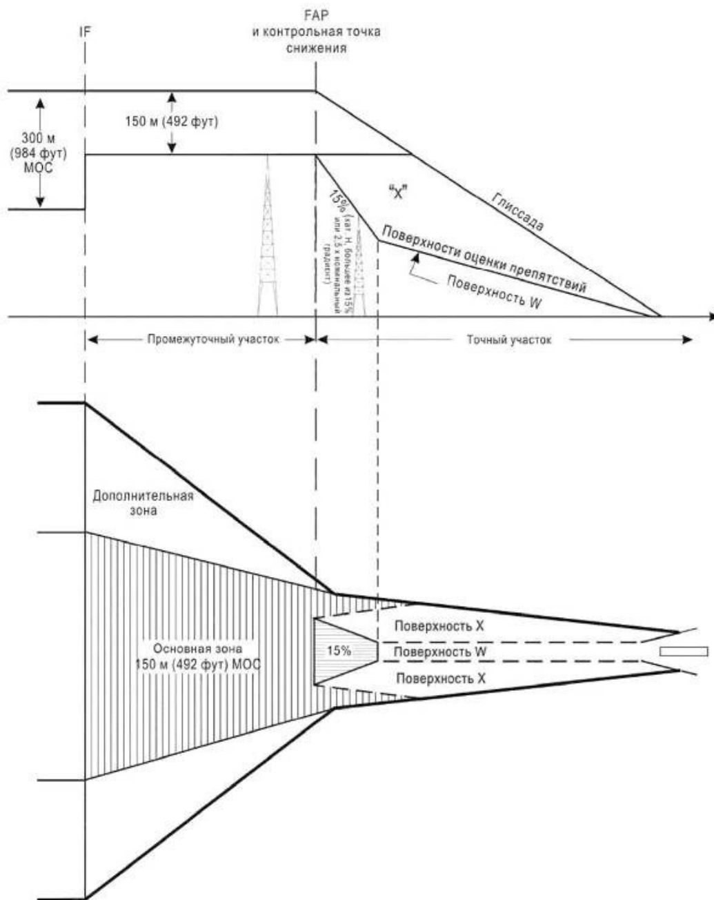
Рисунок III-3-6-2 - Конечная контрольная точка захода на посадку, определяемая контрольной точкой снижения
