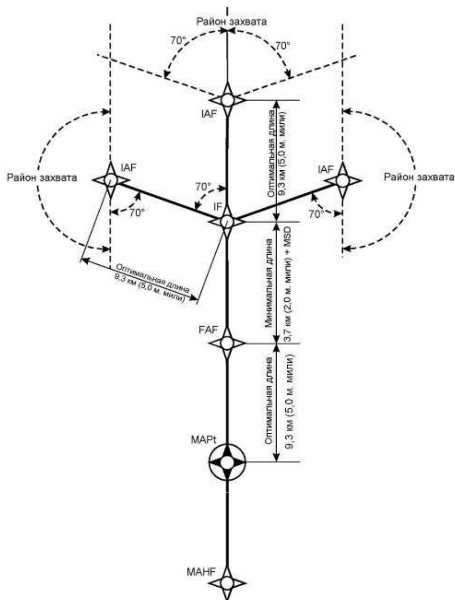
Рисунок III-2-3-2 - Общая Y-образная конфигурация
