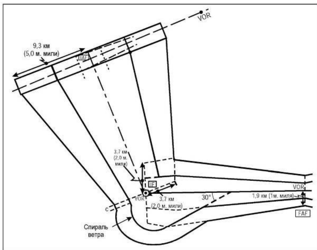
Рис. I-4-3-Доб В-5 - Уменьшение ширины зоны: начальный участок стыкуется с промежуточным участком при развороте
