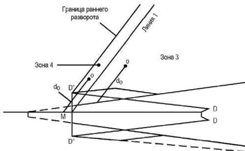
Рисунок II-1-1-Доб А-8 - Случай, когда TNH превышает 140 м (приблизительно) (разворот менее чем на 75^\circ )
