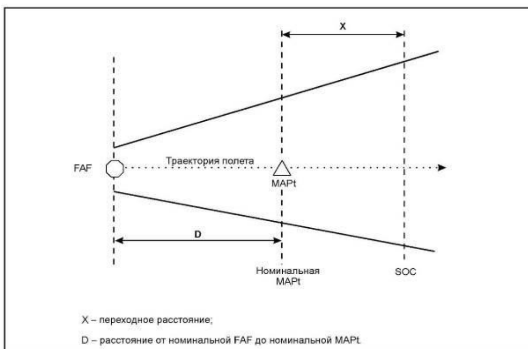
Рисунок I-4-6-2 - Определение SOC в случае, когда MAPt определяется расстоянием от FAF
