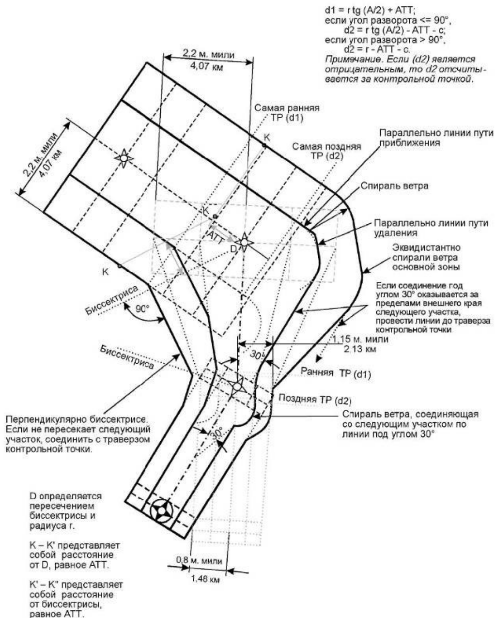
Рисунок IV-2-1 - Начальный, промежуточный и конечный участки захода на посадку
