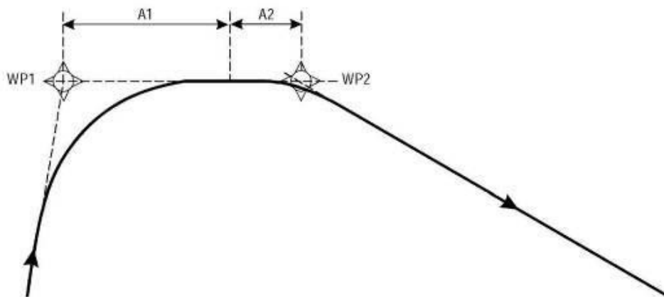
Рисунок III-2-1-2 - Две точки пути "флай-бай"
