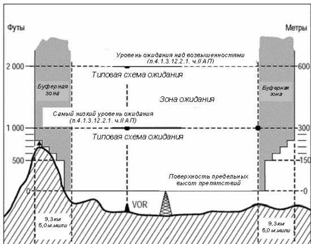
Рисунок II-4-1-4 - Минимальный уровень ожидания, определяемый поверхностью предельных высот препятствий в зоне ожидания и буферной зоне
