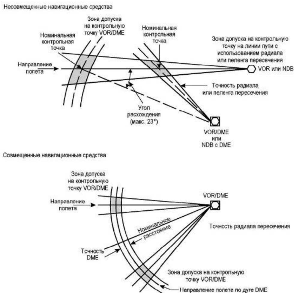
Рисунок 1-2-2-1 - Зоны допуска на контрольные точки пересечения
