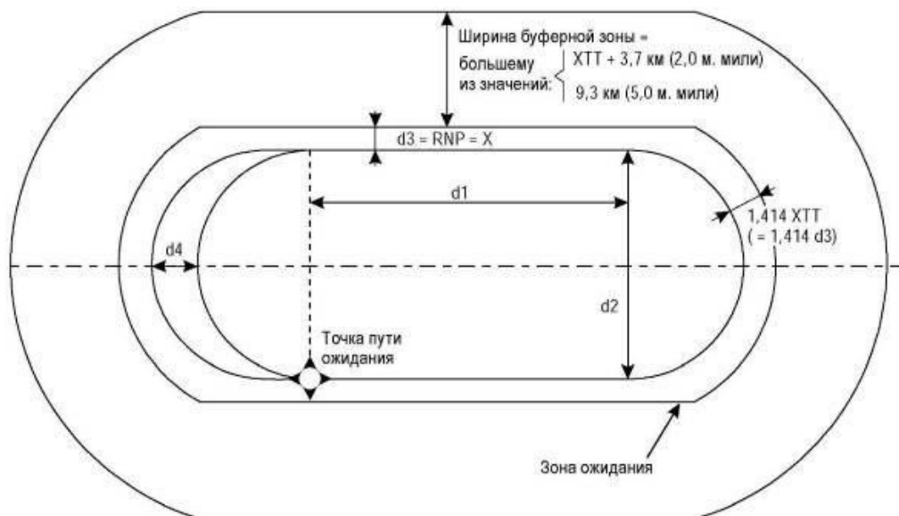
Рисунок III-3-7-4 - Зона ожидания, основанная на RNP: зона запаса высоты над препятствиями
