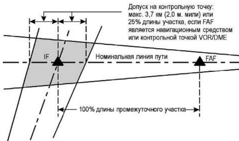
Рисунок 1-2-2-5 - Допуск на контрольную точку в пределах промежуточного участка захода на посадку
