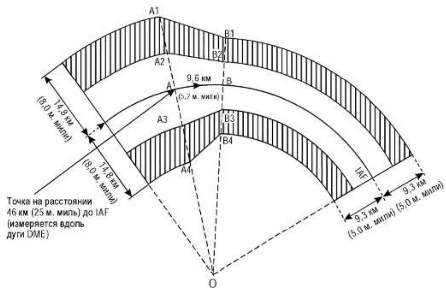
Рисунок I-4-2-3 - Дуга DME (длина участка прибытия больше или равна 46 км (25 м. миль))
