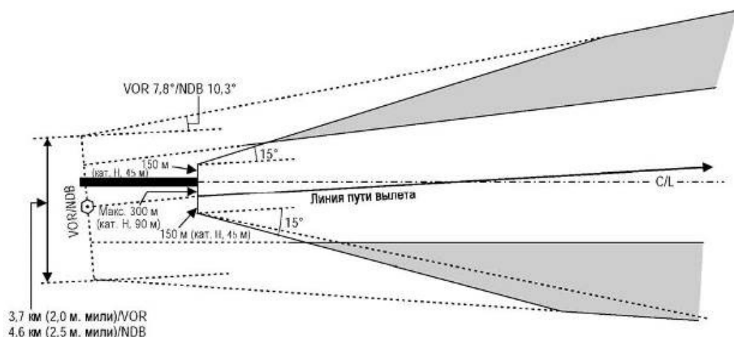
Рисунок I-3-3-8 - Вылет по прямой со смещенным курсом вылета. Линия пути пересекает направление ВПП
