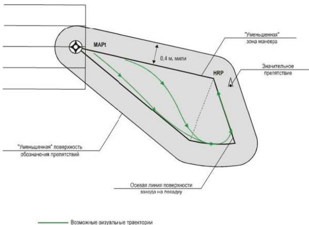
Рисунок IV-2-17 - Метод уменьшения ОСА/Н: уменьшенная "зона маневра" и горизонтальная OIS
