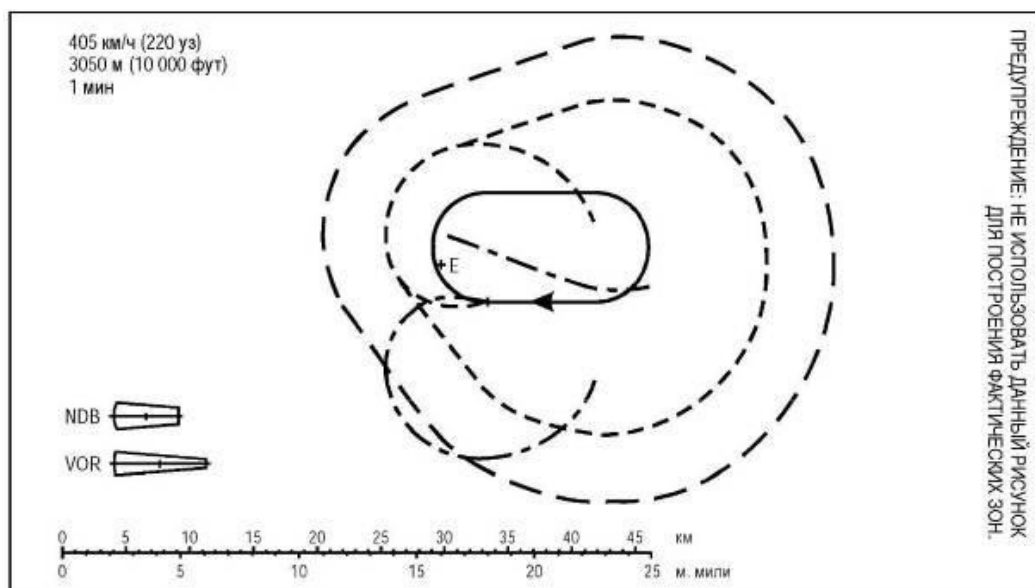
Диаграмма I-4-3-Доб С-8 - Шаблон схемы "ипподром" из [7]
