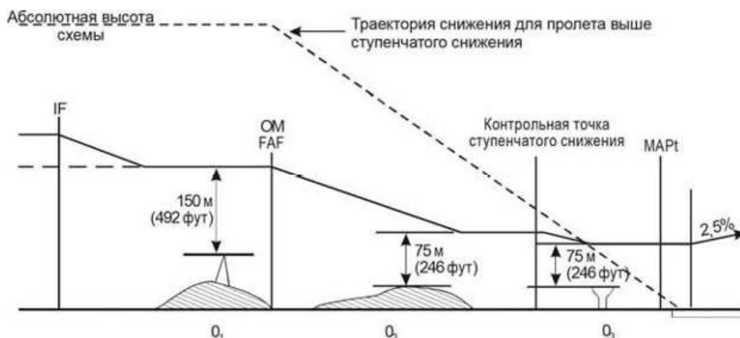
Рисунок II-2-2-2 - Схема только для азимутального оборудования. Запас высоты над препятствиями и абсолютная высота схемы
