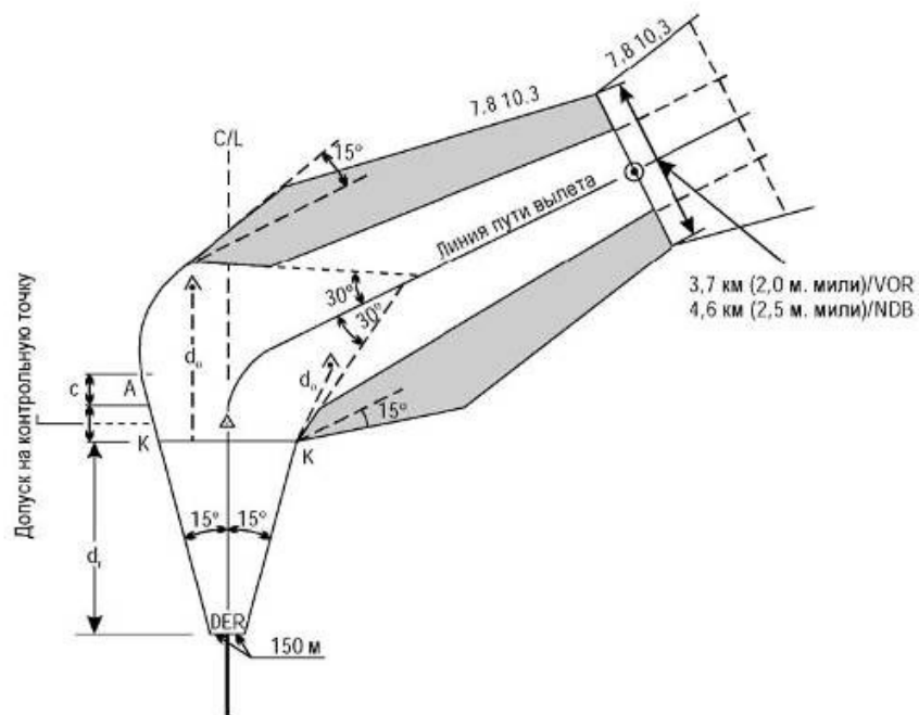
Рисунок I-3-3-11. с) - Вылет с разворотом. Первый разворот в контрольной точке
