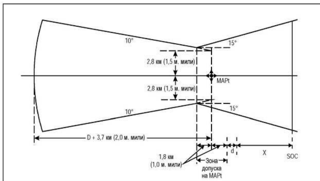
Рисунок II-2-5-2 - Зона конечного этапа захода на посадку
