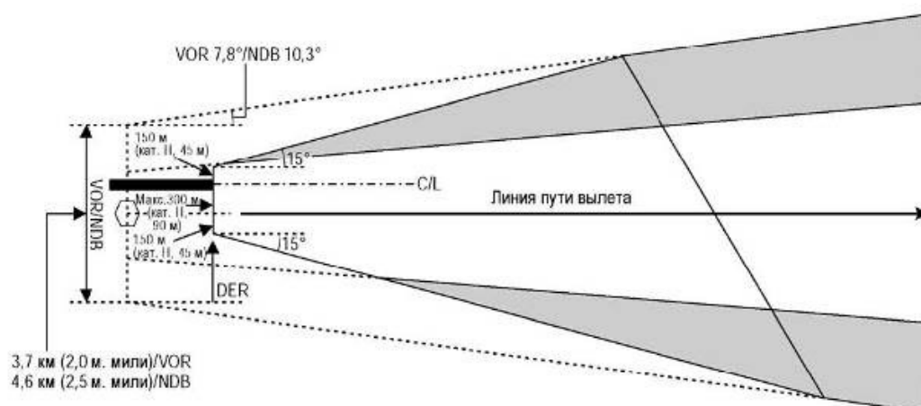
Рисунок I-3-3-6 - Вылет по прямой со смещенным курсом вылета. Линия пути параллельна направлению ВПП
