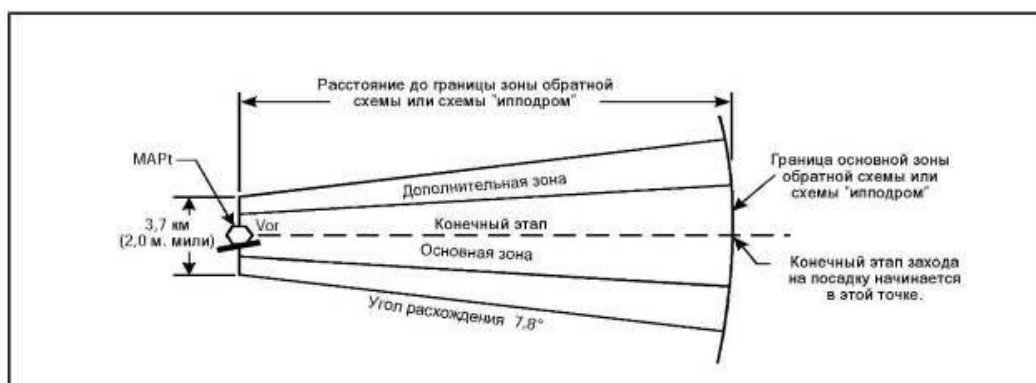
Рисунок II-2-3-1 - Зона конечного этапа захода на посадку (VOR)
