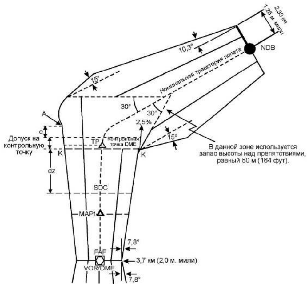
Рисунок I-4-6-15 - Уход на второй круг с разворотом при наличии DME в качестве контрольной точки TP
