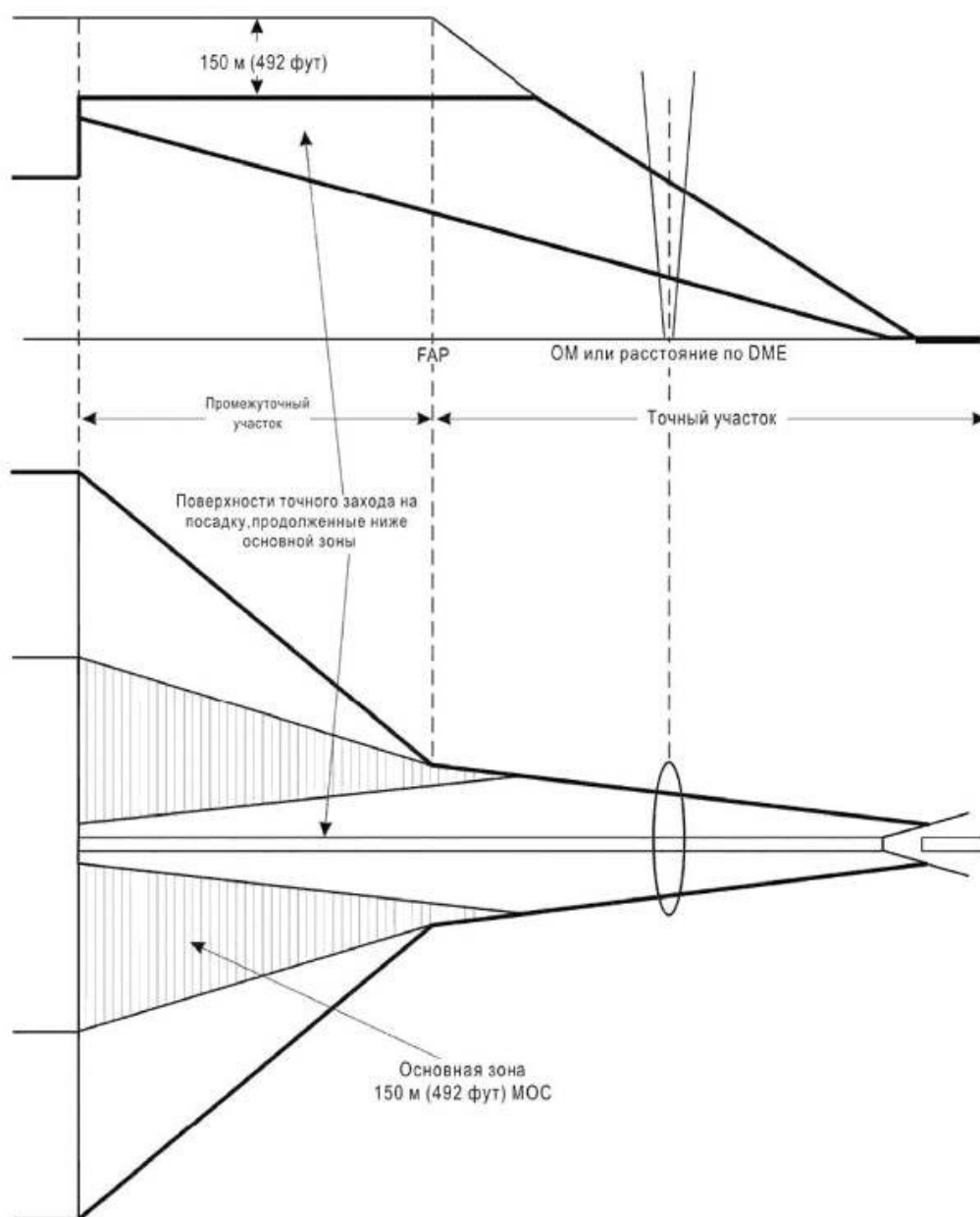
Рисунок II-1-3-4 - Точный участок при отсутствии конечной контрольной точки захода на посадку
