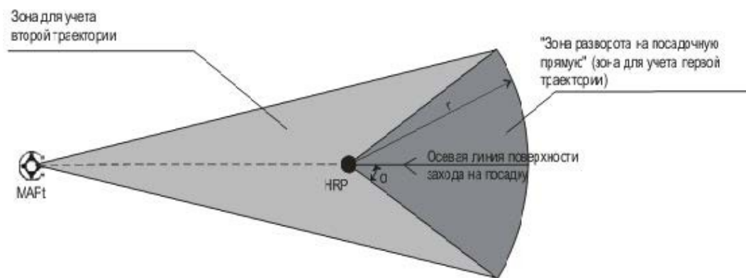
а) "Зона разворота на посадочную прямую" по обе стороны от линии MAPt-HRP
