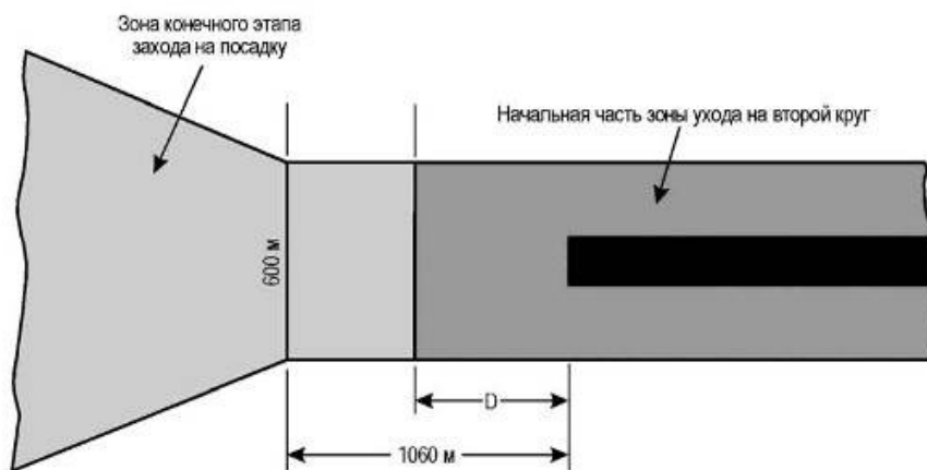
Рисунок II-1-5-4 - Зоны конечного этапа захода на посадку и начального этапа ухода на второй круг по посадочному радиолокатору
