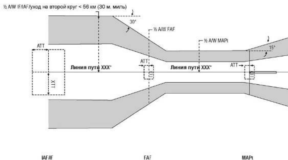
Рисунок III-3-3-2 - Зоны на основе RNP APCH
