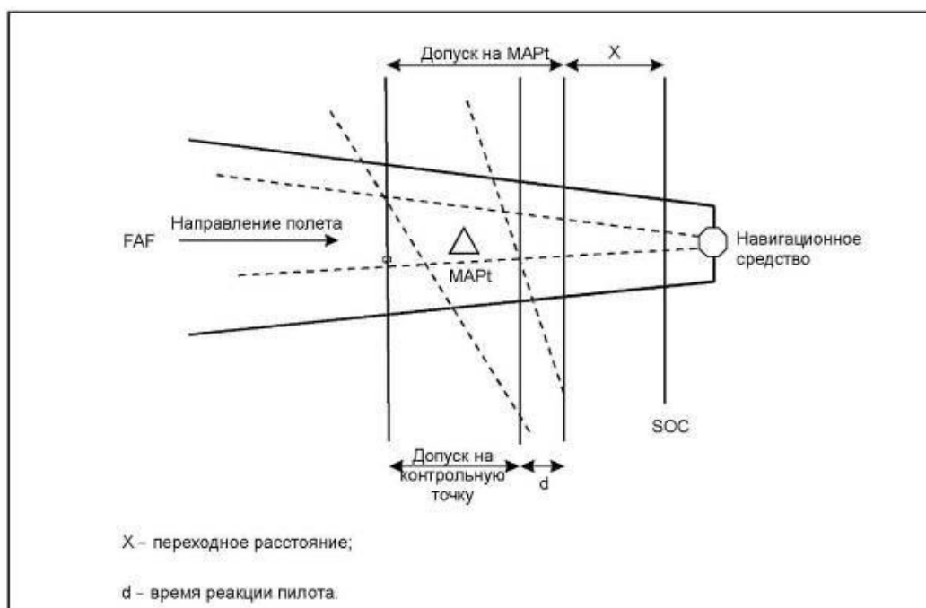
Рисунок I-4-6-1 - Определение SOC в случае, когда MAPt определяется навигационным средством или контрольной точкой
