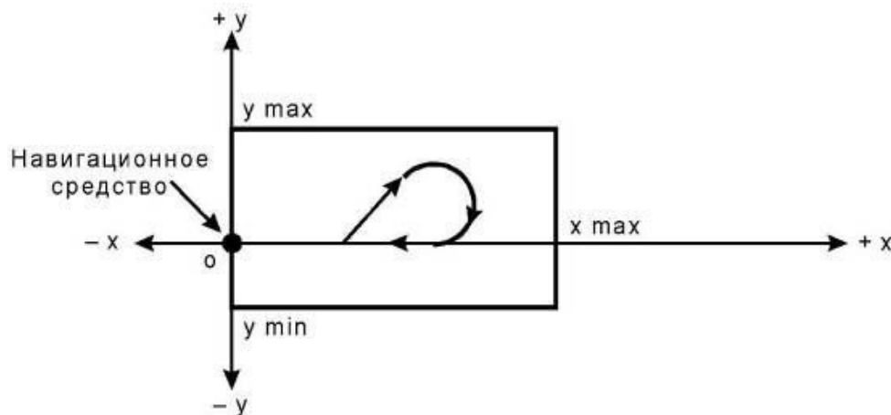
Рисунок I-4-3-Доб С-18 - Построение упрощенной схемы: пример прямоугольника для стандартного разворота
