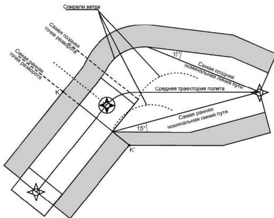
Рисунок III-2-2-6 - Разворот в точке пути "флайовер", после которого следует участок DF. Малый угол разворота
