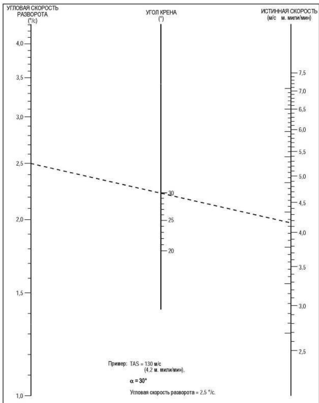
Рисунок II-4-1-Доб А-3 - Угловая скорость разворота в зависимости от угла крена и истинной скорости
