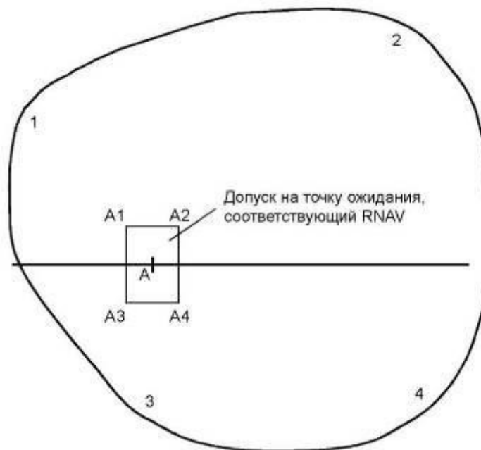
Рисунок III-3-7-Доб А-4 - Основная зона ожидания RNAV для системы RNAV без функции ожидания. Участок удаления определяется по времени
