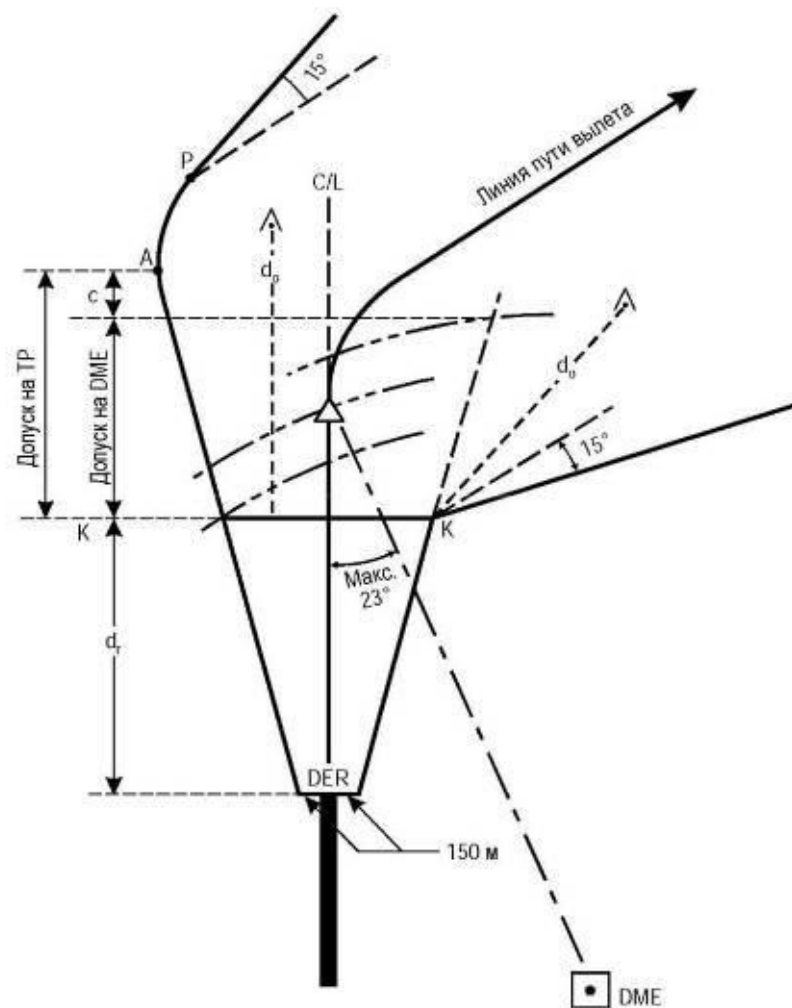
Рисунок I-3-3-11. б) - Точка разворота, не определяемая по пролету над навигационным средством или контрольной точкой
