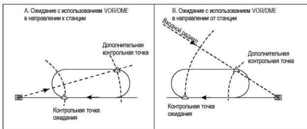
Рисунок II-4-1-3 - Вход через контрольную точку VOR/DME на линии пути удаления
