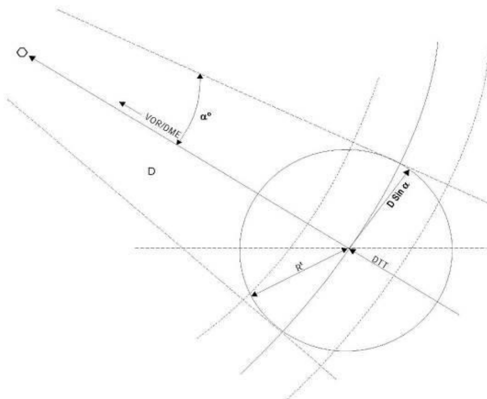
Рисунок III-3-7-2 - Построение зон допуска на точку пути
