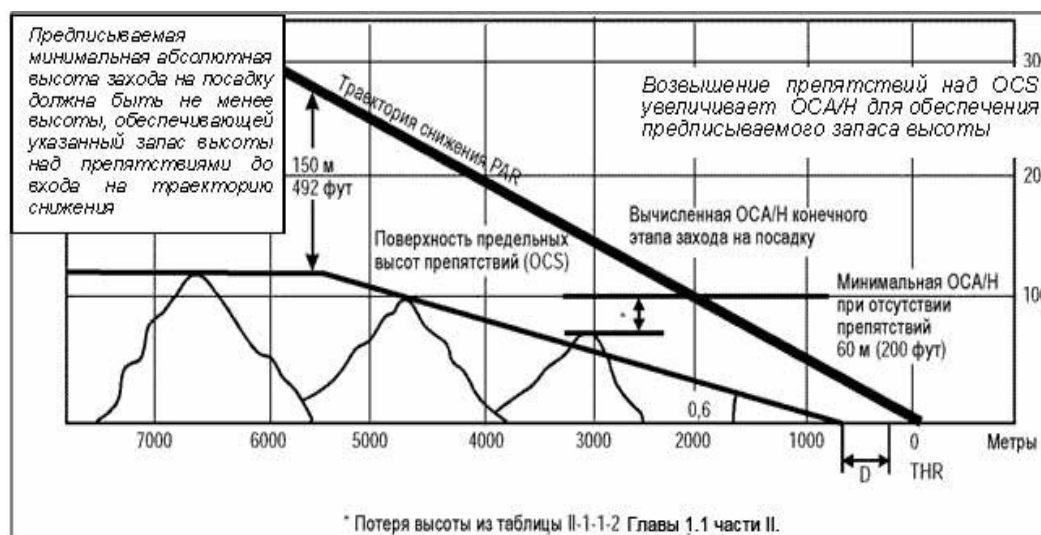
Рисунок II-1-5-1 - Определение ОСА/Н конечного этапа захода на посадку по PAR
