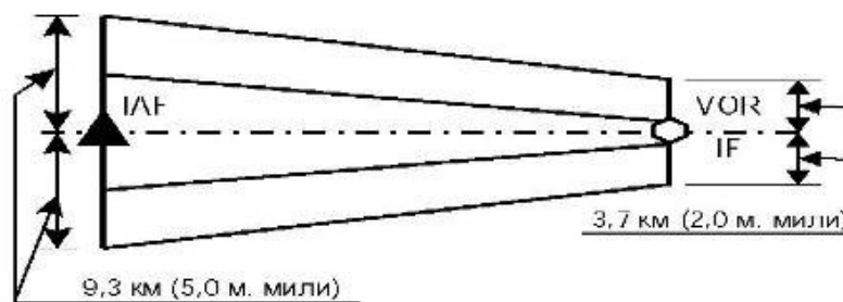
Рисунок I-4-3-Доб В-2 - Случай, когда IAF находится на расстоянии менее или равном 40,5 км (21,9 м. мили) от VOR
