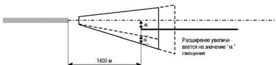
Рисунок I-4-5-9 - Вид в плане; поверхность визуального участка. Смещенный конечный участок захода на посадку параллельно осевой линии ВПП
