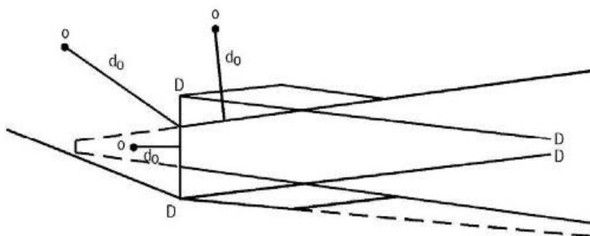
Рисунок II-1-1-Доб А-9 - Случай, когда TNH превышает 140 м (приблизительно) (разворот более чем на 75^\circ ).
